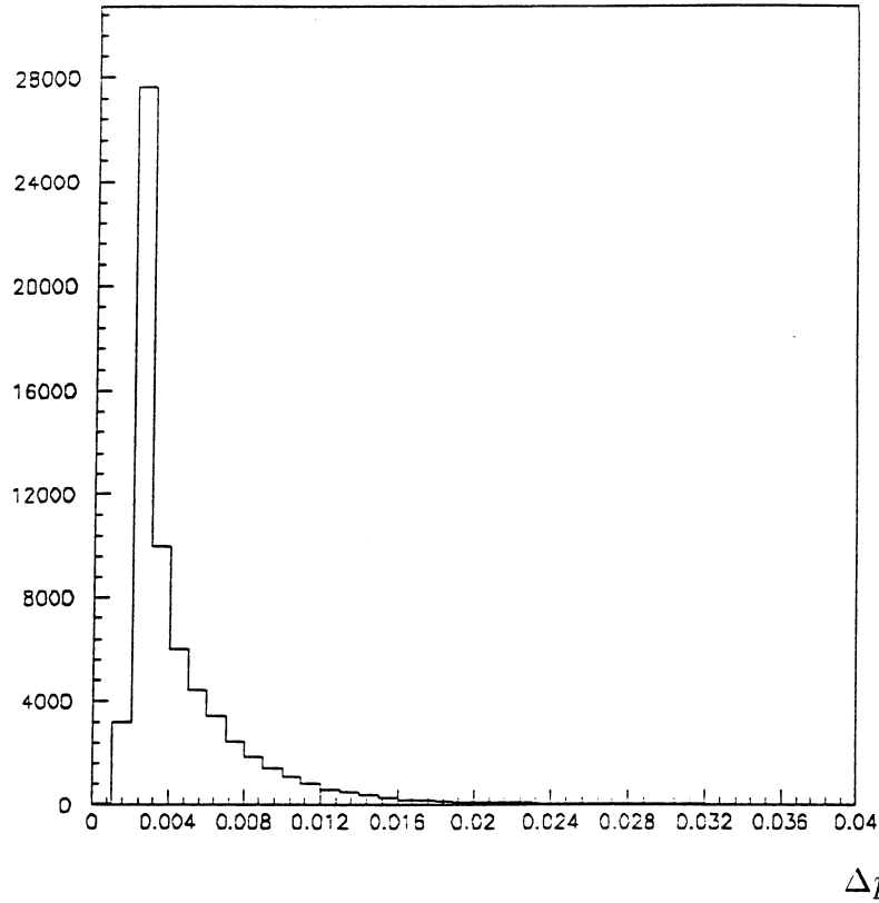
Fig. IV.13 : Distribution de la résolution en impulsion des trajectoires des particules chargées négatives reliées au vertex par le filtre de Kalman.
