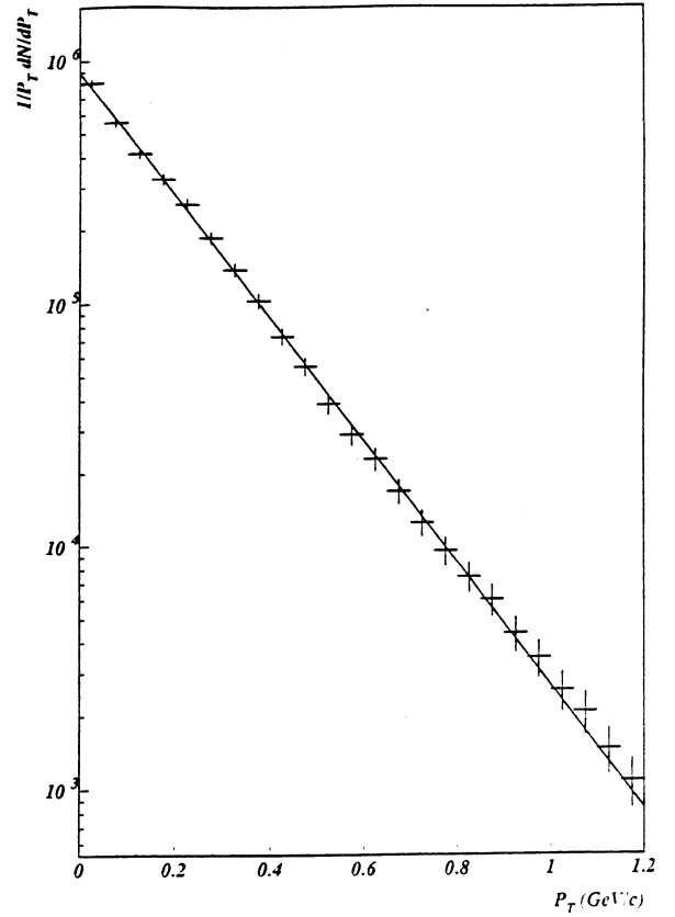
Fig. IV.21.c : Ajustement suivant une exponentielle de la distribution de l'impulsion transverse des événements de type interaction.
