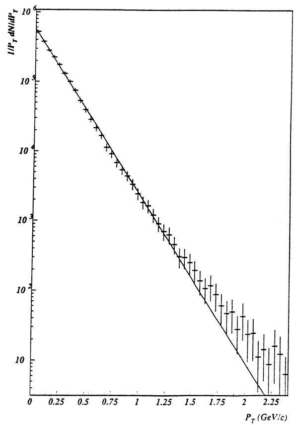
Fig. IV.16.b : Même commentaire que pour la figure IV.15. Le domaine de P_T a été limité à 2,4 GeV/c pour une comparaison avec la figure IV. 18. La droite sert à guider l'œil.
