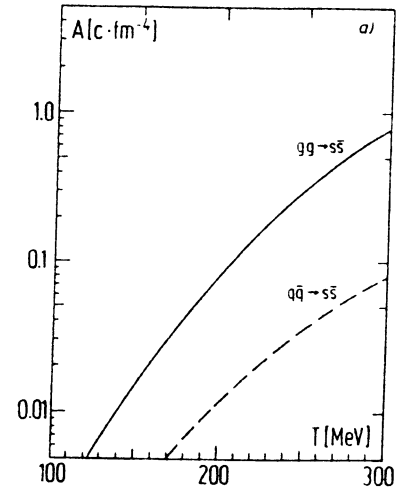
Fig.IV.2 : Taux de production de quarks s à partir des mécanismes gg \rightarrow s\bar{s} et q\bar{q} \rightarrow s\bar{s} en fonction de la température du plasma.
