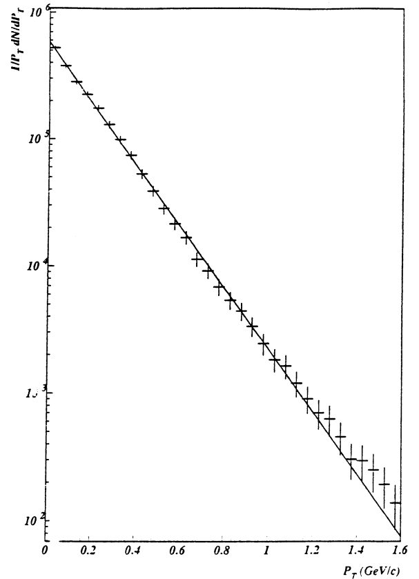
Fig. IV.17.b : Même commentaire que pour la figure IV.15. Le domaine de P_T a été limité à 1,6 GeV/c pour une comparaison avec la figure IV. 19. La droite sert à guider l'œil.
