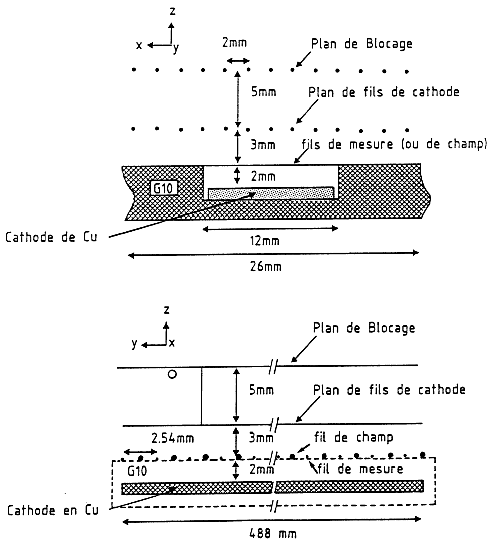
Fig. III.3 : Structure de la platine de mesure.
