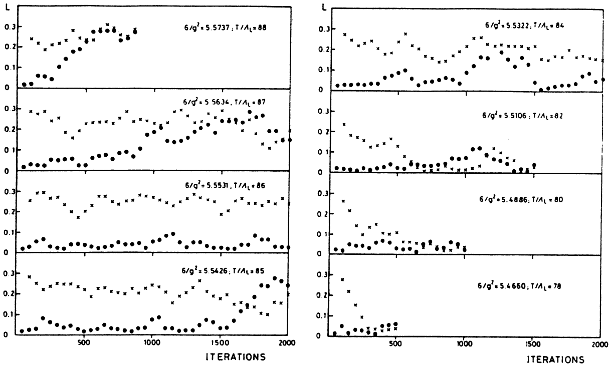
Fig. II.5 : Evolution de \langle L \rangle à partir d'un état désordonné ( \bullet ) et d'un état ordonné ( \times ) pour différentes températures.
