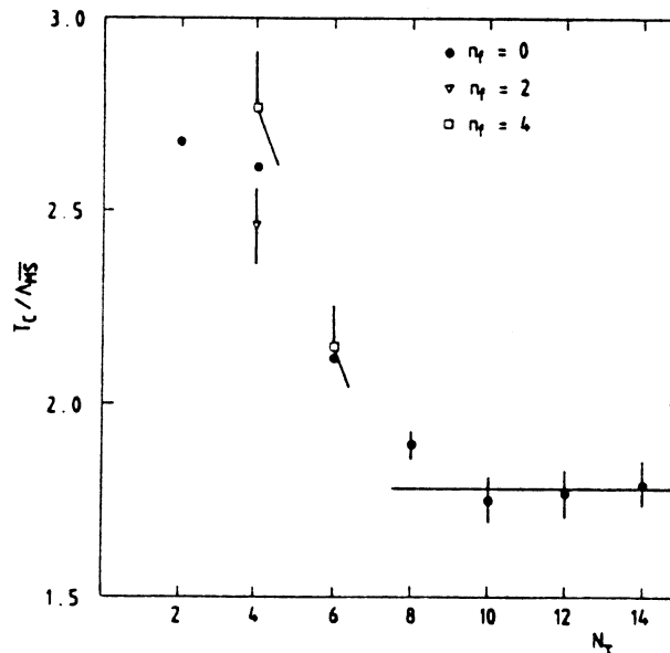
Fig. II.7 : La température critique en fonction du nombre de mailles dans la direction temporelle.
