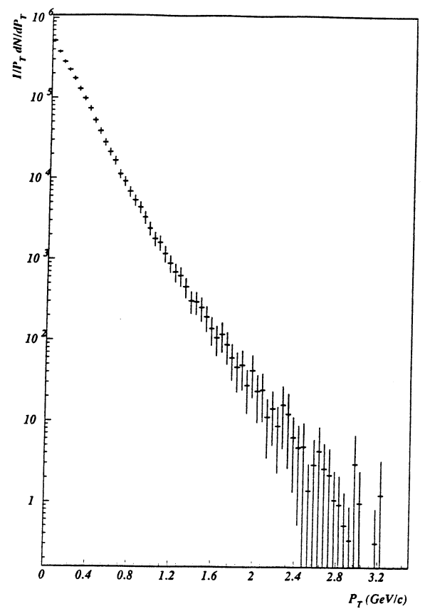
Fig. IV.15 : Distribution corrigée de l'impulsion transverse pour les événements de type central.
