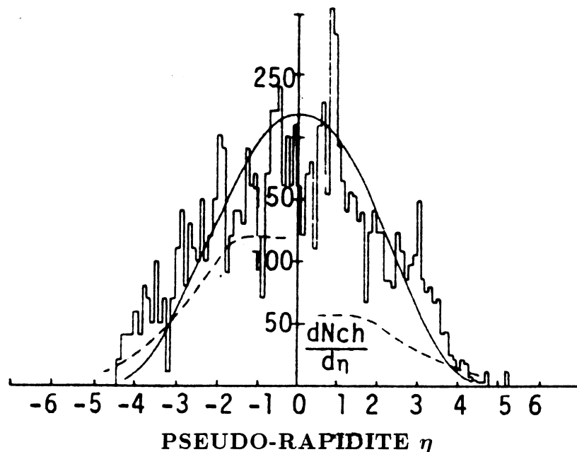
Fig.IV.15 : Distribution de pseudo-rapidité de rayons cosmiques.
