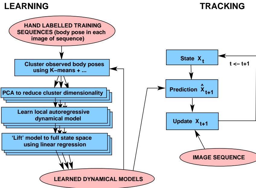
FIG. 3.3 – Une vue d'ensemble du processus d'apprentissage de notre modèle dynamique pour le suivi 2-D.
