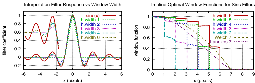
FIG. 7.2 – À gauche: les filtres d'interpolation linéaires qui minimisent l'erreur d'interpolation empirique ont une forme oscillante similaire aux filtres classiques « sinc », mais avec des queues nettement moins étendues – 2–3 oscillations suffisent en pratique – et ils ont aussi de petits discontinuités de gradient à chaque traversée de zéro. À droite: si les filtres empiriques sont exprimés en terme des filtres sinc fenêtrés équivalents, les fonctions de fenêtrage descendent en escalier, et non pas selon l'enveloppe lisse prônée par les textes classiques de traitement du signal.
