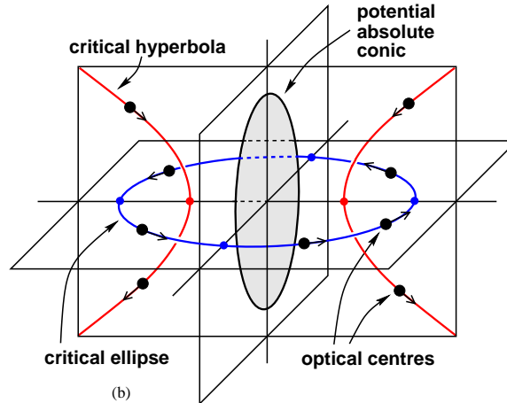
FIG. 8.1 – Un exemple d’une configuration critique. À partir de deux images, et quand les positions et les focales des deux caméras sont inconnues, si les deux caméras tombent dans une configuration relative où elles sont toutes les deux sur une courbe composée d’une hyperbole et d’une ellipse dont la géométrie relative est connue, et avec leurs axes optiques tangents à cette courbe, la configuration est critique et les positions, les focales et la géométrie euclidienne de la scène ne peuvent pas être récupérées de façon stable.
