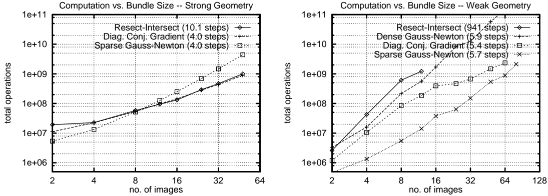
FIG. 8.2 – L'efficacité relative des algorithmes d'ajustement de faisceaux a une forte dépendance sur la géométrie du problème. À gauche: les algorithmes simplistes comme l'alternance classique résection - intersection marchent bien quand la géométrie est forte – ici, une nuage sphérique de points 3-D, contournée par un quart de cercle des caméras qui voient tous les points. À droite: quand la géométrie devient plus faible – ici une ligne de caméras qui voient chacune une zone locale d'une bande étendue de points, pour simuler un « strip » de photogrammétrie aérien – les méthodes simplistes deviennent trop inefficaces, et il faut adopter un méthode de type Newton qui exploite la structure du Hessien. Voir la référence [TMHF00] pour plus de détails.
