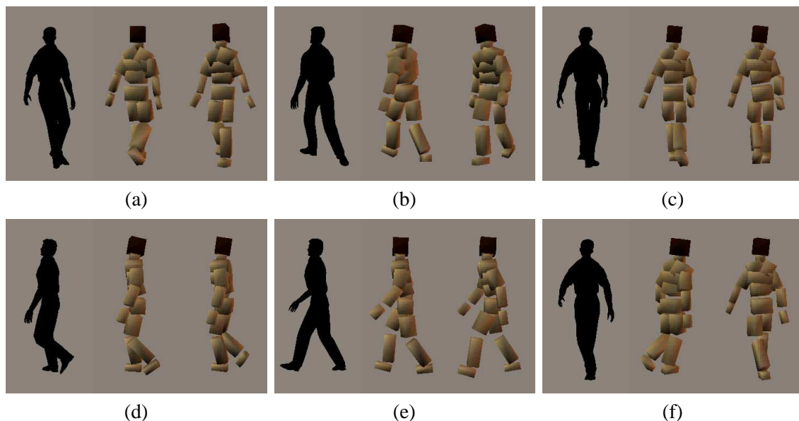
FIG. 4.6 – Quelques exemples de la reconstruction silhouette multi-hypothèse. Chaque panneau montre une silhouette d'origine et les deux reconstructions qui sont jugées les plus probables par la méthode. (a,b) montrent des ambiguïtés face-dos; (c) montre une saute cinématique (échange avant-arrière) des deux jambes; (d,e) montrent des ambiguïtés d'étiquetage entre les deux jambes; et (f) montre un cas où la première solution est erronée suite à une mis-estimation de probabilité (la bonne solution est aussi trouvée, mais elle reçoit une probabilité plus faible).
