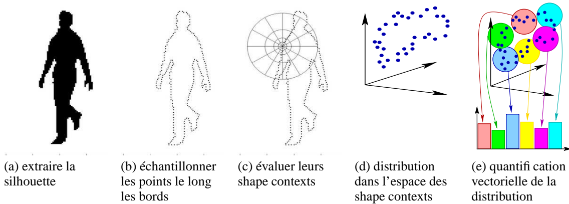
FIG. 4.1 – Le processus d'extraction de descripteur de silhouette. Les descripteurs « shape context » sont calculés à des points régulièrement espacés le long de la silhouette, et la distribution des réponses est encodée dans un histogramme 100-D par quantification vectorielle.
