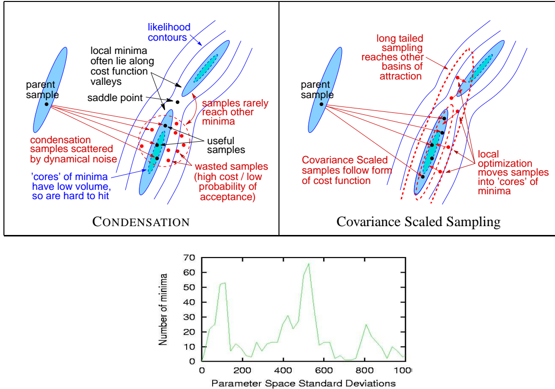
FIG. 2.2 – En haut: pourquoi l'échantillonnage CONDENSATION classique devient insuffisant pour les problèmes mal conditionnés en haute dimension. (i) Si la distribution d'échantillonnage ne suit pas la forme de la vraisemblance (fonction de coût), la plupart des échantillons sont perdus dans les régions de coût élevé aux bords du minimum local (petit rapport de volume entre une ellipsoïde et sa sphère englobante en dimension élevée). (ii) Si la distribution d'échantillonnage n'a pas de queues étendues, les échantillons arrivent trop rarement jusqu'aux voisinages des minima voisins, qui sont typiquement distant d'un grand nombre d'écart types. (iii) En dimension élevée, il est rare de tomber droit dans le noyau central d'un minimum en raison du petit volume du centre par rapport au bassin d'attraction, donc si après l'échantillonnage on n'optimise pas localement les échantillons avant de décider de les retenir ou pas, la plupart d'entre eux sont perdus en raison de leur coût élevé. En bas: histogramme typique de la séparation d'un minimum donné des minima locaux voisins, en écart types. Un échantillonnage Gaussien classique de 35 DDL n'arrivera presque jamais à pénétrer jusqu'à ces minima.
