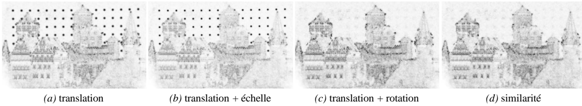
FIG. 7.3 – Un exemple des cartes de stabilité de mise en correspondance locale, sous les transformations indiquées. Par exemple, si on demande que la mise en correspondance soit stable sous les rotations image, la réponse aux points circulaires baisse nettement – comparez les images (a) et (c). Chaque carte présente la valeur propre minimale du tenseur de structure généralisé correspondant. Nos détecteurs déclarent un point clé à chaque maximum suffisamment grand en position et en échelle de la carte de stabilité correspondante.
