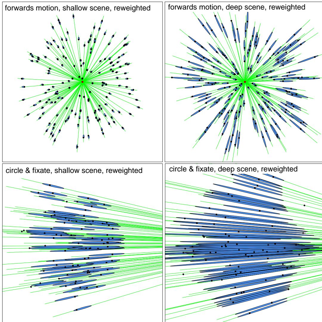
FIG. 7.6 – Quelques exemples des prédictions de la position probable du point correspondant, produites par le modèle Distribution Conjointe de Features projectif deux images (l’analogue DCF d’une matrice fondamentale). La caméra avance (première ligne) et va de gauche à droite (deuxième ligne) dans une scène presque plane (à gauche) et profonde (à droite). Dans le cas de scènes peu profondes, le modèle s’approche d’une homographie image à laquelle s’ajoutent les ellipses d’incertitude de transfert de points. Pour les scènes plus profondes, les ellipses s’étendent progressivement pour s’approcher d’une géométrie épipolaire classique (à laquelle s’ajoutent encore une fois les incertitudes). Contrairement aux modèles homographiques et épipolaires classiques, l’estimation de la DCF reste stable dans tous ces cas, sans sélection de modèle, et la recherche des points correspondants le long des droites épipolaires s’adapte naturellement à la profondeur de la scène observée.
