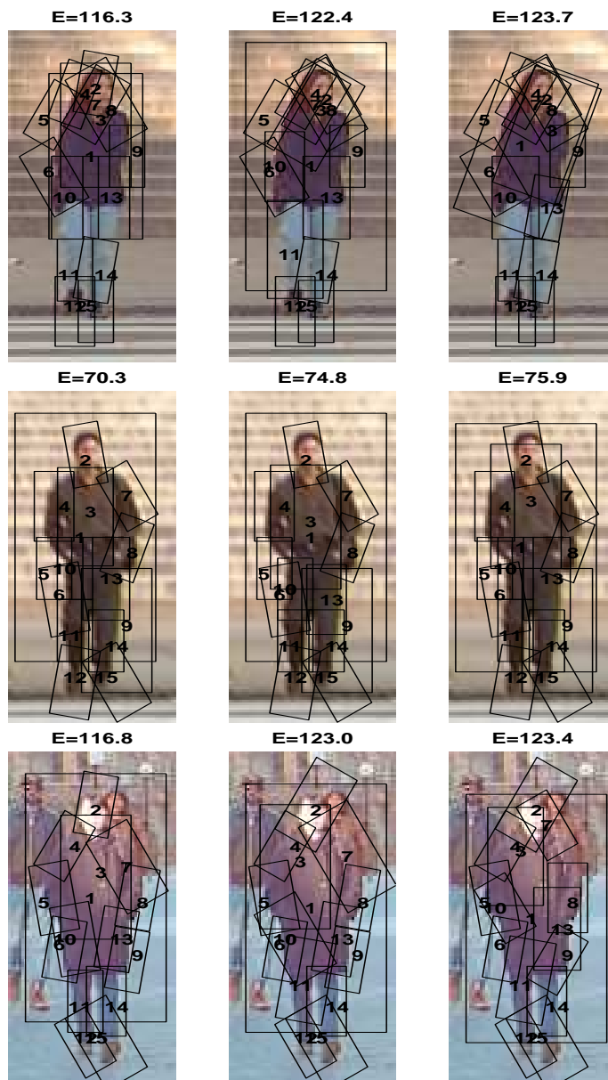
FIG. 3.2 – Detections de personne triées par ordre de probabilité décroissant, et leurs log-vraisemblances correspondantes, selon la méthode programmation dynamique sur les détecteurs machine à vecteur de support. Trois detections chacune pour trois personnes sont montrées, sur la base de piétons de MIT.
