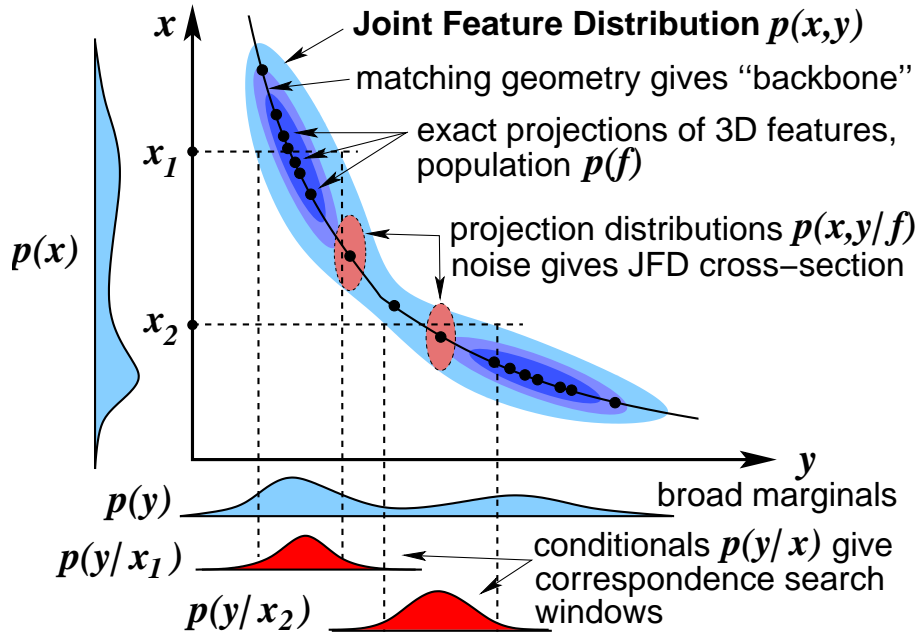
FIG. 7.5 – La mise en correspondance « Distribution Conjointe de Features (DCF) » est basée sur l'apprentissage d'un modèle de la distribution conjointe des positions image des paires, triples, etc, de primitifs correspondants entre deux, trois, etc, images. En raison des contraintes (géométriques ou autres) qui lient les primitifs correspondants entre images, la DCF est en générale assez étroite dans l'espace conjoint, quoique ses marginales (projections) dans les images individuelles soient floues. (Dans le cas des contraintes géométriques rigides, l'épaisseur de la DCF est donnée par le bruit d'extraction de primitif). À partir du modèle, conditionner sur la position d'un primitif image donné prédit la distribution des positions de son/ses correspondant(s) dans la/les autre(s) image(s). Cette information peut être utilisée pour guider la recherche des primitifs correspondants.
