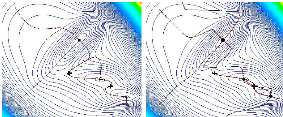
FIG. 2.4 – Les trajectoires de suivi de vecteur propre (à gauche), et de balayage d'hyper-surface (à droite), dans un problème synthétique 2-D simple. Les points marquent les trois minima de la fonction de coût, et les croix marquent les deux points de selle. Les trajectoires qui sont lancées à partir de chaque minimum trouvent les autres minima.
