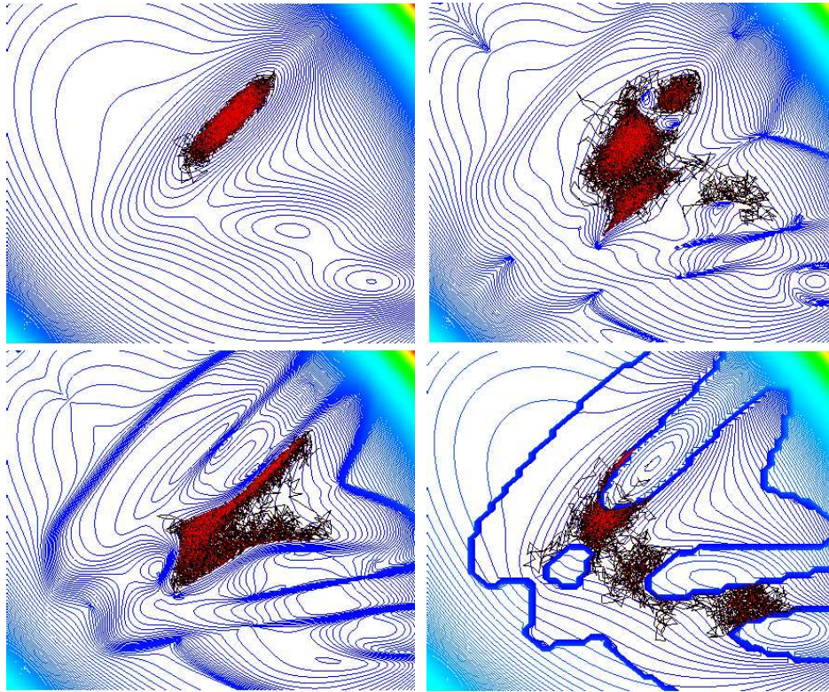
FIG. 2.6 – L'effet des deux paramètres qui déterminent la forme de la fonction de coût hyperdynamique. Première ligne: à gauche, sans modification hyperdynamique, l'échantillonnage chaîne de Markov est coincé – il n'arrive pas à sortir du minimum initial. À droite, une petite contribution hyperdynamique commence à faire sortir la recherche du minimum. Deuxième ligne: une contribution hyperdynamique plus forte focalise l'échantillonnage sur les zones des deux points de selle. À gauche: avec une échelle de transition spatiale grande, l'échantillonnage se focalise sur le premier point de selle. À droite: une échelle spatiale plus petite rend la fonction de coût plus raide et plus convulsée, et disperse les échantillons sur les deux points de selle.
