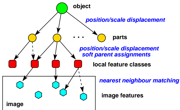
FIG. 9.1 – La structure de notre modèle de reconnaissance d’objets par parties. Le modèle est hiérarchique avec l’objet à la racine, les parties en fils, éventuellement les sous-parties, et au fond un ensemble de classes type – classées selon l’apparence et la position spatiale – de features image. Entre chaque sous-partie et son parent, il y a une transformation incertaine en position et en échelle qui caractérise le déplacement relative de la sous-partie, et la souplesse / le rigidité de ses liens avec son parent. Les attributions des parents des sous-parties sont aussi incertaines (appries pendant la phase d’apprentissage). Au fond de l’arbre, chaque classe de features est mis en correspondance avec le feature image observé le plus proche.
