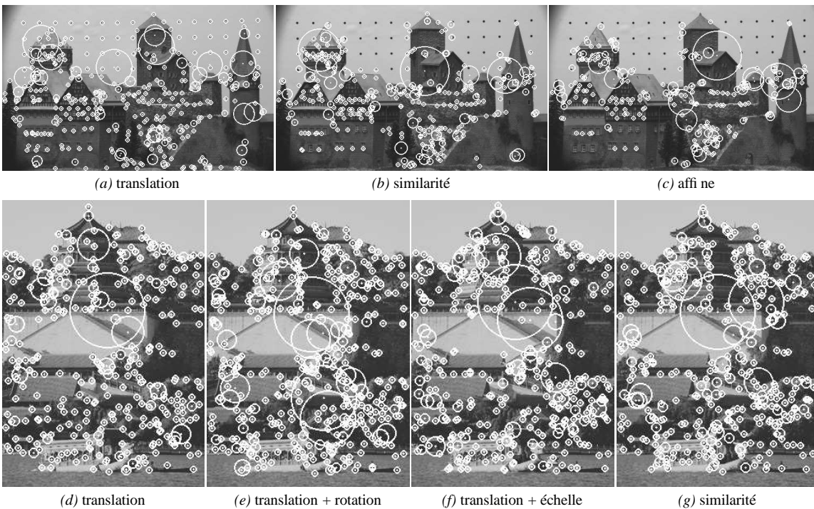
FIG. 7.4 – Quelques exemples de points clé trouvés par nos détecteurs, sélectionnés pour être stables sous les transformations infinitésimales indiquées.
