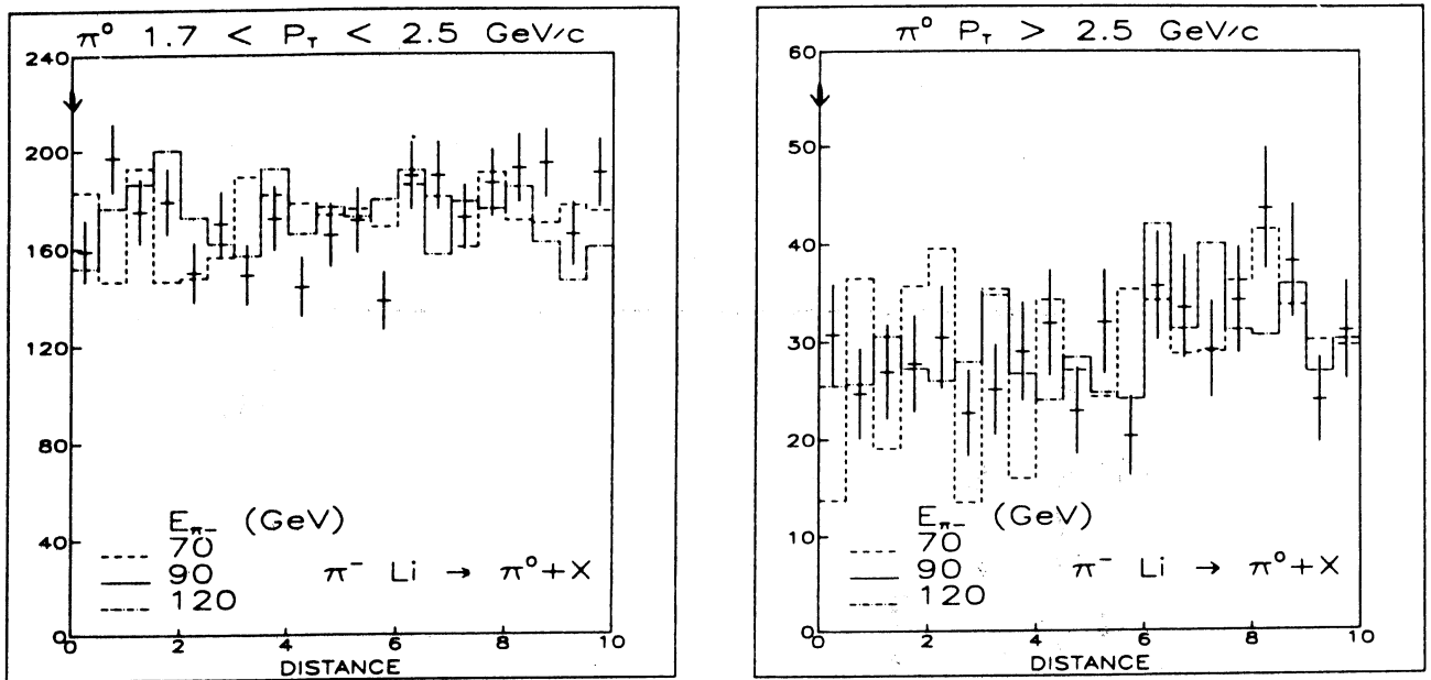
Fig. VI-7: Flux d'énergie dans le plan transverse (pions \pi^- incidents)
