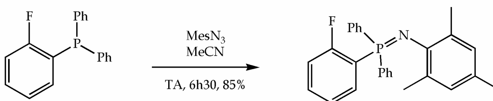
Figure 2.9 Synthèse et utilisation de \text{MesN}_3 dans la littérature.
