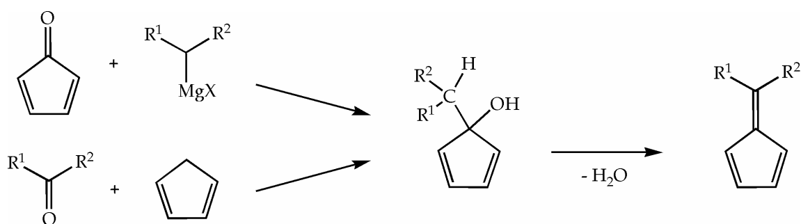
Figure 2.14 Synthèse d'un fulvène par déshydratation d'un alcool formé par 2 voies.
