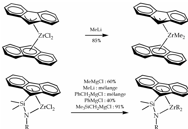
Figure 3.7 Exemples d'alkylation de complexes métallocène (25) et de CGC (21) .
