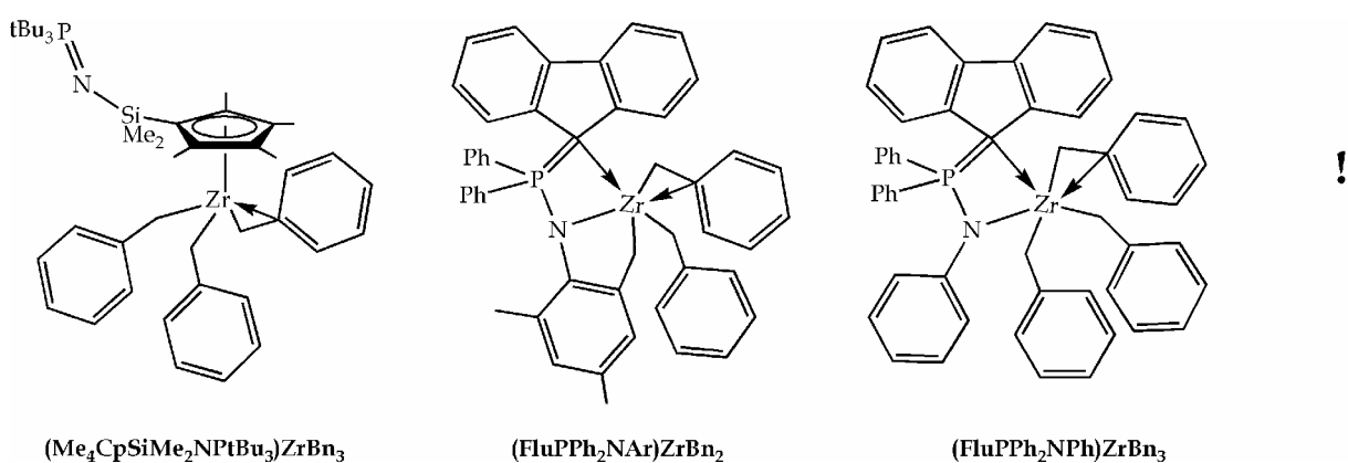
Figure C.5 Complexes synthétisés.
