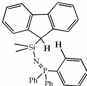
Figure 3.21 Protons acides du ligand HFluSiMe 2 NPPh 3 .
