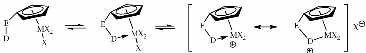
Figure I.13 Autoactivation d'un complexe de type CGC pour la polymérisation des oléfines. D = groupement donneur (base de Lewis), M = métal du groupe 4 (acide de Lewis).
