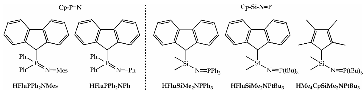
Figure 3.17 Ligands synthésisés.
