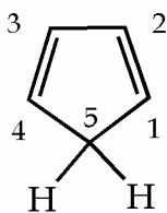
cyclopentadiène
