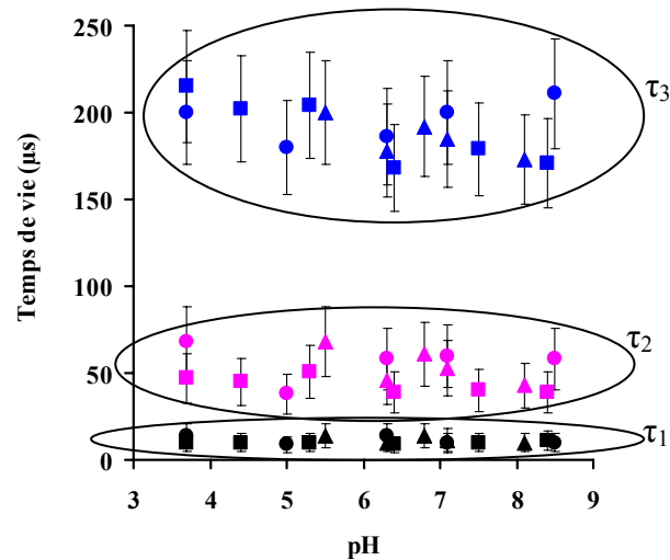
Figure 44 : Distribution des trois temps de vie \tau_1 , \tau_2 et \tau_3 nécessaires à l'ajustement des déclins temporels de fluorescence des fractions « quartz » issues des expériences de sorption réalisées à des concentrations aqueuses uranyle initiales ( [U_i] ) de 100 \mu\text{M} (triangles), 50 \mu\text{M} (ronds) et 10 \mu\text{M} (carrés), en fonction du pH. (Conditions expérimentales : solution électrolyte : [\text{NaNO}_3] = 0,1 \text{ M} ; T = 298 \text{ K} ; R = 25 \text{ g/l} ; atmosphère contrôlée en \text{N}_2 (g)).
