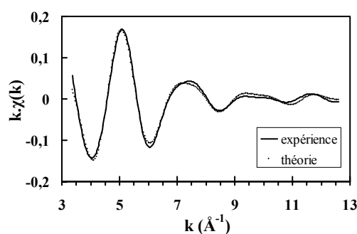
Figure 45 : Spectre EXAFS expérimental de l'échantillon de référence Q_{1000} comparé au spectre théorique.
