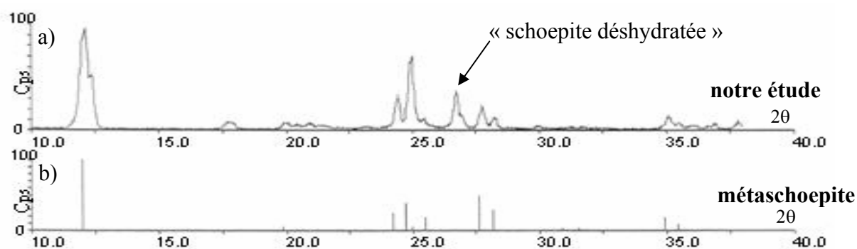
Figure 22 : (a) Diffractogramme du produit de référence de type « schoepitique » synthétisé, identifié comme un mélange de métaschoepite et de « schoepite déshydratée ». (b) Raies de diffraction de la métaschoepite synthétique indexée JCPDS 18-1436. La raie à 26,6^\circ en (a) indique la présence de « schoepite déshydratée » [95].
