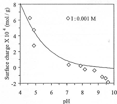
Figure 3 : Variation de la charge de surface d'un gel d'aluminium mis au contact d'une solution électrolyte \text{NaClO}_4 de concentration (I), en fonction du pH (la charge de surface est mesurée par titrages potentiométriques) et comparaison avec la courbe modélisée obtenue en appliquant les données mentionnées dans [11].
