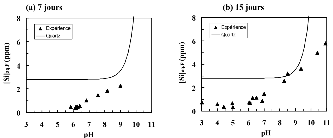
Figure 12 : Courbe de solubilité du quartz (trait) et concentrations expérimentales finales de Si dissous ( [\text{Si}]_{\text{aq,F}} ) (triangle) dans les solutions issues des expériences de sorption de U(VI) sur le
