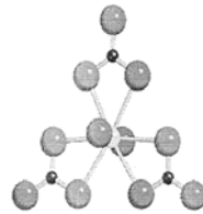
Figure 6 : Représentation de la structure géométrique du complexe tri-carbonato uranyle UO_2(CO_3)_3^{4-} [71]. La charge globale -4 du complexe n'est pas indiquée sur la figure.
