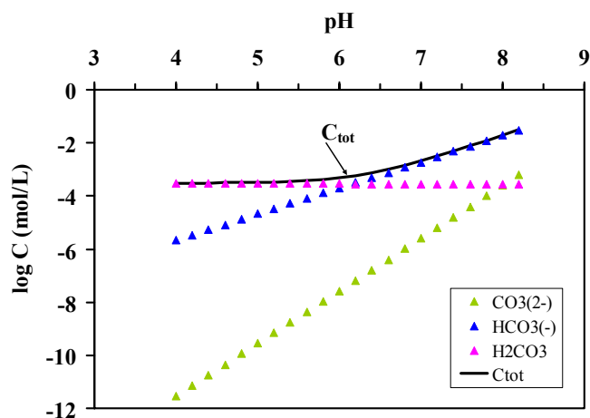
Figure 7 : Distribution des espèces carbonatées en équilibre avec une atmosphère de CO_2(g) ( pCO_2 = 10^{-2} atm) en fonction du pH. Le tracé épais représente la concentration totale en carbonates dissous ( C_{tot} ) ; (Solution électrolyte : 0,1 M NaNO_3 ).
