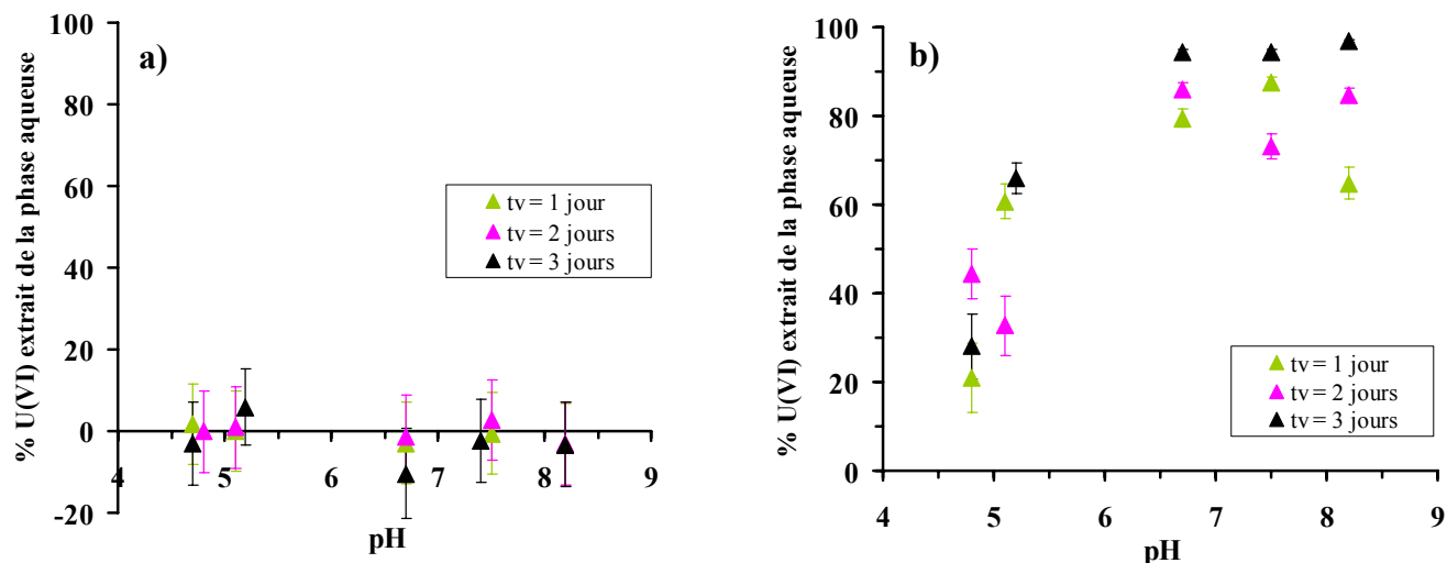
Figure 17 : Pourcentage de U(VI) extrait de la phase aqueuse (a) par formation de précipités uranyle et (b) par formation additionnelle de colloïdes uranyle, pour des solutions de concentration initiale en U(VI) dissous de 10 \mu\text{M} , à différents pH et temps de vieillissement ( t_v ). (Conditions expérimentales : solution électrolyte : [\text{NaNO}_3] = 0,1 \text{ M} ; T = 298 \text{ K} ; atmosphère contrôlée en \text{N}_2 (g)).
