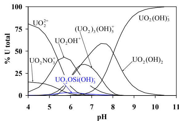
Figure 14 : Distribution calculée des espèces aqueuses uranyle en fonction du pH, dans des solutions électrolytes 0,1 M \text{NaNO}_3 , maintenues à 298 K et à l'abri du \text{CO}_2 atmosphérique, pour des concentrations totales en Si des solutions simulées et reportées sur la Figure 13 b (solutions au
