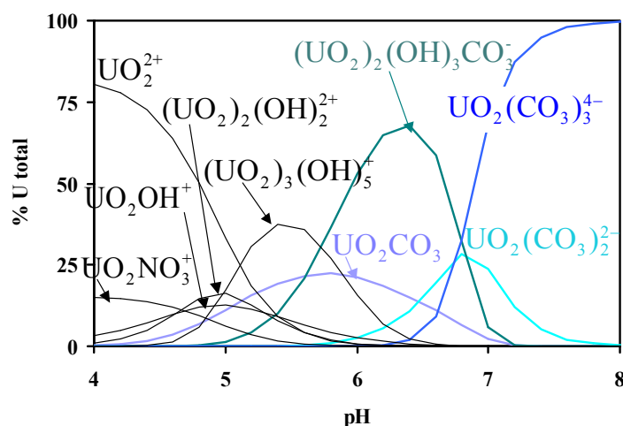
Figure 9 : Distribution calculée des espèces aqueuses de l'ion uranyle en fonction du pH, dans des solutions électrolytes 0,1 M NaNO 3 , maintenues à 298 K et à l'équilibre avec une atmosphère de N 2 (g) additionnée de 0,9 % en volume de CO 2 (g). La concentration totale en U(VI) est de 50 μM. Les données thermodynamiques utilisées sont reportées dans le Tableau 4 et le Tableau 5. La précipitation de minéraux uranyle n'est pas prise en compte. Les espèces dont la proportion est inférieure à 5 % de l'uranium total ne sont pas représentées.
