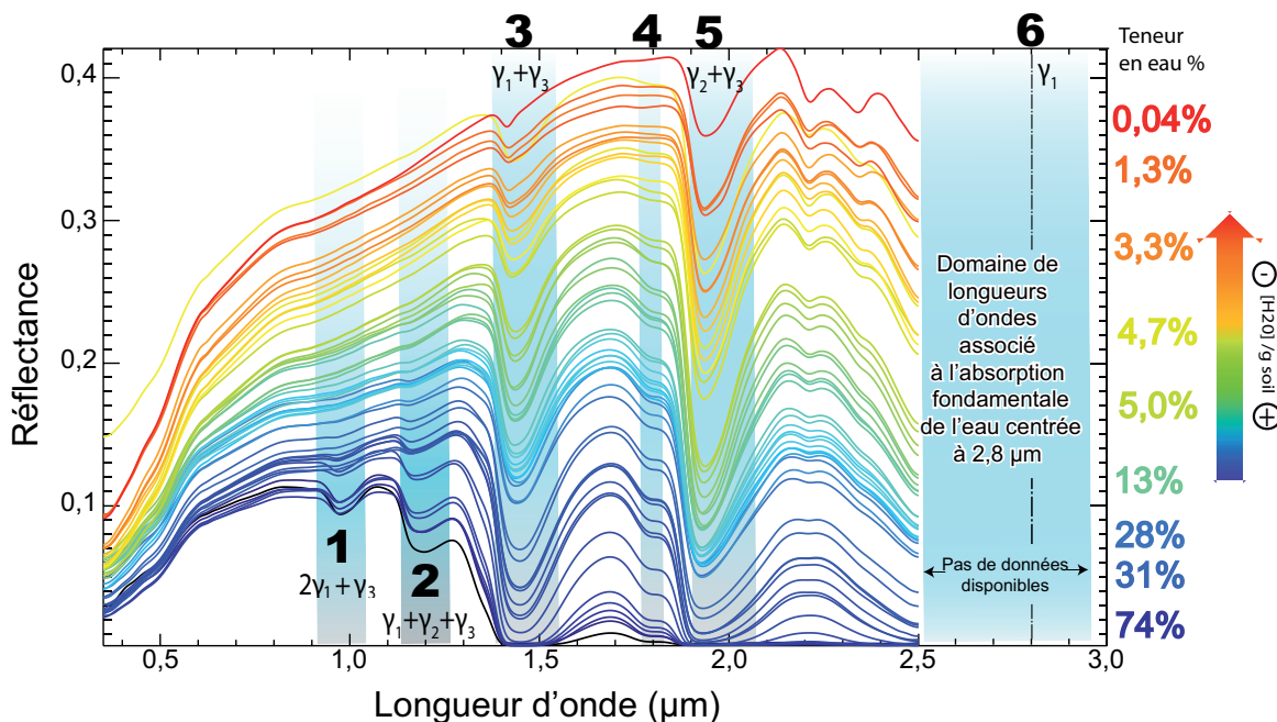
FIG. VI.1.1 – Évolution spectrale d'un sédiment sableux au cours de sa déshydratation. Les barres grisées localisent approximativement les absorptions spécifiques de l'eau depuis les courtes longueurs d'ondes aux grandes longueurs d'ondes. Successivement disparaissent les bandes centrées à 1 – 0,97 \mu\text{m} ; 2 – 1,2 \mu\text{m} ; 3 – 1,4 \mu\text{m} ; 4 – 1,79 \mu\text{m} ; 5 – 1,9 \mu\text{m} . Le chiffre 6 correspond à l'absorption fondamentale de l'eau centrée à 2,8 \mu\text{m} . Notons que le domaine de longueurs d'ondes de l'instrument l'ASD FieldSpec3 FR ne permet pas de couvrir la gamme spectrale spécifique à l'absorption fondamentale.
