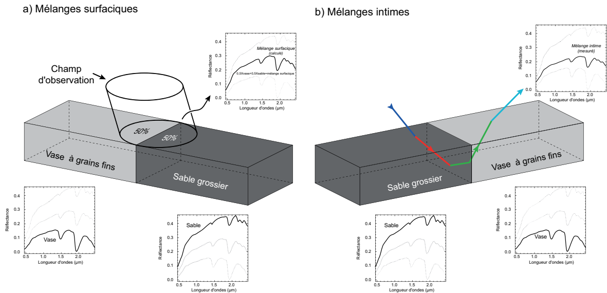
FIG. III.5.3 – a) Mélanges surfaciques. Le spectre résultant du mélange correspond à une combinaison linéaire des spectres des surfaces qui composent le champs d'observation du capteur, soit 50 % de vase et 50 % de sable. b) Mélanges intimes. Le spectre résultant est mesuré en laboratoire. Le rayonnement incident (trait en bleu) interagit avec le matériau. Il est réfracté au niveau des interfaces des grains voisins dont la composition et les tailles peuvent être différentes (traits en rouge et vert). Le trait en cyan correspond au rayonnement mesuré ; il résulte de la convolution sur le chemin optique de chacune des particules rencontrées et le milieu interstitiel (eau, air) (Modifié d'après Roy 2007).
