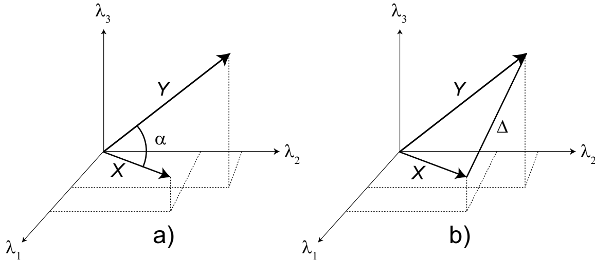
FIG. III.5.2 – Principe de classification représentant deux métriques couramment utilisées en télédétection hyperspectrale. a) le Spectral Angle Mapper, \alpha ; b) la distance Euclidienne minimum (DEM), \Delta .
