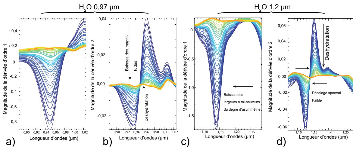
FIG. VI.1.6 – Évolution spectrale des bandes d'absorption spécifiques de l'eau d'un sédiment sablo-vaseux au cours de la déshydratation (échantillon n°2 c.f. § Annexe A). Les figures a et b montrent respectivement les dérivées premières et secondes de l'absorption centrée à 0,97 \mu\text{m} . Les figures c et d montrent respectivement les dérivées premières et secondes de l'absorption centrée à 1,2 \mu\text{m} .
