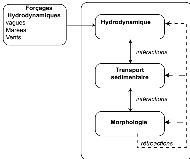
FIG. I.2.12 – Composantes d’un système morphodynamique côtier
