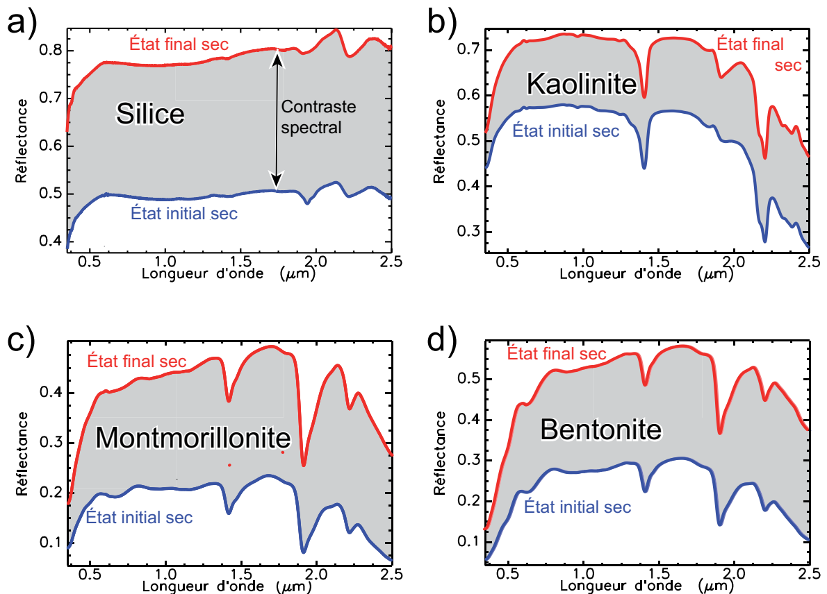
FIG. VI.1.9 – Spectres de réflectance illustrant le contraste spectral associé au phénomène de réarrangement des particules au sein des matériaux à la suite de leur déshydratation. Les spectres sont représentés à l'état initial (avant déshydratation) et à l'état final (après déshydratation). Les formes spectrales ne changent pas, seuls leurs niveaux de réflectivité varient. Le fort niveau de réflectivité des spectres à l'état final est dû à une diminution de la rugosité et à une baisse de la porosité au cours de la déshydratation. a) poudre de silice hyperfine, b) argile de type kaolinite, c) argile de type montmorillonite, d) argile de type bentonite.
