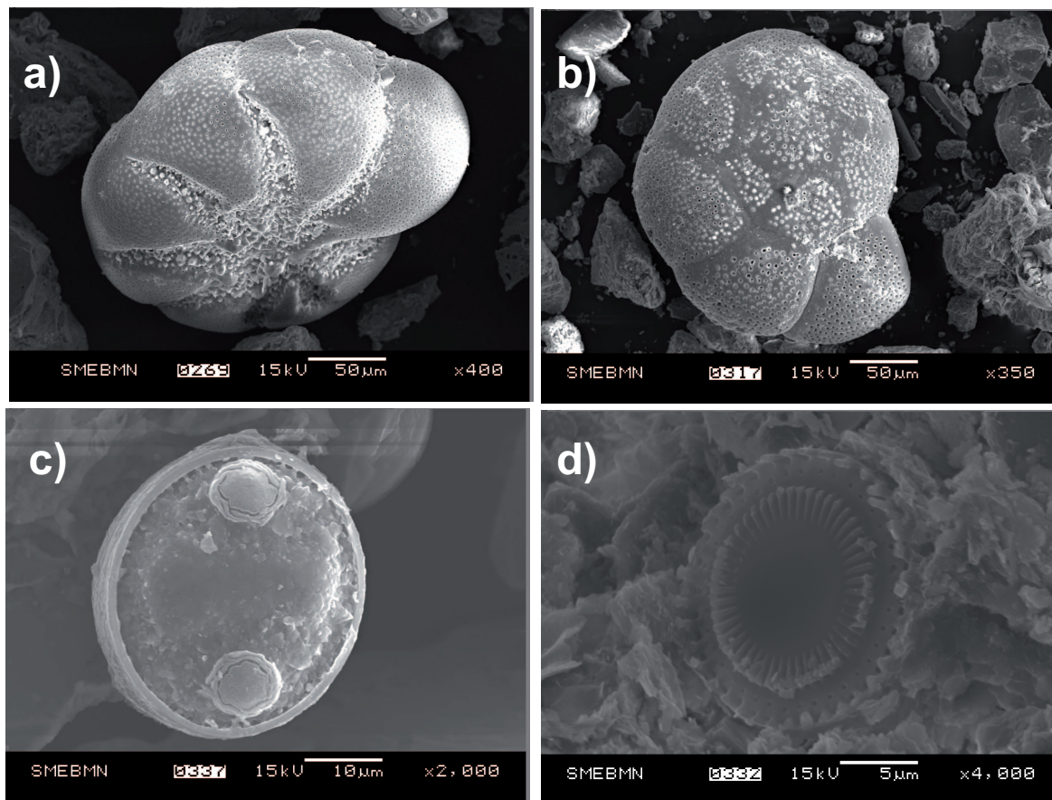
FIG. IV.2.5 – Images acquises au microscope électronique à balayage (M.E.B.) illustrant les micro-organismes carbonatés. a) et b) sont des exemples de foraminifères dont les tests sont perforés ; c) microfossile d'origine systématique inconnue ; d) plaque de coccolithe.
