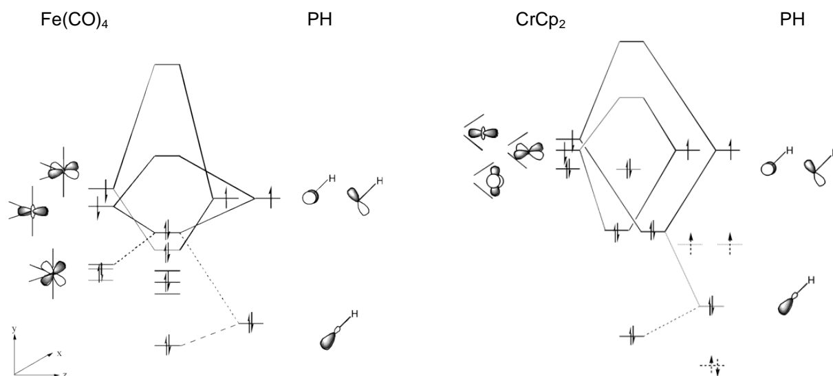
Schéma 13 : Diagrammes des orbitales moléculaires de \text{Fe}(\text{CO})_4(=\text{PH}) (à gauche) et \text{CrCp}_2(=\text{PH}) (à droite). Les pointillés indiquent les énergies des orbitales de \text{PH} lorsqu'il est à distance infinie de \text{CrCp}_2 .
