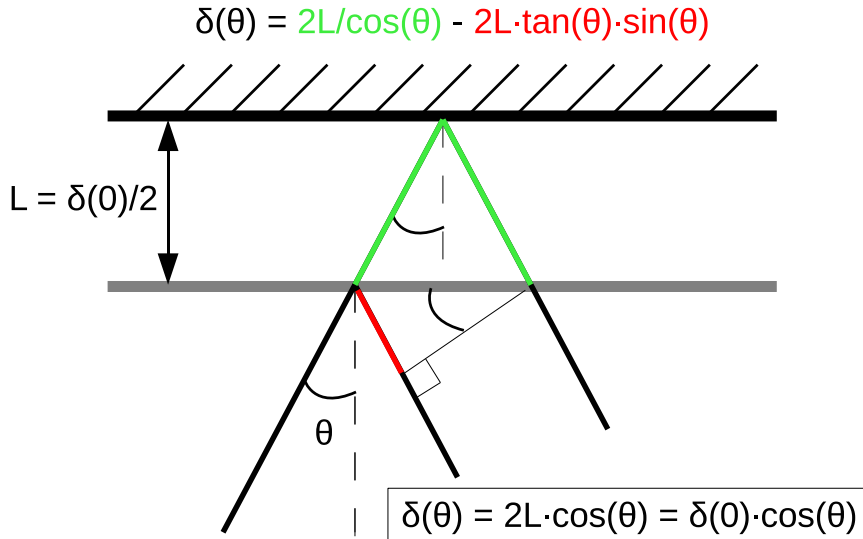
FIG. 1.22 – Influence de champ du spectromètre sur la différence de marche. Celle-ci dépend, pour une position donnée des miroirs de l'incidence des rayons.
