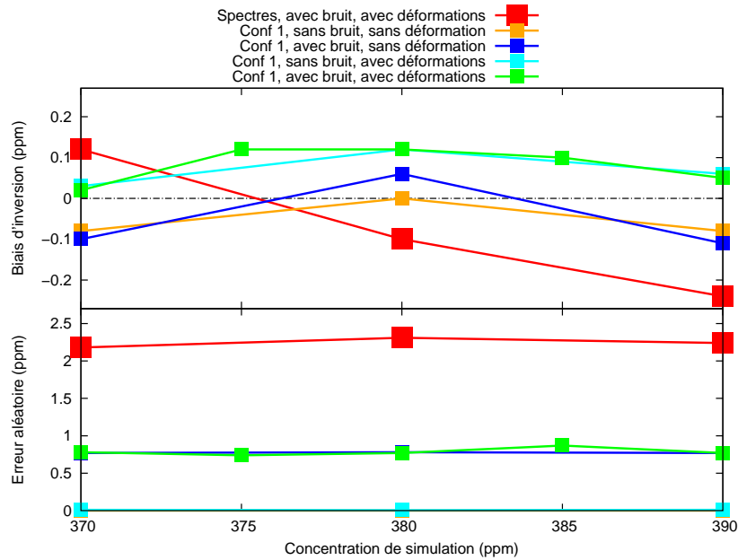
FIG. 4.28 – Différents cas d'inversion des interférogrammes avec la première configuration instrumentale, où les échelles d'étalonnage sont situées au voisinage de la différence de marche nulle. On reprend, pour comparaison, les résultats d'inversion des spectres avec bruit et déformations de la figure 4.26. L'erreur aléatoire obtenue en inversant les interférogrammes sans bruit et sans déformation (en jaune) est située autour de 0.
