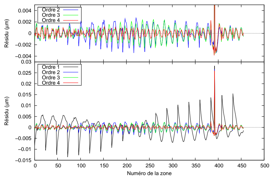
FIG. 2.17 – Résidu de déformation des différences de marche après corrections des mouvements d'ensemble d'ordres différents. On voit que la prise en compte d'un polynôme d'ordre 2 permet de réduire considérablement le résidu. Le graphe du haut représente uniquement les corrections d'ordres 2, 3 et 4 avec une échelle mieux adaptée.
