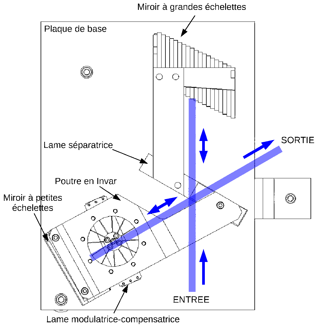
FIG. 2.12 – Vue de dessus du cœur interférométrique
