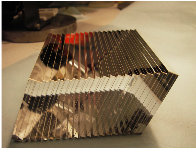
FIG. 2.10 – Miroir à grandes échellettes du nouveau cœur interférométrique. On notera que pour des raisons de facilité d'assemblage, les lames constituant les marches ont toutes la même taille (elles sont juste décalées les unes par rapport aux autres), contrairement au miroir précédent (voir la figure 1.25).
