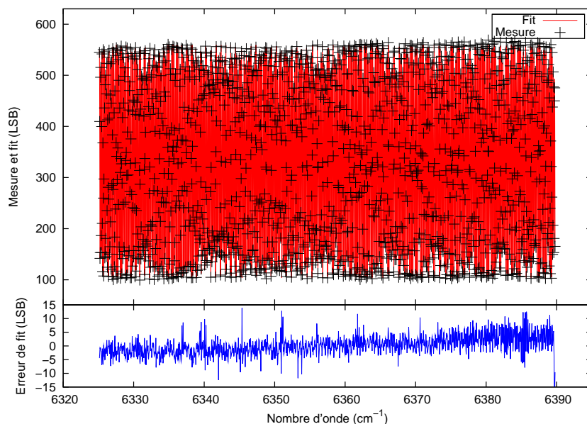
FIG. 3.7 – Optimisation de la fonction d’ajustement lors du traitement d’une mesure laser pour l’étalonnage des différences de marche. Les paramètres d’une fonction de modélisation ont été optimisés pour minimiser les différences avec la mesure. En particulier, la différence de marche a été ajustée. Cette figure représente le signal mesuré pour une échelle (donc une différence de marche) en fonction du nombre d’onde. La fréquence dépend de la différence de marche. Sur le graphe, on distingue également le maximum et le minimum de modulation du signal interférométrique qui varie avec la différence de marche. Ce type d’ajustement sera reproduit pour toutes les échelles.
