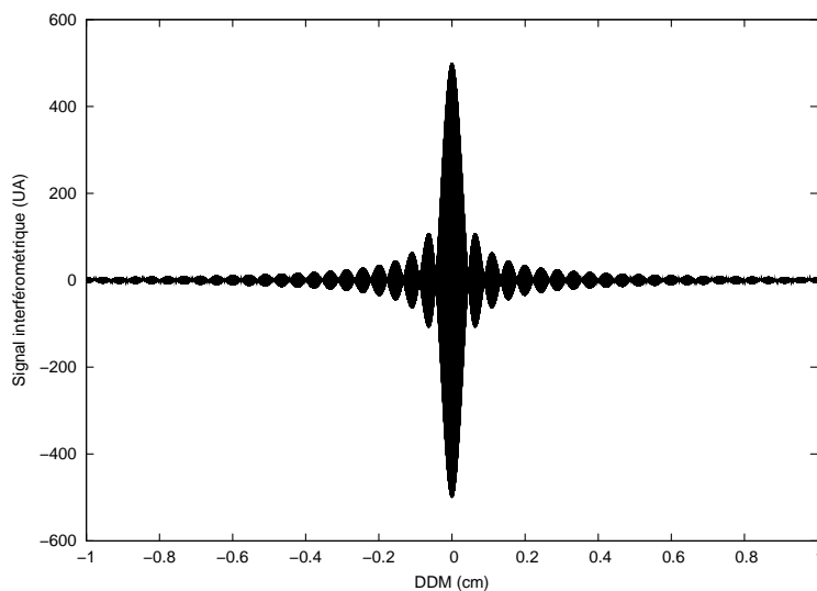
FIG. 1.12 – Simulation d'un interférogamme de source « large » spectralement entre -1 et 1 cm de différence de marche. La période d'échantillonnage de la courbe est égale à environ un quart de la longueur d'onde centrale. On distingue bien sur ce graphe l'enveloppe de l'interférogamme qui est représentative du spectre observé, et dont la porteuse a pour période la longueur d'onde centrale.
