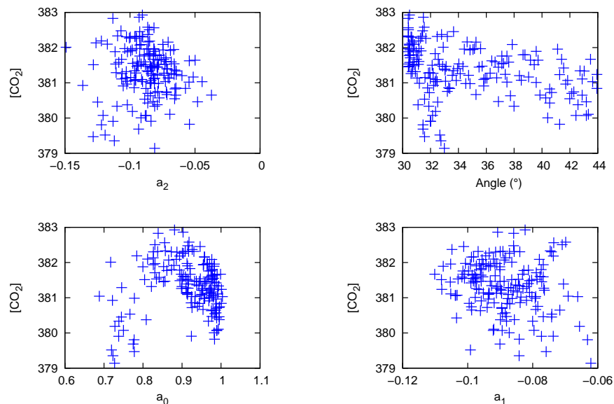
FIG. 5.9 – Concentration en dioxyde de carbone retrouvée en fonction des coefficients de réflectance et de l'angle solaire zénithal.
