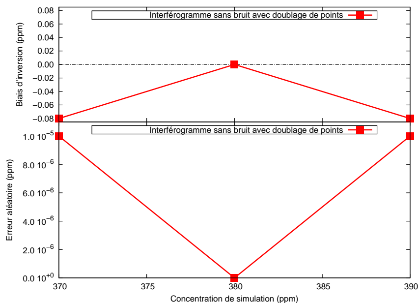
FIG. 4.18 – Inversions de l'interférogramme sans bruit. Le graphique supérieur représente le biais d'inversion en fonction de la concentration de simulation tandis que le graphique inférieur représente l'erreur aléatoire d'inversion.
