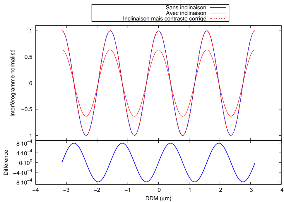
FIG. 3.14 – Étude de l'effet de l'inclinaison des échelettes sur le contraste interférométrique. Le graphe du haut représente les interférogrammes normalisés. L'interférogramme bleu est calculé sans inclinaison, son contraste est égal à 1. L'interférogramme en rouge, ligne pleine, est calculé pour une inclinaison des miroirs faisant varier la phase de \pi . Le contraste est égal à 0,6. La courbe en pointillés rouges représente l'interférogramme après correction du contraste. Le graphe du bas montre la différence entre l'interférogramme corrigé et l'interférogramme théorique idéal.
