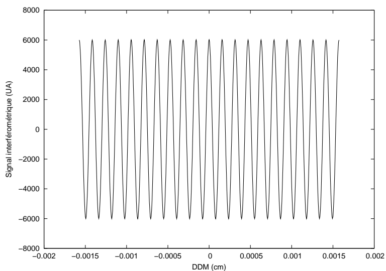
FIG. 1.13 – Simulation d'un interférogamme de source « large » spectralement entre -10 et 10 longueurs d'onde en différence de marche. La période d'échantillonnage de la courbe est environ 30 fois plus petite que la longueur d'onde centrale. On voit la variation sinusoïdale de période égale à la longueur d'onde centrale, porteuse de l'enveloppe de l'interférogamme. On remarquera que la diminution de contraste due à l'enveloppe est trop faible pour être visible sur l'intervalle étroit de différence de marche considéré.
