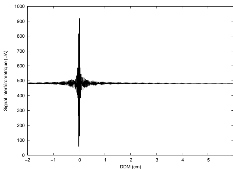
FIG. 1.11 – Simulation d'un interférogramme de source « large » spectralement entre -2 et 6 cm de différence de marche. On distingue une partie constante aux alentours de 500 : la ligne de base. Les variations autour de la ligne de base constituent le signal interférométrique. C'est le signal utile pour la mesure des spectres. La période d'échantillonnage de la courbe est environ 10 fois plus grande que la longueur d'onde centrale.
