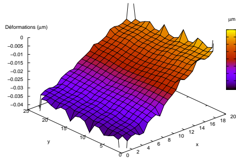
FIG. 2.18 – Déformations spatiales de l'interféromètre mesurées entre 2 mesures espacées de 8 jours. Les valeurs sont en différence de marche optique.
