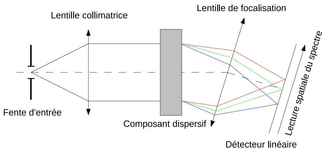
FIG. 1.5 – Schéma de principe d'un spectrographe à prisme ou à réseau. Les couleurs différentes des faisceaux en sortie de l'élément dispersif représentent les longueurs d'onde des rayons.
