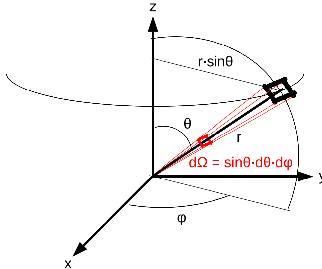
FIG. 1.1 – Représentation d'un angle solide. L'élément différentiel d'angle solide est donné pour des coordonnées sphériques.
