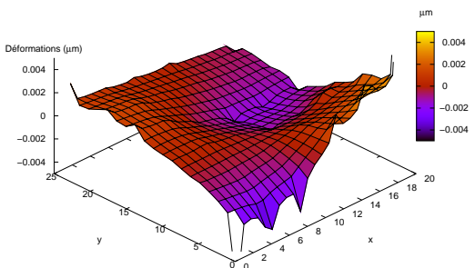
FIG. 2.19 – Résidu de déformations spatiales de l'interféromètre après correction de l'ordre 1, pour une période de 8 jours. Les valeurs sont en différence de marche optique.
