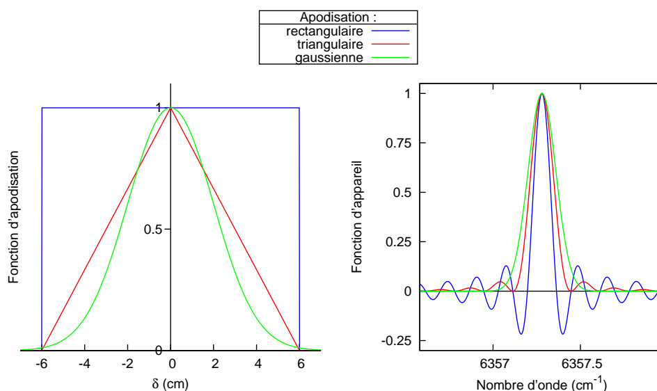
FIG. 1.16 – Fonctions d'appareil pour différentes fonctions d'apodisation. A gauche, on présente les fonctions d'apodisation, à droite les fonctions d'appareil correspondantes. Pour les courbes en bleu l'apodisation est rectangulaire, c'est l'apodisation naturelle due à la limitation de la différence de marche. Pour les courbes en rouge, l'apodisation est triangulaire et, pour les courbes vertes, elle est gaussienne.
