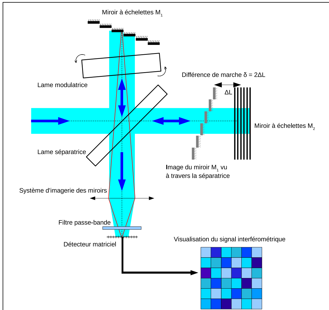
FIG. 1.24 – Interféromètre de Michelson statique, schéma de principe
