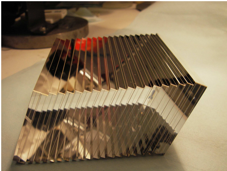
FIG. 2.10 – Miroir à grandes échelettes du nouveau cœur interférométrique. On notera que pour des raisons de facilité d'assemblage, les lames constituant les marches ont toutes la même taille (elles sont juste décalées les unes par rapport aux autres), contrairement au miroir précédent (voir la figure 1.25).
