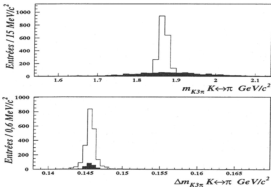
Figure VII.7: spectre en masse pour les événements où les masses du pion et du kaon de même charge ont été inversées dans la simulation (en noir). L'histogramme présente le spectre du vrai signal.
