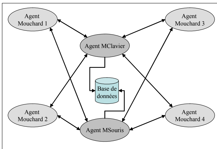
Figure III.9. Architecture du moucharde électronique. Le nom des agents moucharde est celui des agents d'interface précédé d'un « M » [Trabelsi et al. , 2004 b].
