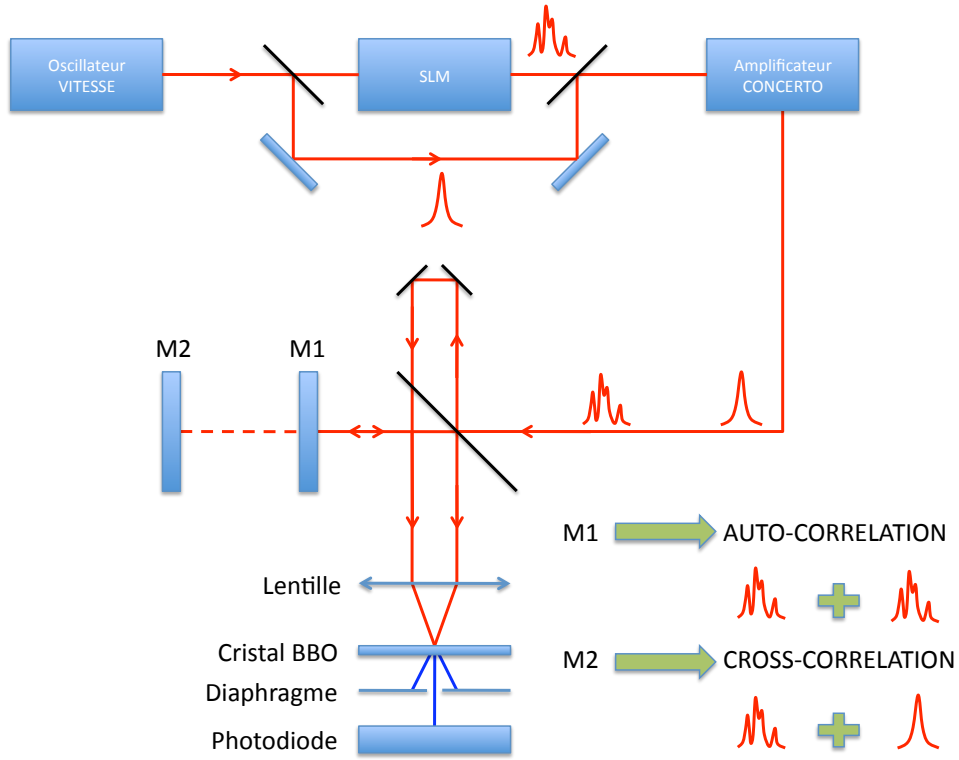
FIGURE 2.7 – Schéma de fonctionnement du corrélateur d'intensité en configuration non-linéaire. M1 miroir pour l'auto-corrélation. M2 miroir pour la cross-correlation.
