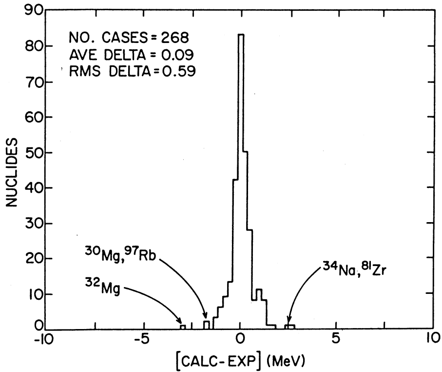
Fig. 1. Histogramme de la différence entre l'excès de masse calculé par Liran et Zeldes et sa valeur expérimentale ( emprunté à P. Hausteин, Hau.84 ).
