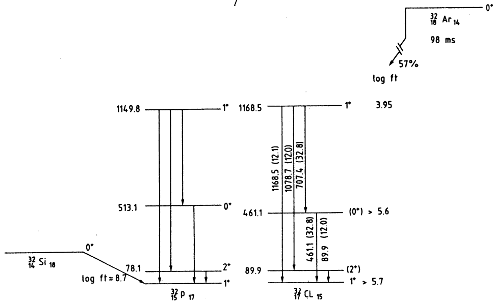
Fig. 1a. Schéma de décroissance des niveaux liés de ^{32}\text{Cl} établi au cours de ce travail et comparé à celui du noyau miroir ^{32}\text{P} .
