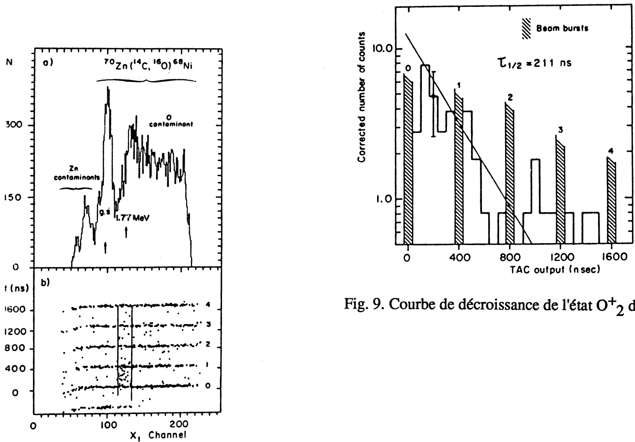
Fig. 8. a) Spectre en rigidité magnétique des ions ^{16}\text{O} . b) Distribution en temps des évènements liés à la désexcitation du niveau \text{O}^+_2 de ^{68}\text{Ni} en fonction de la rigidité magnétique des ions ^{16}\text{O} .
