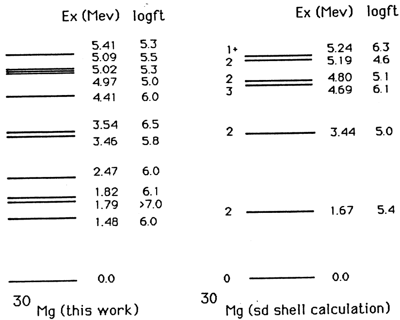
Fig. 25. Comparaison entre les états liés observés dans ^{30}\text{Mg} et ceux prévus par un calcul de modèle en couche dans l'espace de configuration 2s-1d.
