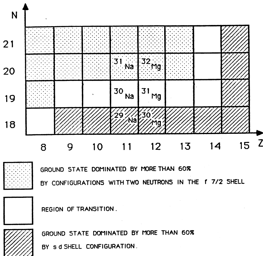
Fig. 26. Carte des configurations des états fondamentaux dans la région de ^{30}\text{Na} établie par Povès ( Pov.87 ).
