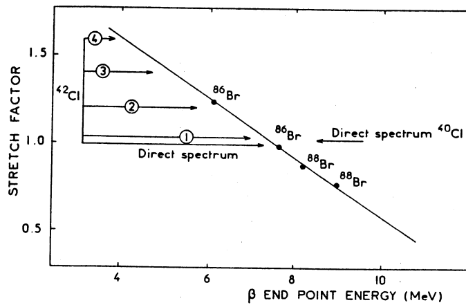
Fig. 6. Calibration du coefficient d'étirement pour a) ^{40}\text{Cl} et b) ^{42}\text{Cl} .
