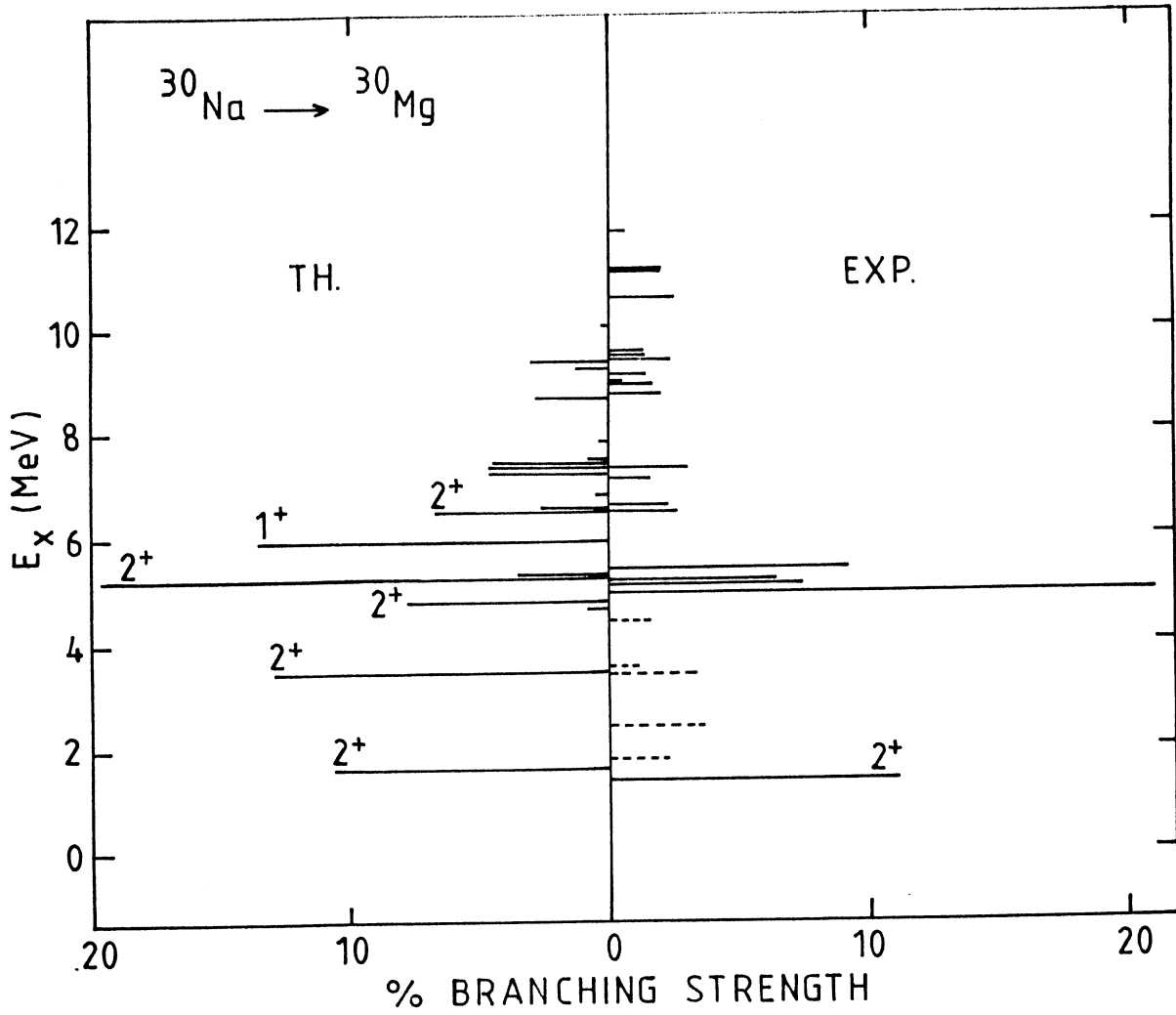
Fig. 30. Comparaison de la force de transition B expérimentale et calculée dans l'espace 2s-1d pour la décroissance de ^{30}\text{Na} .
