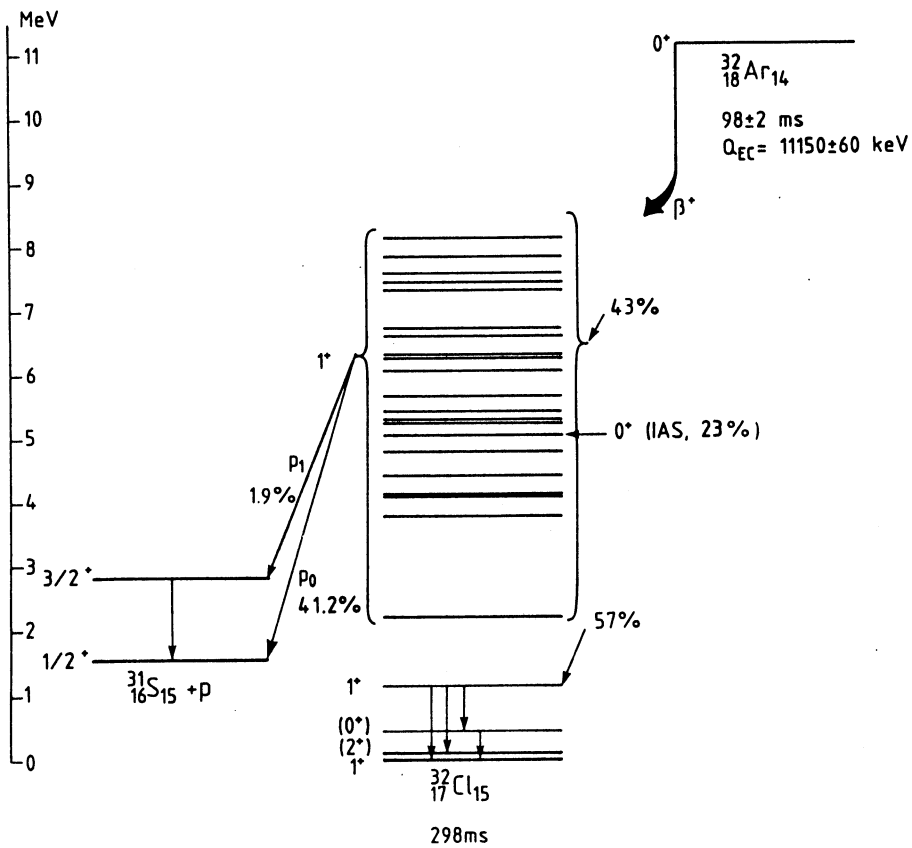
Fig. 1b. Schéma de la décroissance \beta^+ de ^{32}\text{Ar} .
