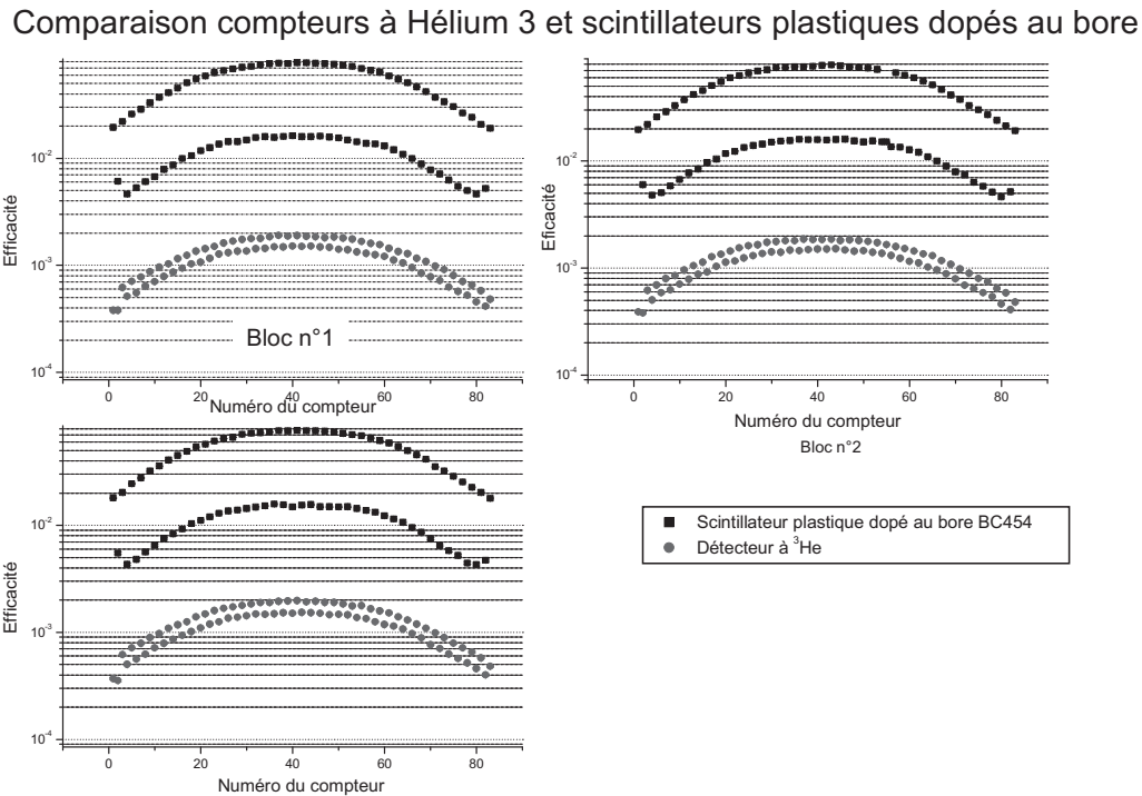
FIG. 7.12: Comparaison de l'efficacité de détection pour des scintillateurs dopés au bore et des détecteurs à base d'Hélium 3 mis en oeuvre dans l'A.C.C.
