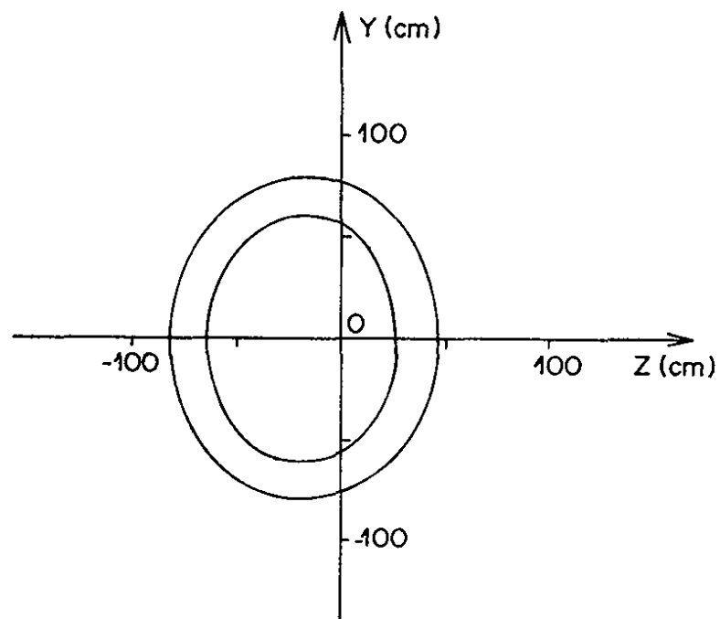
Fig. I.7 : Définition du volume fiduciaire
