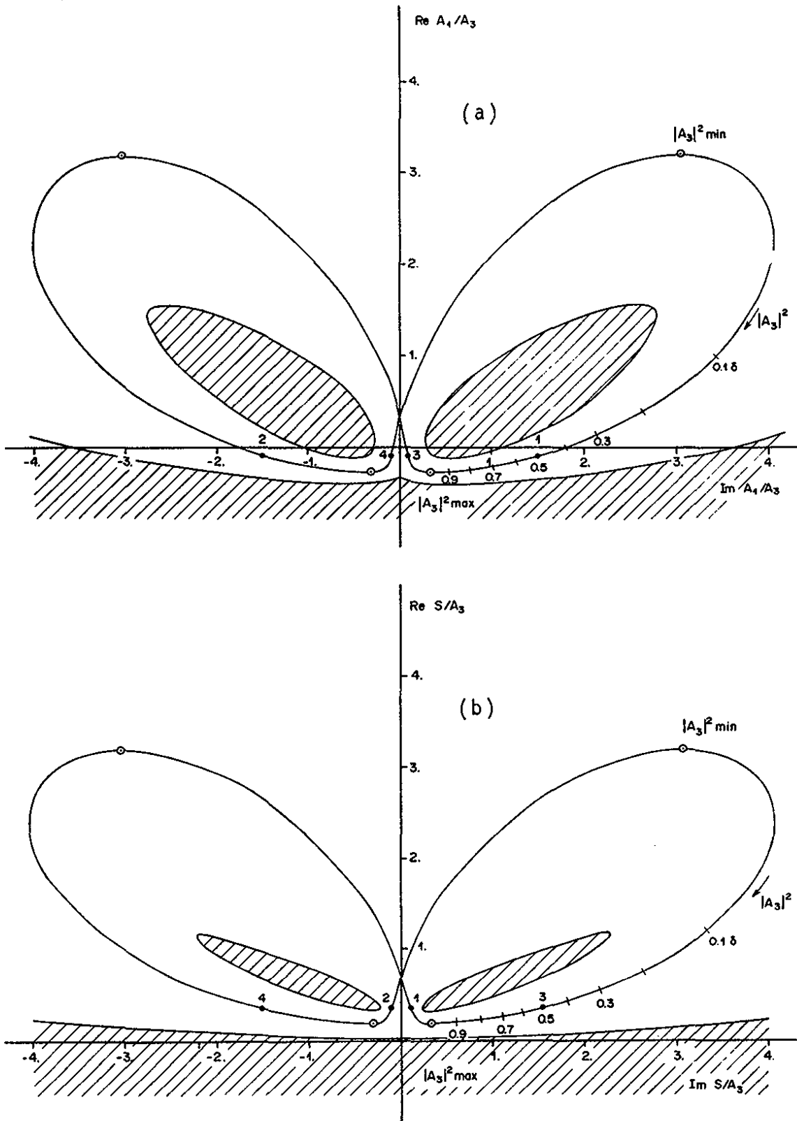
Fig. IV.10 : Variation des vecteurs a) \frac{A_1}{A_3} , b) \frac{S}{A_3}
