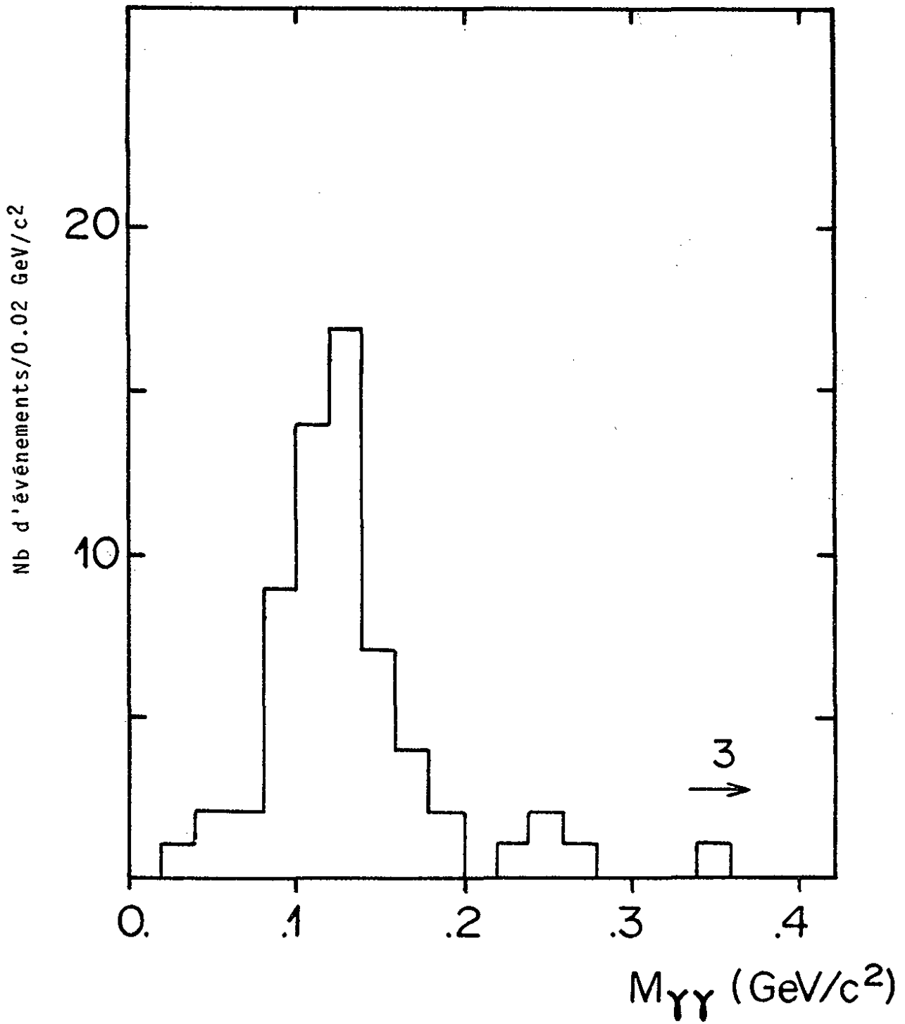
Fig. II.19 : Distribution de la masse gamma-gamma pour les 66 événements à 2 gammas sûrs candidats à la réaction \bar{\nu}_{\mu}p \rightarrow \bar{\nu}_{\mu}p\pi^0
