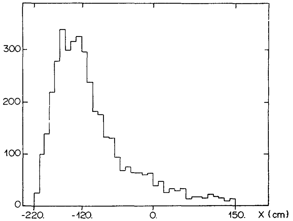
Fig. III.4 : Distribution en X (le long de l'axe du faisceau) pour les protons isolés dans la chambre
