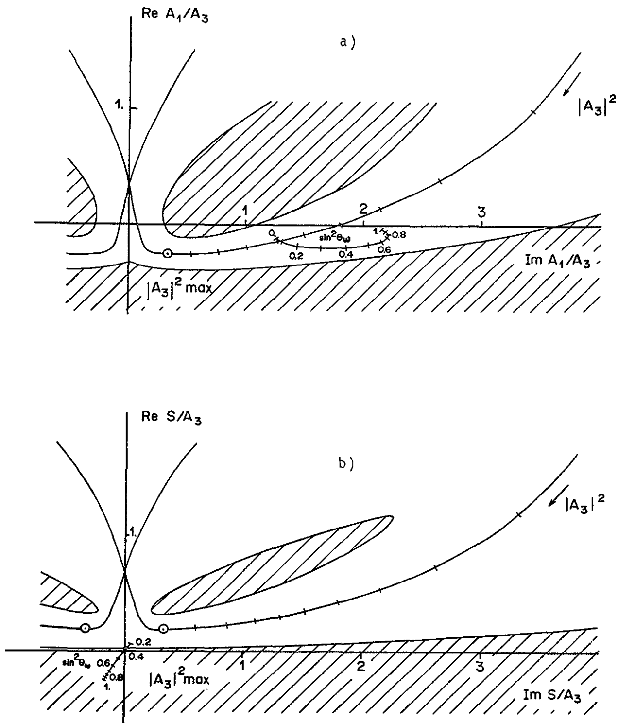
Fig. IV.11 : Prédictions théoriques calculées par G.L. Fogli dans les plans complexes a) A_1/A_3 , b) S/A_3 en fonction de \sin^2 \theta_W et comparaison avec nos résultats expérimentaux.
