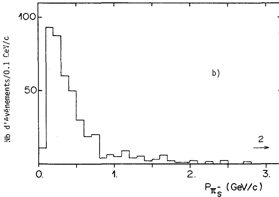
Fig. II.7 : Distribution en impulsion a) des \pi^- ambigus b) des \pi^- sûrs pour les événements de type courant chargé
