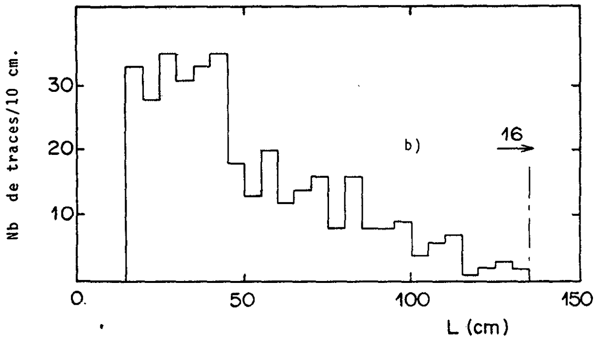
Fig. II.17 : a) Distribution en impulsion, b) Distribution en longueur, des traces négatives qui interagissent
