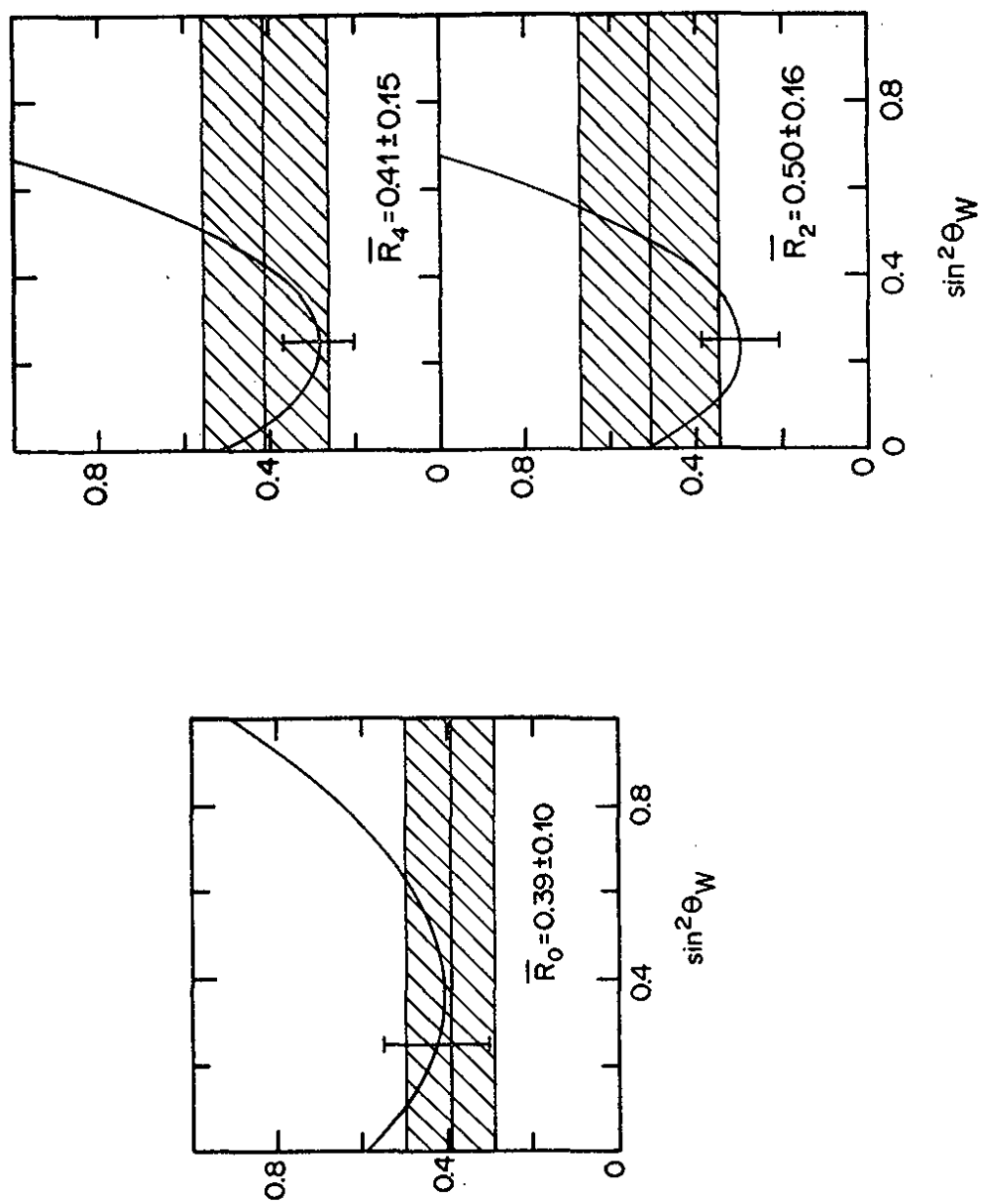
Fig. IV.5 : Prédiction théorique sur les rapports des sections efficaces \bar{R}_0 , \bar{R}_2 et \bar{R}_4 calculés en fonction de \sin^2 \theta_W avec le modèle d'Adler comparées avec nos résultats expérimentaux.
