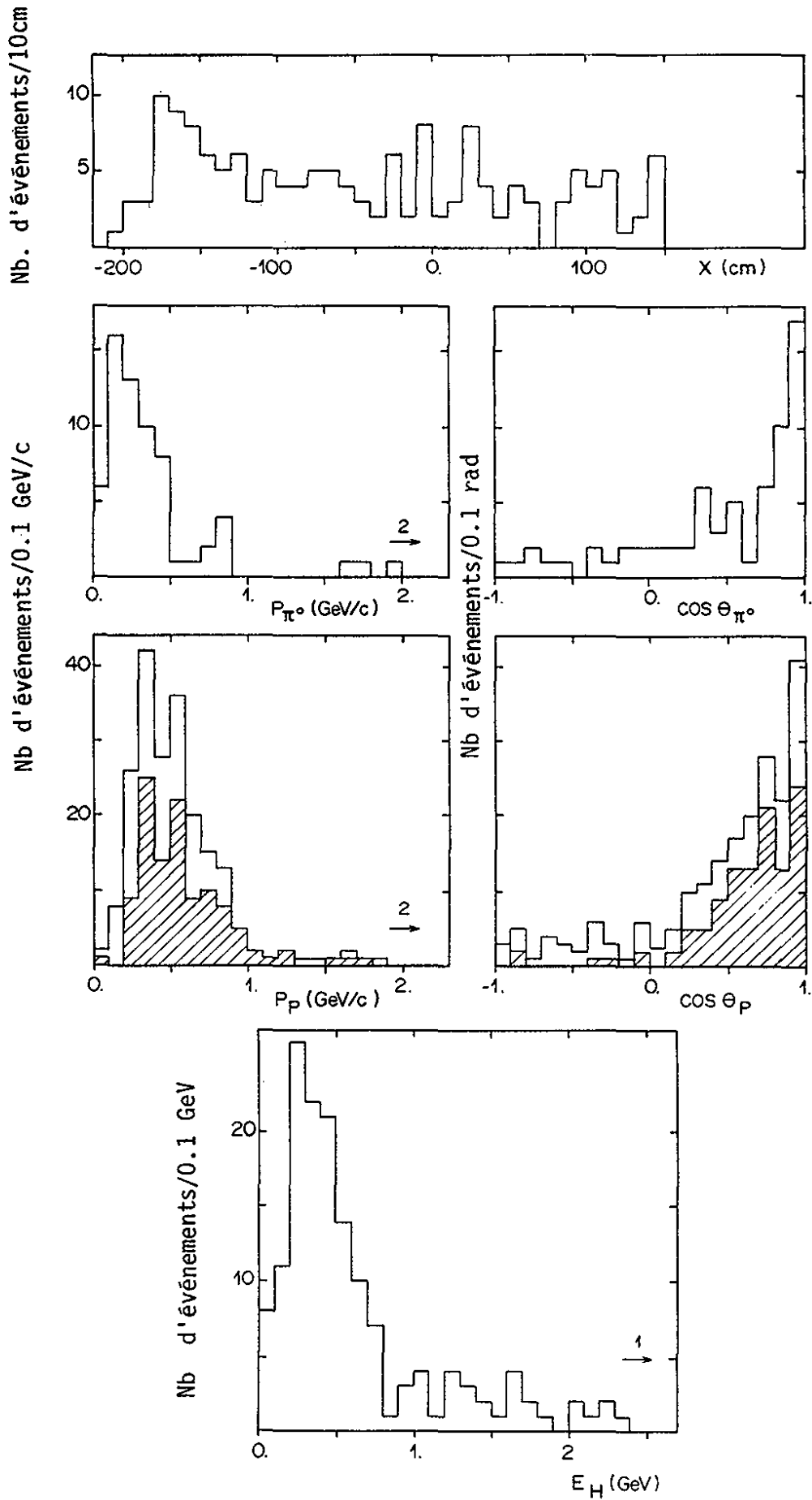
Fig. II.18 : Distributions relatives aux 154 événements sélectionnés pour la réaction \bar{\nu}_{\mu} p \rightarrow \bar{\nu}_{\mu} p \pi^0 Les parties hachurées correspondent aux événements avec 1 seul proton.
