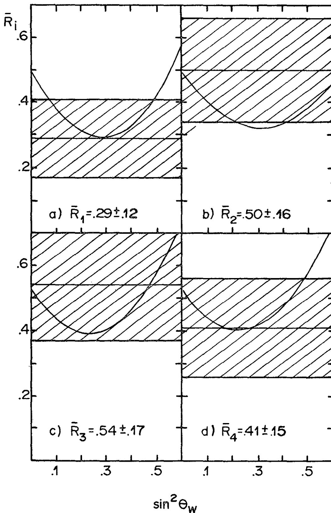
Fig. IV.6 : Prédiction théorique des rapports des sections efficaces \bar{R}_i ( i = 1, 4 ) calculés en fonction de \sin^2 \theta_W avec le modèle de Fogli et Nardulli. Comparaison avec nos résultats expérimentaux.
