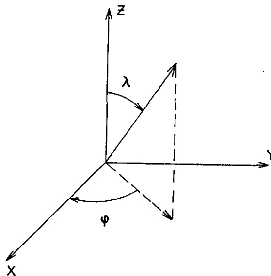
Fig. I.5 : Définition des angles d'enfoncement \lambda et azimuthal \phi dans le système de la chambre
