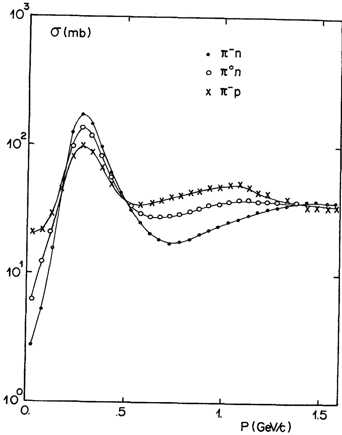
Fig. III.10 : Sections efficaces totales \pi N sur nucléon lié ( P_{fmax} = .250 \text{ GeV}/c )
