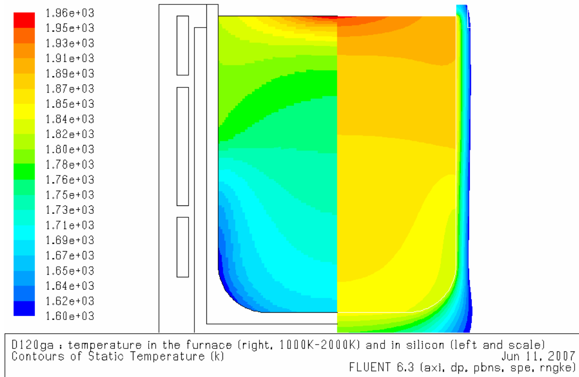
Figure V-19. Champ de température pour un creuset froid de 120mm garni silice avec blocage de l'écoulement et « puissance plasma » appliquée à la surface.
