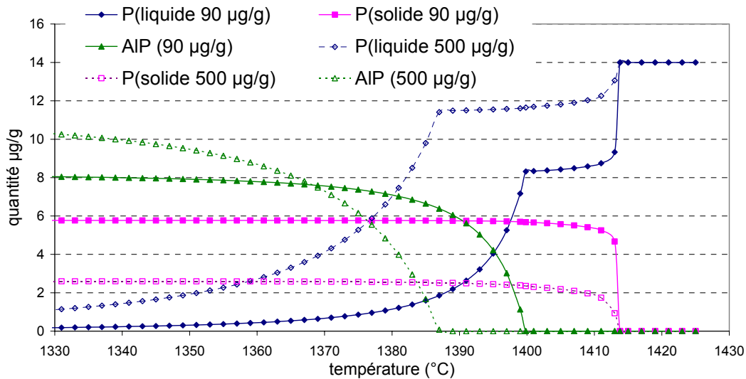
Figure IV-16. Effet de l'ajout d'aluminium sur la ségrégation du phosphore (teneur en Al = 90 ou 500 µg/g, teneur en P = 14 µg/g).
