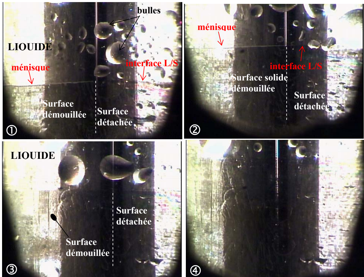
Figure III-4-6. Séquence vidéo de l'expérience de GaSb solidifié sous atmosphère [90%Ar/10%H 2 ] (M18) montrant à la fois du démoillage localisé (surface démoillée avec facettes) et du détachement thermomécanique où la surface du solide est incrustée de bulles.
