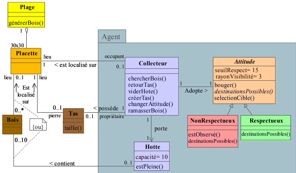
Figure 9-5 : Diagramme de classe de Dracol.
