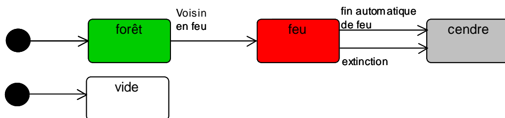
Figure 5-28 : diagramme d'état-transition d'une cellule (fireDiffusion).
