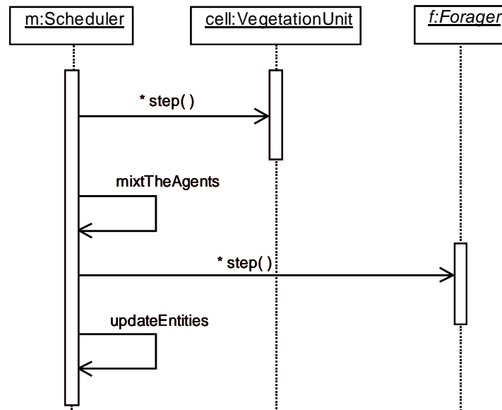
Figure 9 : Diagramme de séquence principal décrivant un pas de temps de ECEC.
