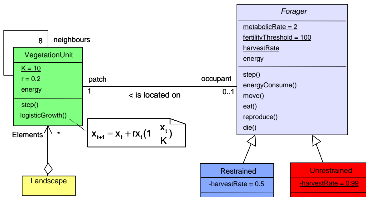
Figure 8 : Diagramme de classe de ECEC
