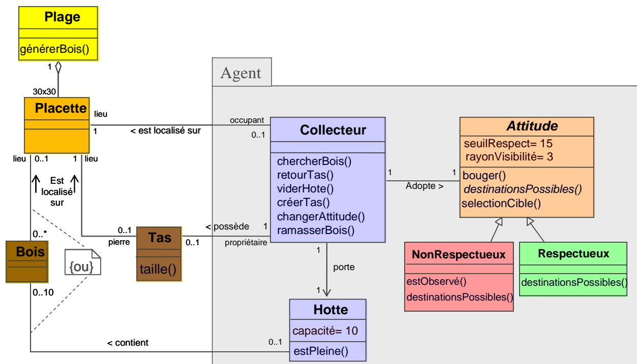
Figure 9-5 : Diagramme de classe de Dricol.
