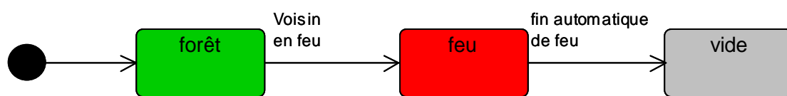
Figure 5-18 : Diagramme d'état-transition d'une cellule.
