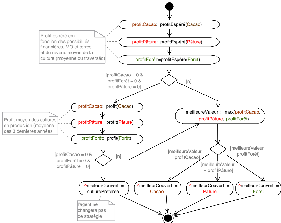
Figure 19 : Diagramme d'activité pour estimer le meilleur couvert (estimerMeilleurCulture)
