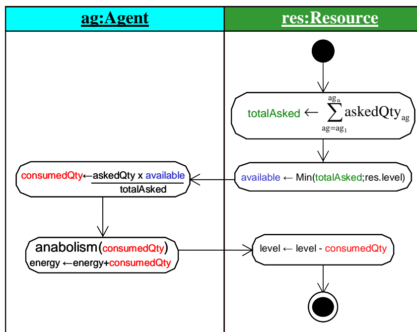
Figure 7 : Diagramme d'activité présentant la distribution de la ressource pour le scénario 2.
