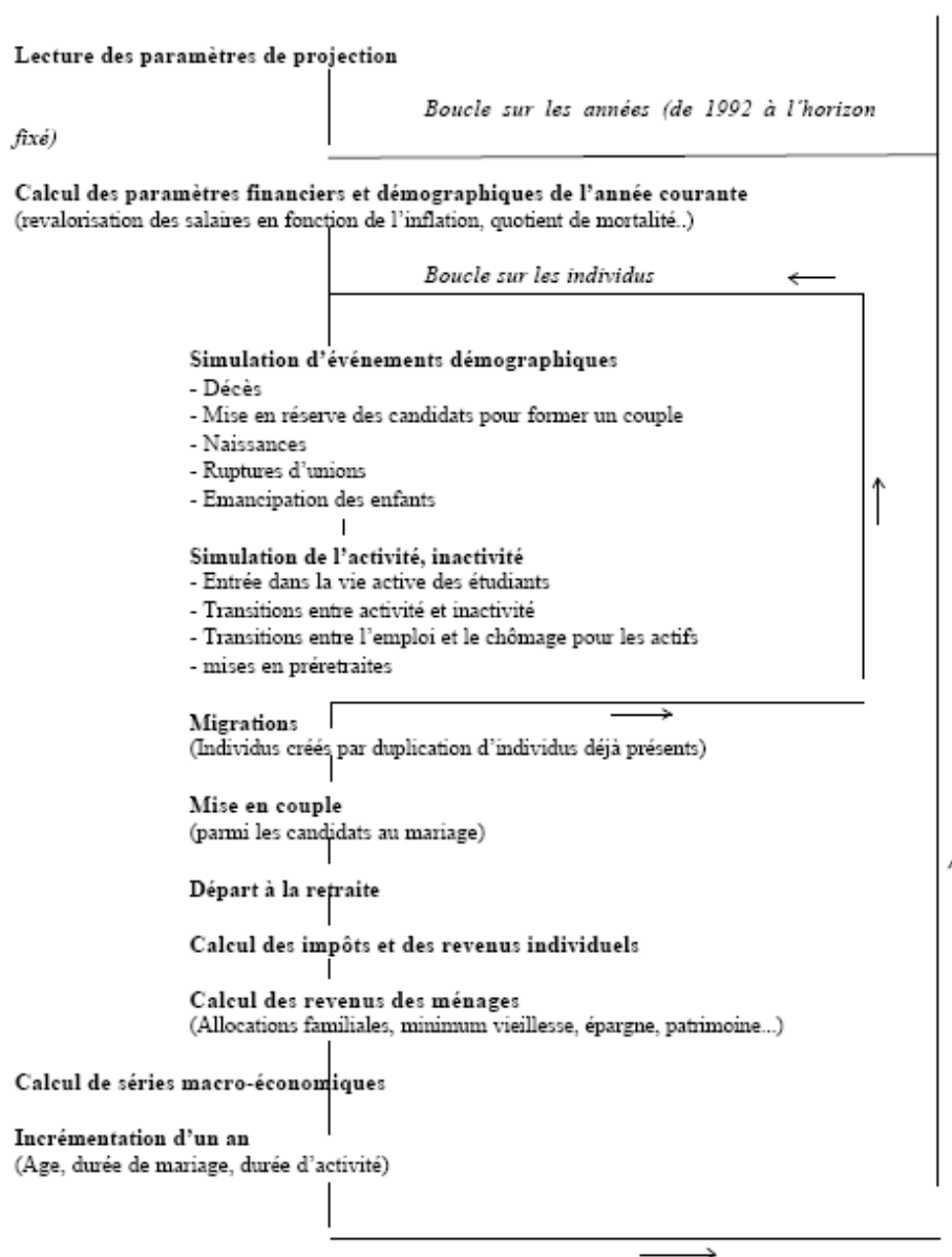
Figure 5-24 : Structure de Destinie : enchaînement des événements démographiques. Figure issue de [INSEE, 1999].
