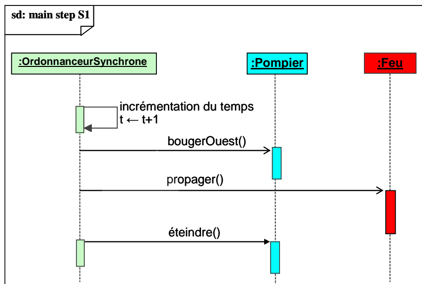
Figure 5-32 : Diagramme de séquence du pas de temps principal de l'ordonnanceur synchrone S1. Au sens d'UML, les flèches symbolisent les messages qui transitent d'une entité vers l'autre. Si l'extrémité de la flèche est pleine, le message est synchrone : cela signifie que l'entité appelante est bloquée jusqu'à la fin de l'exécution du message envoyé. Si l'extrémité de la flèche est creuse, le message est asynchrone : l'entité appelante n'est pas bloquée; elle peut continuer ses activités (envoyer d'autres messages) sans attendre que l'entité exécutant le message ait fini son traitement.
