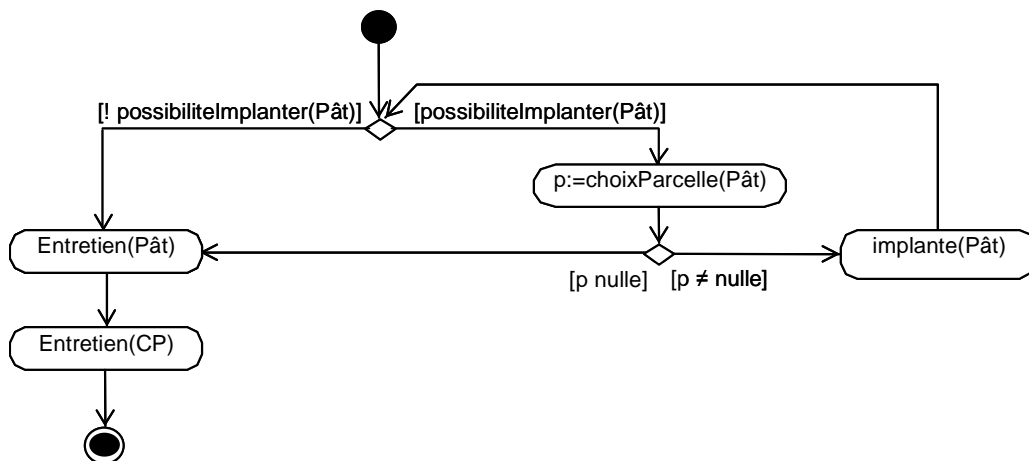
Figure 17 : Diagramme d'activités d'un Eleveur en saison sèche : gestionLots_sèche() .
