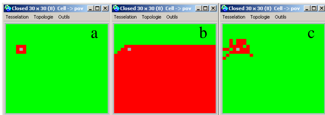
Figure 5-19 : Résultats après un pas de temps de trois gestions différentes du temps: (a) approche synchrone, (b) approche asynchrone non mélangée et (c) approche asynchrone avec mélange aléatoire de l'activation. Les trois simulations ont été effectuées à partir d'un même état initial : une grille de 30x30 en voisinage 8 (Moore), couverte de forêt avec un foyer de départ du feu toujours localisé au même endroit.
