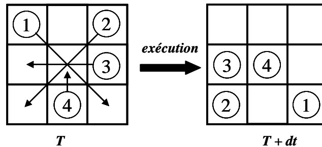
Figure 5-25 : Le problème de la granularité des actions (d'après [Michel et al., 2001]). Les mobiles 1, 2 et 3 se déplacent à des vitesses de deux cases par pas de temps, et le mobile 4, à une vitesse d'une case. Les quatre mobiles se déplaçant vers une position convergente, n'entrent cependant pas en collision.
