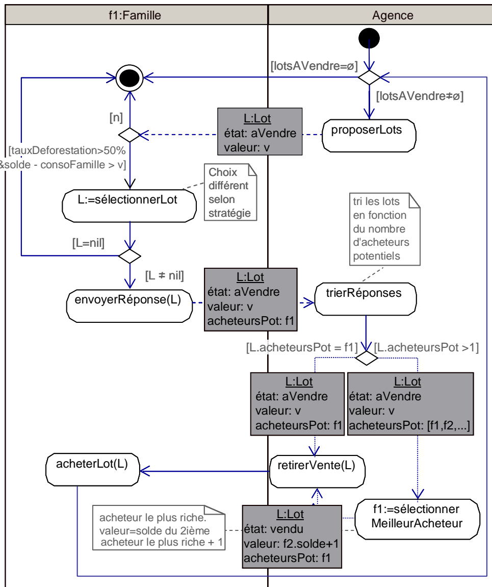
Figure 22 : Vente d'un lot par l'agence, selon un procédé centralisé de type vente au plus offrant (Diagramme d'activités en swimlines et object flow)
