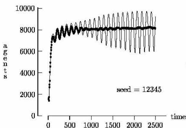
Figure 5-27 : Comparaison de l'évolution asynchrone et synchrone d'une population d'agents, d'après [Lawson et Park, 2000]. Le trait fin représente l'évolution du nombre d'agents par un traitement synchrone alors que le trait épais montre cette même évolution par gestion asynchrone du temps.
