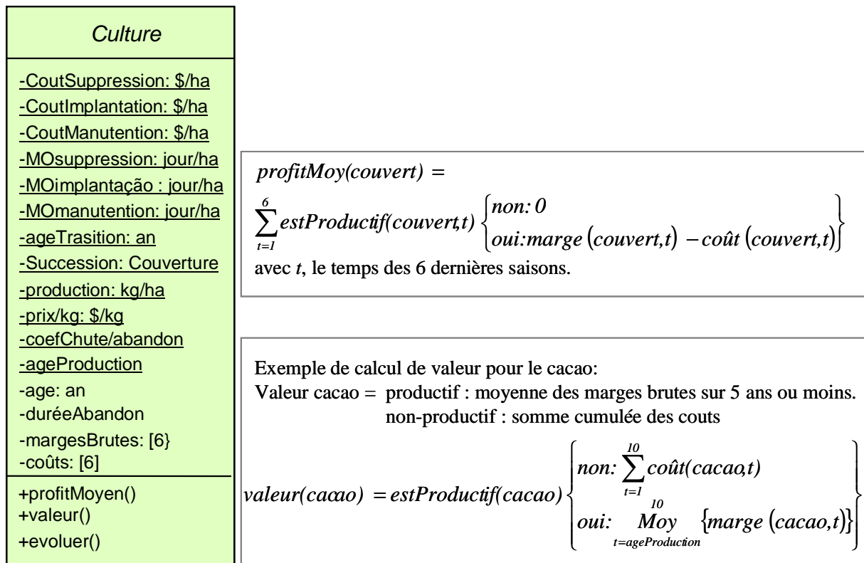
Figure 13 : Tous les attributs de la classe Culture et détails du calcul de la valeur et du profit moyen.
