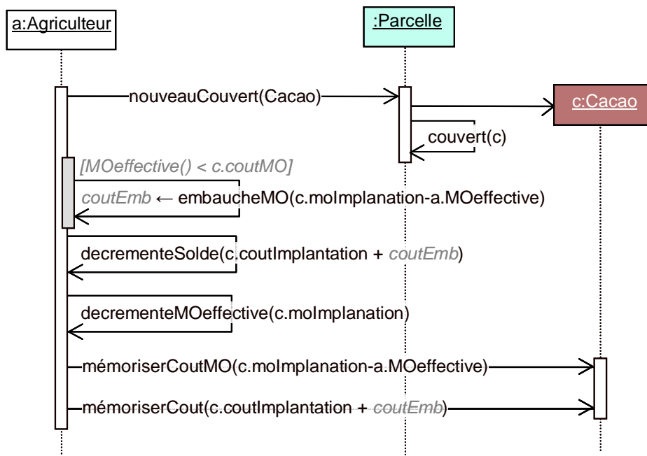
Figure 14 : Implantation d'une culture (Diagramme de séquence)
