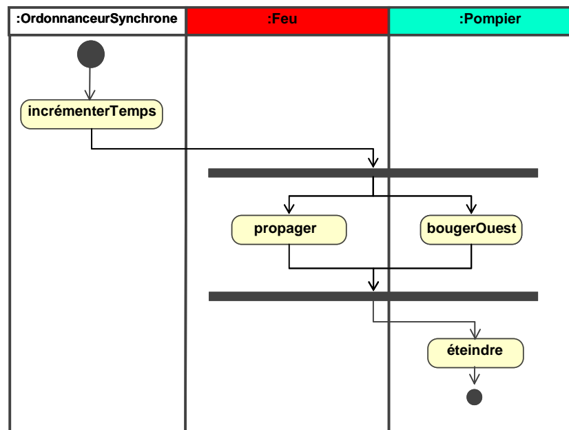
Figure 5-33 : Diagramme d'activité du pas de temps principal de l'ordonnanceur synchrone S1. Les couloirs de natation (swimlanes) permettent de séparer les activités selon les objets qui les exécutent. Les barres de synchronisations permettent d'identifier les activités synchrones (en haut et en bas) des activités asynchrones ou parallèles (au milieu).
