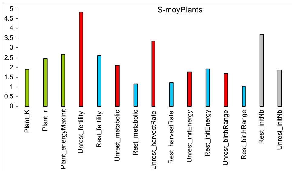
Figure 8-4 : Sensibilité locale pour la sortie "niveau d'énergie moyen des plantes" au dernier pas de temps (500). Les sensibilités (eq. (9.5)) sont présentées en valeur absolue. Les 3 premiers indices correspondent à des attributs attachés à la classe Plant; les indices rouges et bleus clairs indiquent respectivement des attributs des classes UnrestrainedForager et RestrainedForager. Les 2 indices gris clairs sont rattachés à la classe d'initialisation de simulation.
