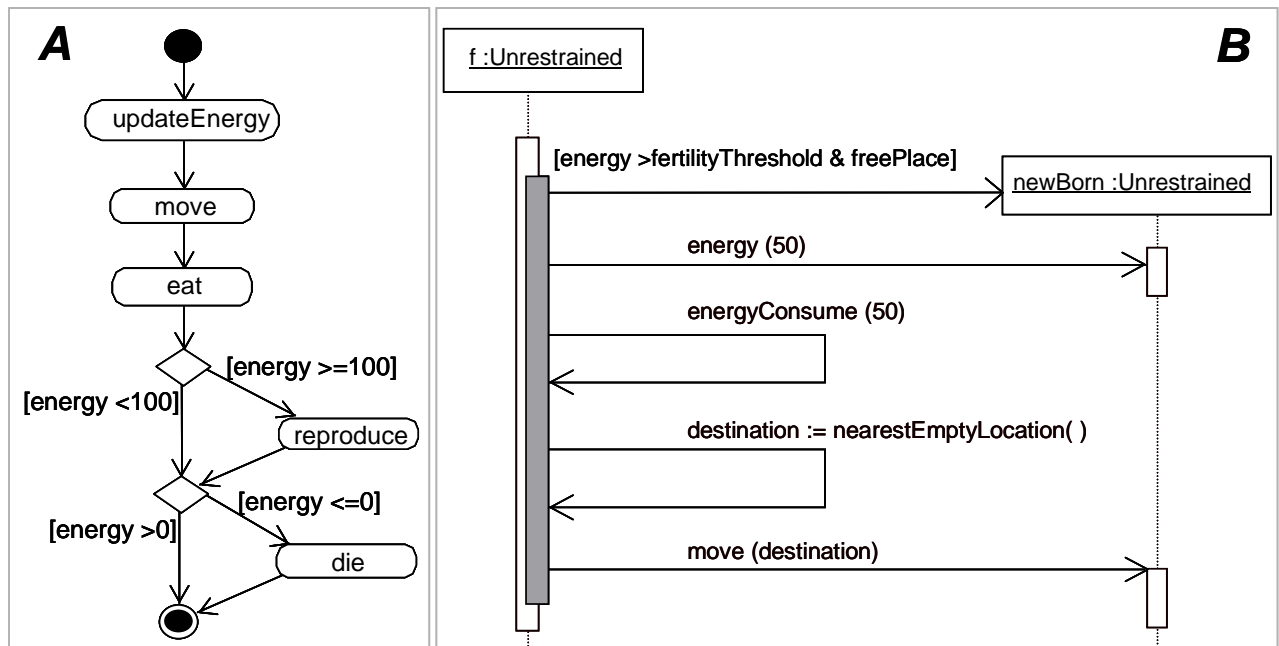
Figure 10 : A- Diagramme d'activité décrivant le "step" d'un ruminant.
