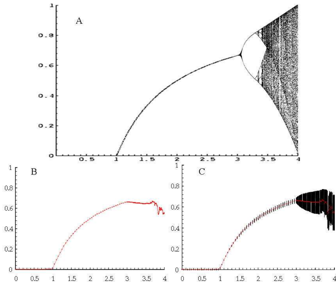
Figure 8-2 : Analyse de sensibilité du modèle de Verhulst discret : X_{t+1}=a.X_t(1-X_t) . Pour chaque simulation de 1000 pas de temps, on étudie les réponses du modèle aux variations du paramètre a qui varie de 0 à 4 en augmentant de 0,001 à chaque simulation :
