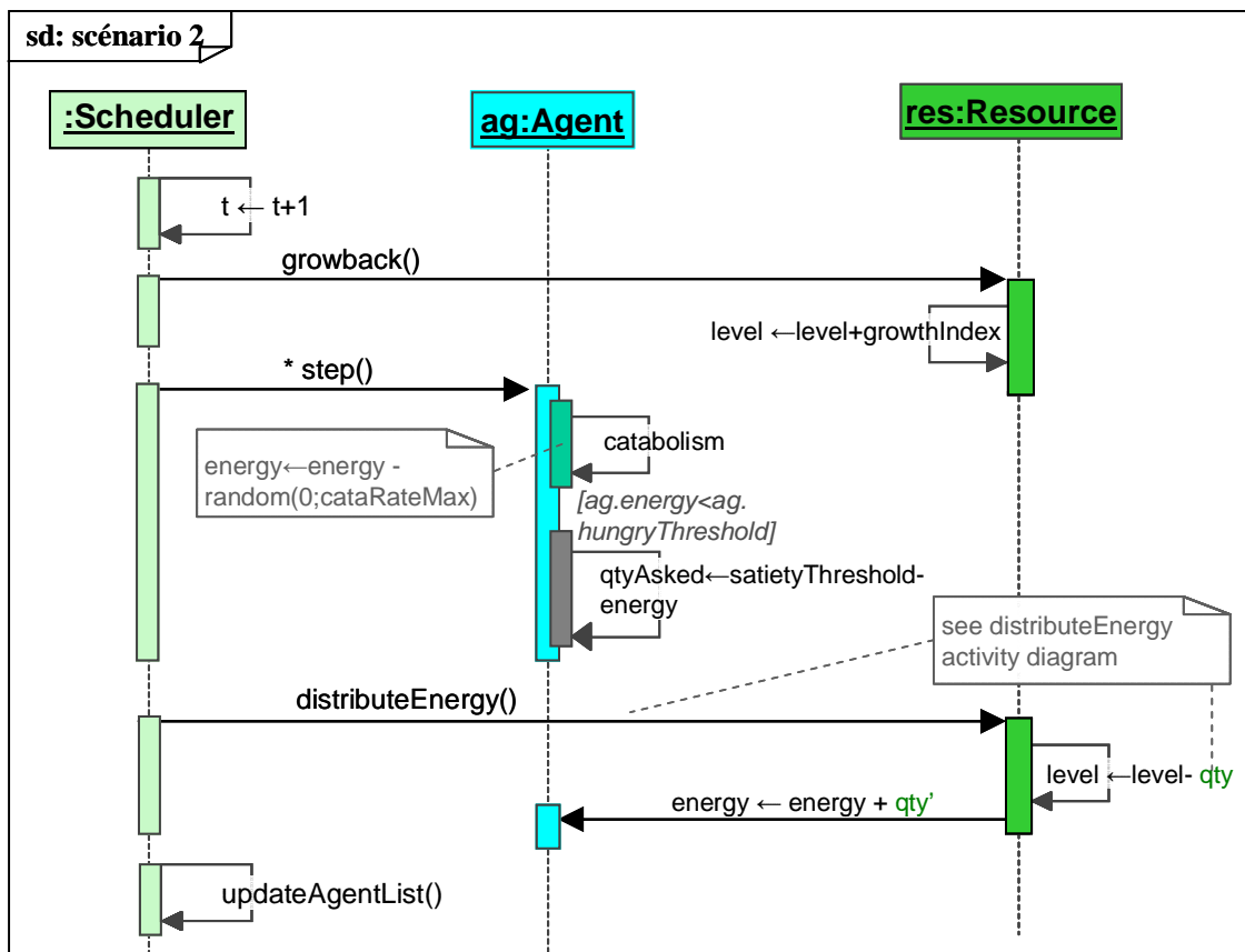
Figure 6 : Diagramme de séquence du scénario 2
