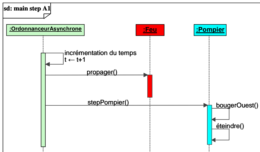
Figure 5-31 : Diagramme de séquence du pas de temps de l'ordonnanceur asynchrone A1.
