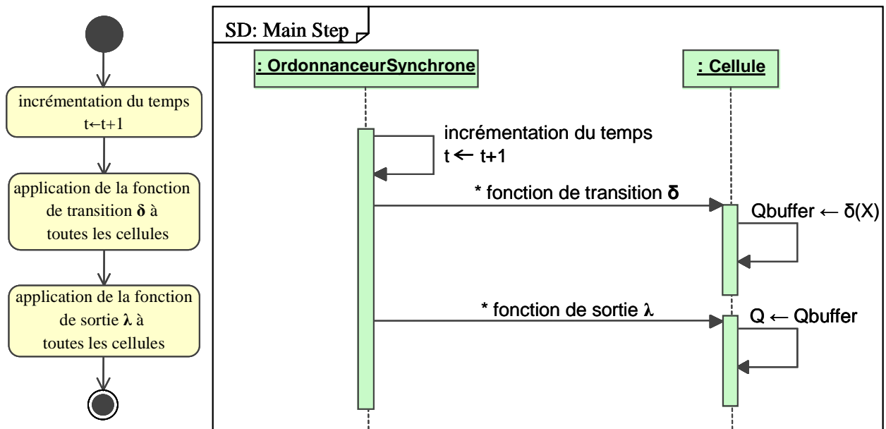
Figure 5-15 : Le cas d'un ordonnanceur synchrone implique deux phases : une phase de calcul de la fonction de transition et une de mise à jour des variables de sortie. A gauche, diagramme d'activité d'un pas de temps d'un simulateur DTSS. A droite, diagramme de séquence d'un pas de temps d'un ordonnanceur synchrone d'automate cellulaire.
