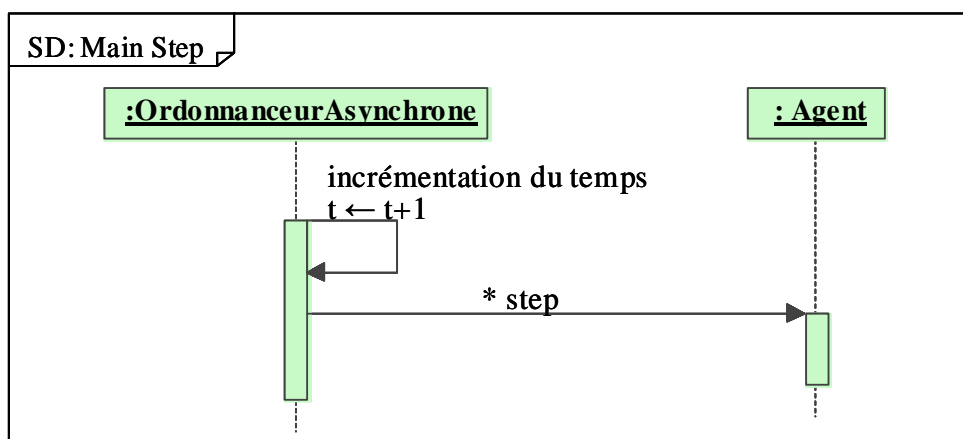
Figure 5-16 : Diagramme de séquence d'un pas de temps d'un ordonnanceur asynchrone. L'astérisque placé devant le "step" signifie en UML que l'appel de méthode est effectué sur toutes les instances d'Agent. Cette représentation ne montre pas quelles sont ces instances, ni dans quel ordre elles sont activées. De mon point de vue, ceci constitue une faiblesse.
