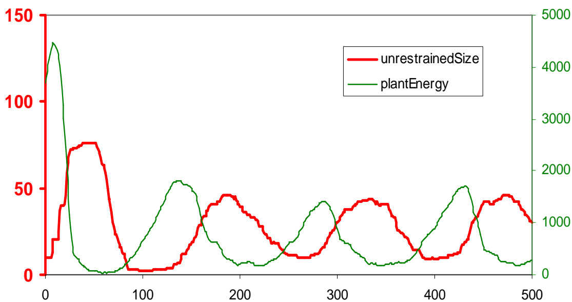
Figure 11 : Evolution de l'énergie des plantes (proies) et de la taille de la population des agents non-restreints (prédateurs)
