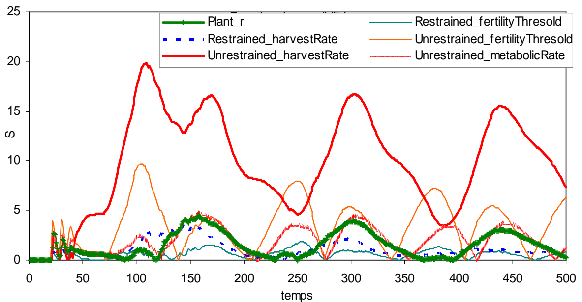
Figure 8-16 : Fonctions de sensibilité des paramètres les plus importants pour la taille de la population des agents non-restreints.
