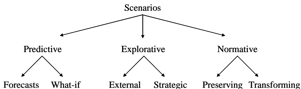
Figure 2-1 : Typologie des scénarios, d'après [Börjeson et al., 2006]
