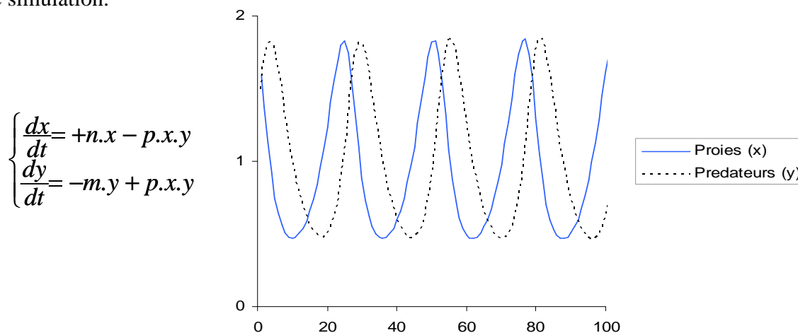
Figure 3-2 : Système d'équation différentiel du modèle de Volterra et évolutions temporelles des populations de proies et de prédateurs qui oscillent de façon endogène au modèle. ( n est le taux de natalité des proies; m , le taux de mortalité des prédateurs ; le paramètre p représente l'efficacité de la prédation. Pour cette simulation particulière, n=m=p=1 ).
