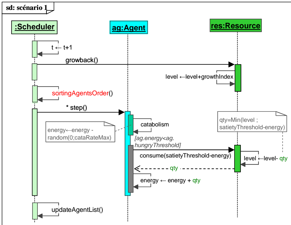
Figure 5 : Diagramme de séquence du scénario 1
