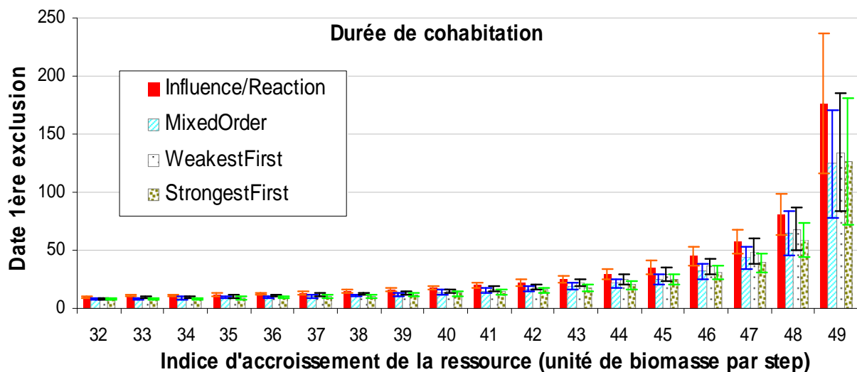
Figure 7-9 : Graphe comparatif des durées moyennes de cohabitation de 10 agents en fonction de la croissance de la ressource. La durée moyenne avant exclusion sert d'indicateur pour comparer quatre scénarios de gestion des interactions : gestion selon le principe "Influences-Réaction" (en rouge), gestion standard par prélèvements directs par les agents (hachuré), gestion standard commençant par les agents les plus faibles (blanc) et gestion standard commençant par les plus forts (en pointillé).
