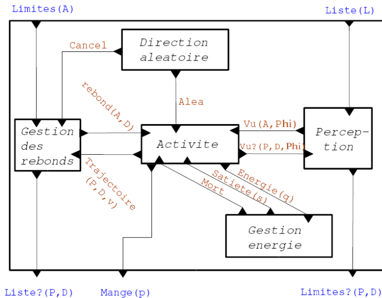
Figure 5-13 : Représentation graphique du modèle couplé de l'agent copépoce. En bleu, figurent les événements externes attachés aux ports d'entrée ou de sortie du modèle couplé. Les événements véhiculés par les connexions internes figurent en rouge. (D'après [Duboz, 2004])
