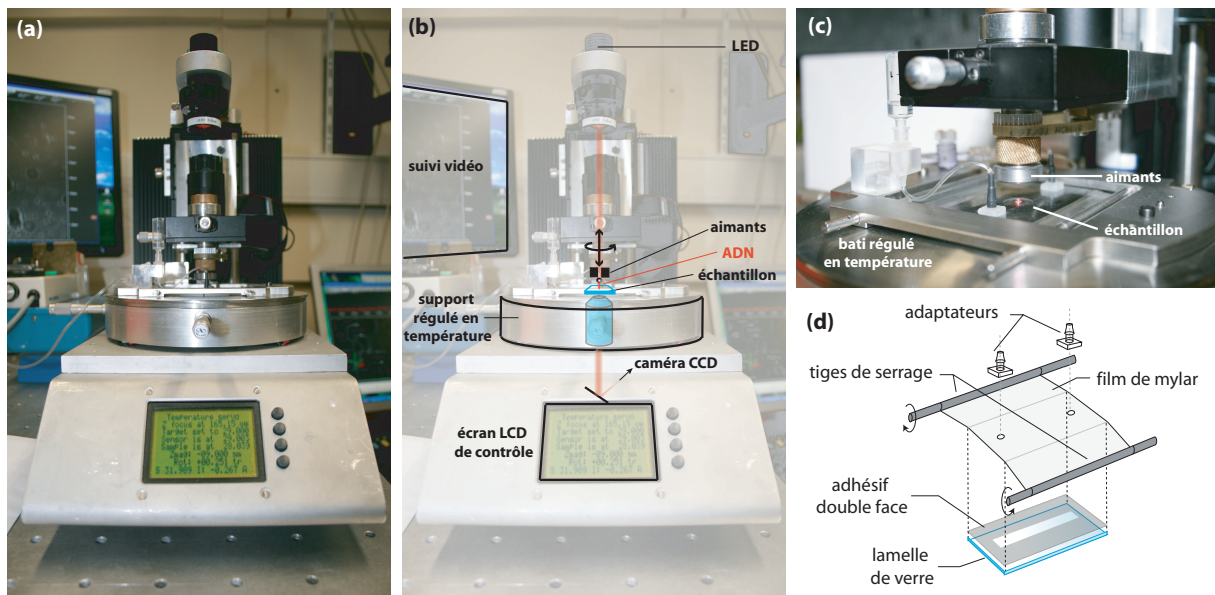
FIGURE 5.3 – Le dispositif des pinces magnétiques. (a) Photo de l'ensemble du dispositif. (b) Schéma de principe. Une LED est focalisée sur l'échantillon. La zone d'intérêt est imagée par un objectif sur une caméra CCD. Des aimants placés au-dessus de l'échantillon permettent d'exercer une force et une contrainte de torsion sur une bille magnétique ancrée à la surface par une molécule d'ADN (lien rouge). La bille, les aimants et la molécule d'ADN ne sont pas représentés à l'échelle. (c) Gros plan de l'échantillon. Des puits permettent l'injection de fluide jusque dans la chambre microfluidique dans laquelle se déroule l'expérience. Les aimants placés au-dessus de l'échantillon peuvent être translattés verticalement et entraînés en rotation autour de l'axe vertical. (d) Principe d'assemblage de la micro-chambre. Un microcanal est creusé au centre d'un film adhésif double-face. Celui-ci est placé entre une lamelle de verre et un film de mylar tendu entre deux tiges. Deux trous percés dans le mylar permettent, après y avoir collé des adaptateurs, d'injecter les fluides par des tubes. Les dimensions du canal ainsi créé sont de près de 50 \text{ mm} \times 5 \text{ mm} \times 60 \mu\text{m} , soit un volume de près de 15 \mu\text{L} .
