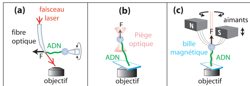
FIGURE 4.3 – Schéma de principe (a) de la microfibre optique, (b) des pinces optiques, (c) des pinces magnétiques.
