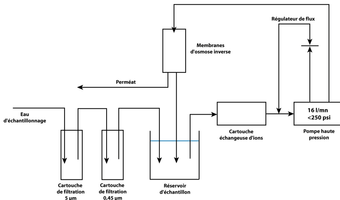
Figure 1.5: Représentation schématique du montage de concentration de la MOD d'échantillons d'eau par le procédé d'osmose inverse
