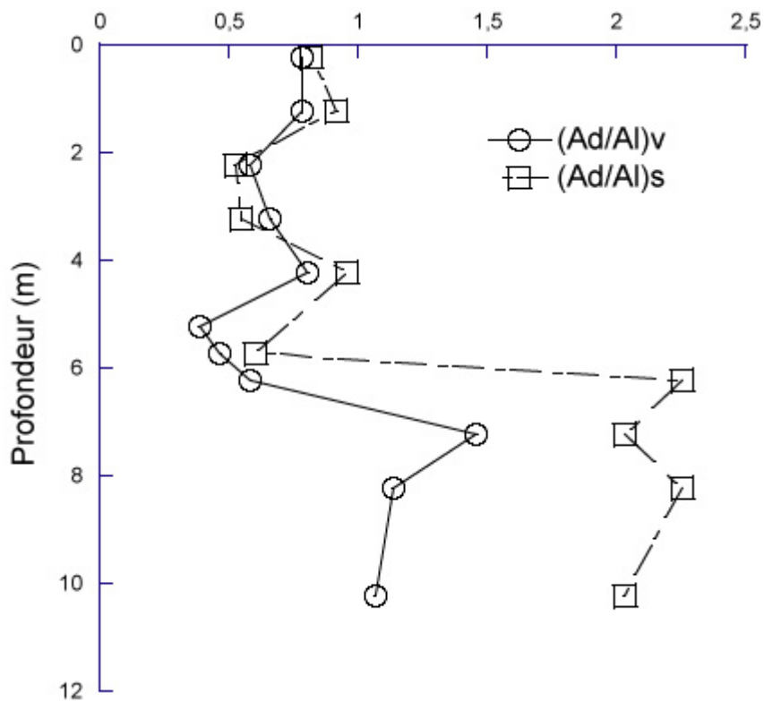
Figure 3.11: Évolution des rapports acide/aldéhyde des familles vanillyles et syringyles dans un affleurement de la zone de recharge de l'aquifère des sables de l'Astien
