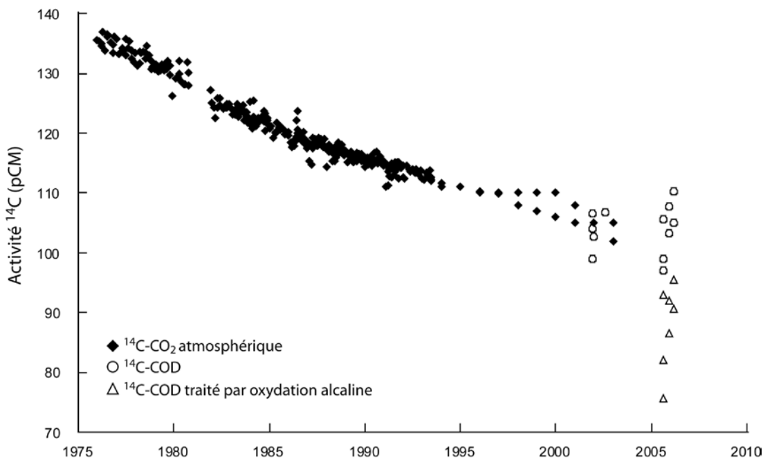
Figure 2.3: Activités ^{14}\text{C} du \text{CO}_2 atmosphérique entre 1975 et 2003, du COD de la rivière des Outaouais et du fleuve Saint-Laurent. Les teneurs en ^{14}\text{C} du COD de l'année 2002 proviennent de Lamontagne, (2004)
