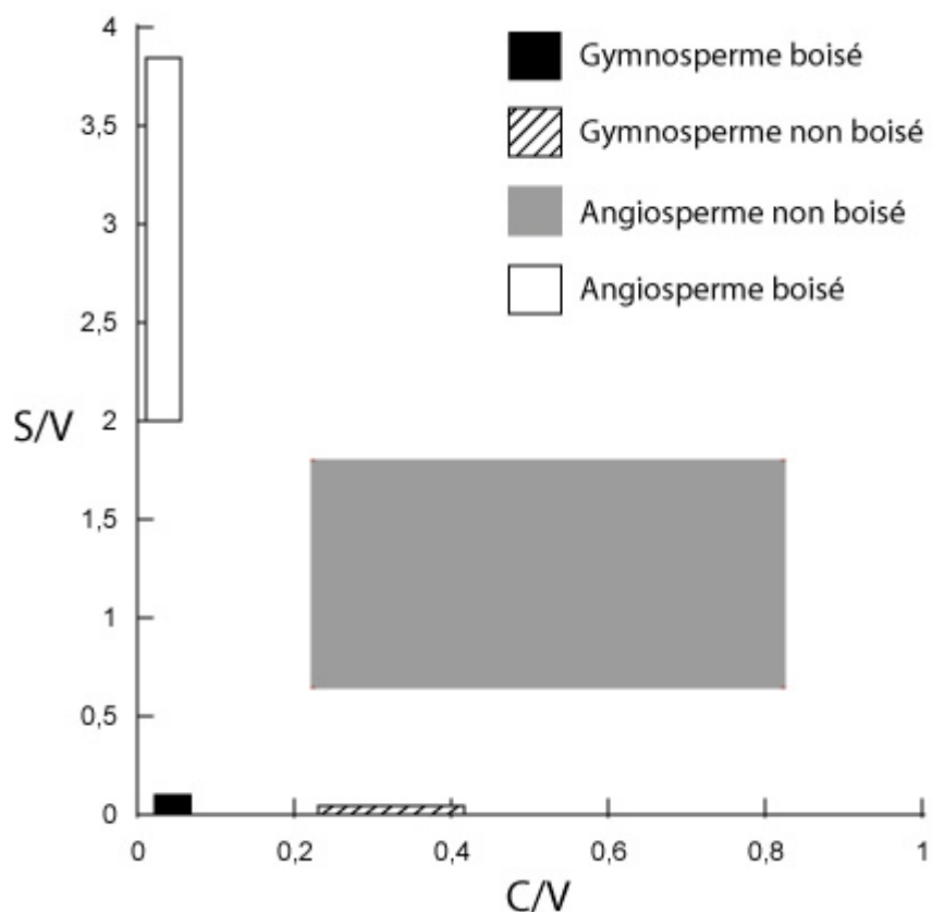
Figure 1.7: Diagramme illustrant les gammes de valeurs des rapports S/V et C/V pour des sources pures d'angiospermes et de gymnospermes
