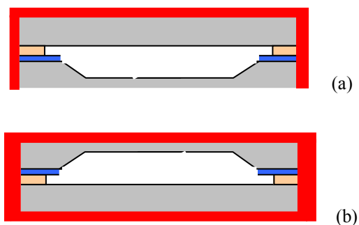
Fig. 4.17 Dépôt de la couche hermétique pour les boîtiers étanchés : (a) dépôt d'une couche de parylène de 5\mu\text{m} d'épaisseur sur la face arrière ; (b) dépôt d'une couche de parylène de 5\mu\text{m} d'épaisseur sur la face avant des boîtiers
