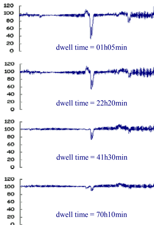
Fig. 4.27 Spectres FTIR du gaz contenu dans un boîtier de 20 \text{mm}^3 , avec une épaisseur de scellement de 100 \mu\text{m} , pris à intervalles réguliers après la fin de l'exposition au \text{N}_2\text{O}
