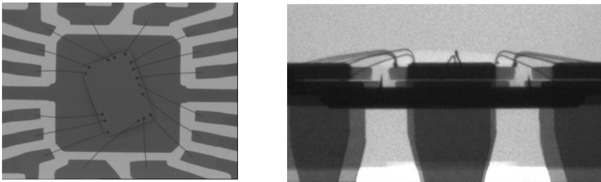
Fig. 1.5 Images RX du microcâblage d'un boîtier QFP
