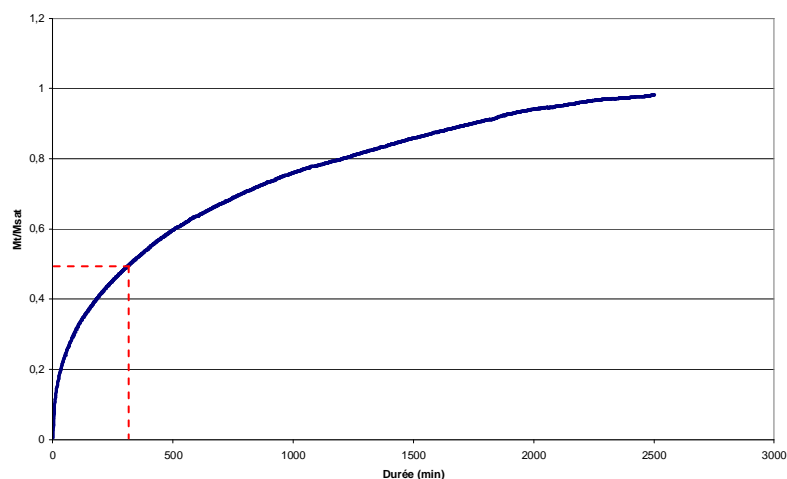
Fig. 3.6 Représentation de la courbe M_t/M_\infty
