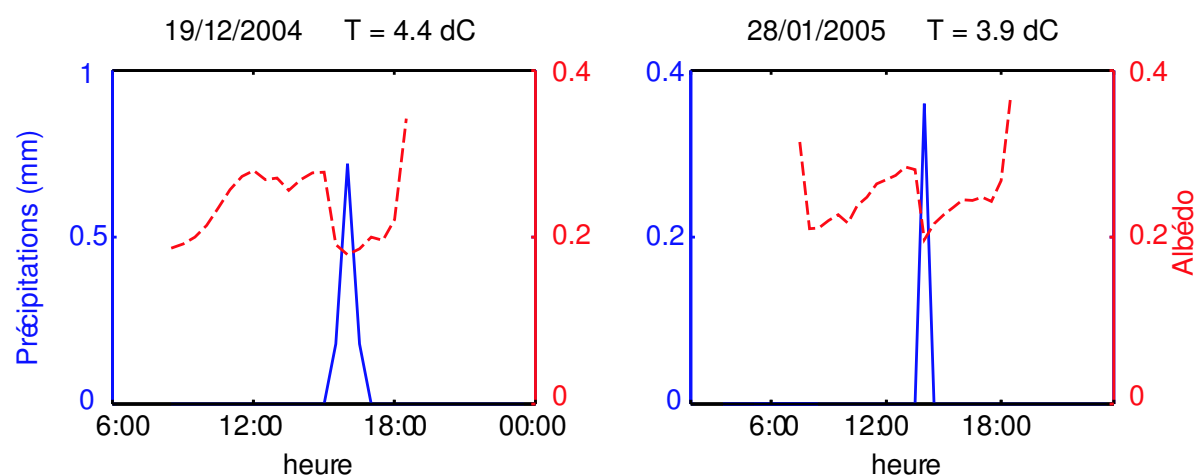
FIG. 3.2. Exemples de variations de l'albédo observé lors de deux événements pluvieux le 19/12/2006 et le 28/01/2006. En rouge pointillé : albédo; en bleu trait plein : précipitations. Les mesures sont au pas de temps demi-horaire. Les variations d'angle zénithal faussent l'interprétation de l'albédo en dehors de la plage 9h-16h. La température non ventilée est donnée pour le maximum des précipitations, et indique que les précipitations sont bien liquides à ce moment là.
