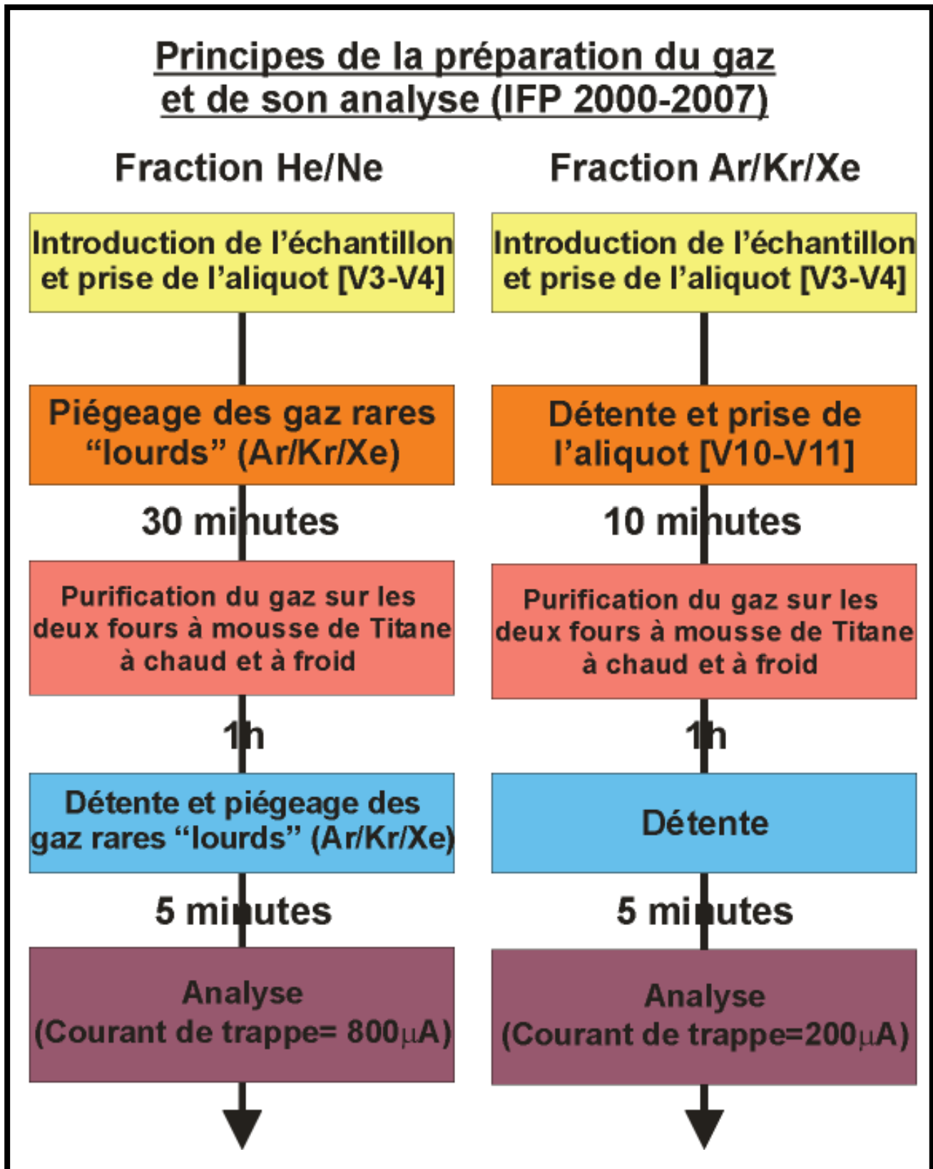
Figure A.6: Protocole analytique de préparation du gaz sur la ligne de l'IFP (2000-2007).
