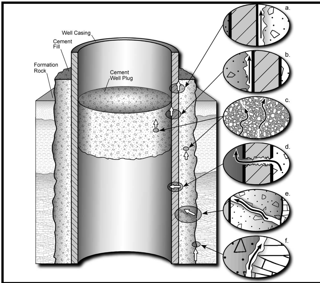
Figure 3.7 : Les chemins potentiels des fuites dans les puits abandonnés (Gasda et al., 2004b).
