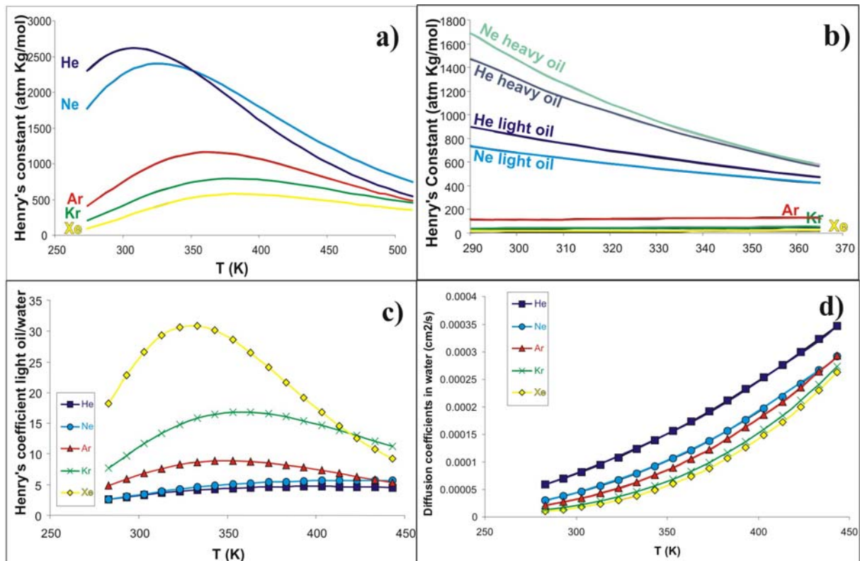
Figure 2.3 : Constantes de Henry des différents gaz rares en fonction de la température, dans le cas d'une eau douce, d'une huile lourde et d'une huile légère.
