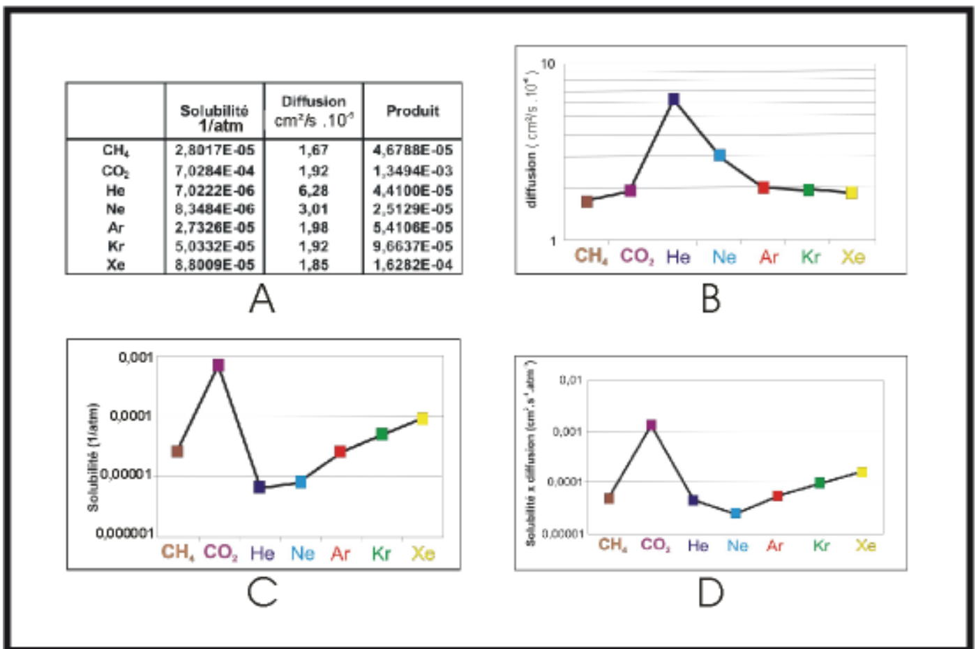
Figure 4.3: - A - Tableau des valeurs de solubilité (en atm -1 ) et de diffusion (10 -5 .cm 2 s -1 ) dans l'eau douce à 20°C et à 1 atmosphère pour le CO 2 , le CH 4 , et les gaz rares.
