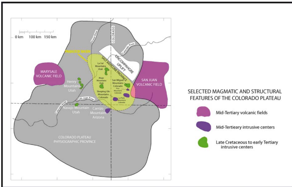
Figure 3.69: Centres intrusifs et épisodes magmatiques ayant affecté la partie nord du Plateau du Colorado. (Image de J.-L. Faure, d'après Ross, 1983).
