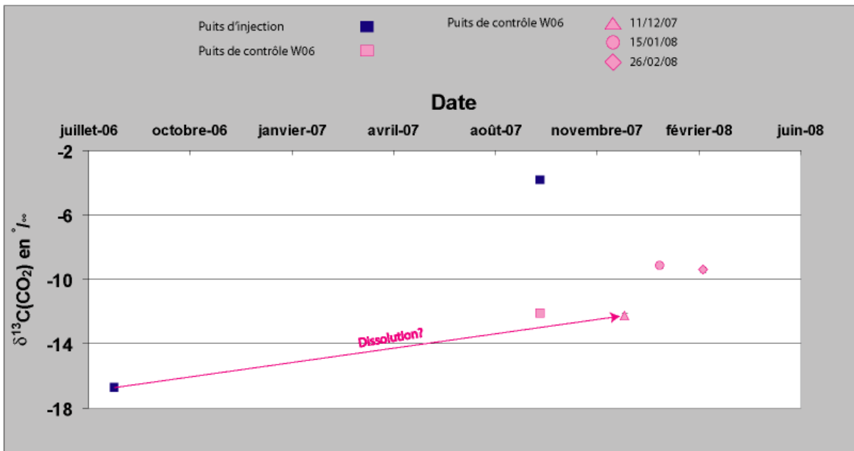
Figure 4.52: Evolution des rapports CO_2/\beta He et du \delta^{13}C(CO_2) au cours du temps pour le gaz injecté et les gaz prélevés sur le puits de contrôle W06.
