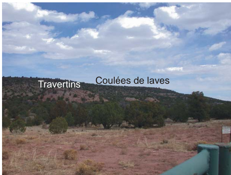
Figure 3.61: Dépôt de travertins et coulées basaltiques à proximité du puits 10-22.
