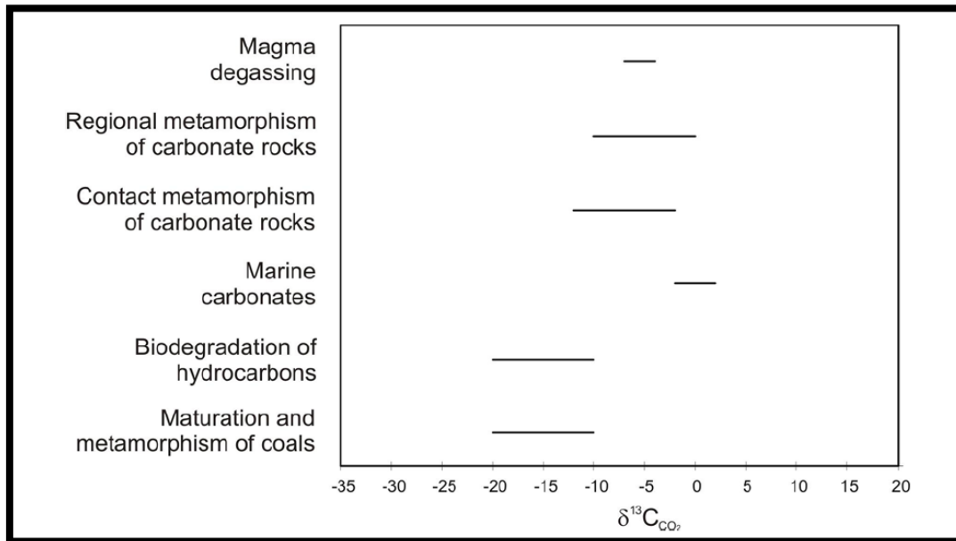
Figure 3.4: Les compositions isotopiques des différentes sources de CO 2 naturel (D'après IEA, 2005).
