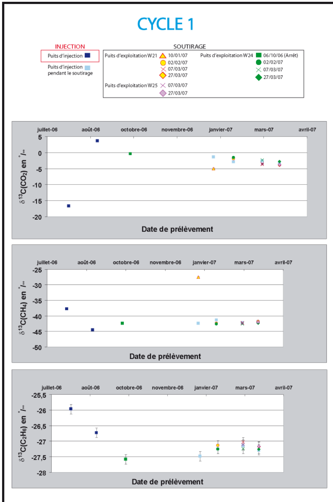
Figure 4.13: Evolution au cours du temps de la composition isotopique des gaz injectés et soutirés au cours du cycle 1. Cas du \delta^{13}\text{C}(\text{CO}_2) , \delta^{13}\text{C}(\text{CH}_4) et du \delta^{13}\text{C}(\text{C}_2\text{H}_6) .
