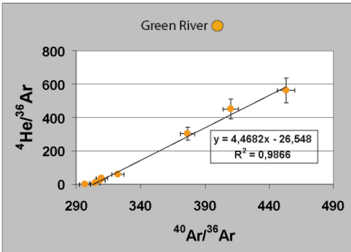
Figure 3.72: Diagramme ^4\text{He}/^{36}\text{Ar} versus ^{40}\text{Ar}/^{36}\text{Ar} pour les événements de Green River.
