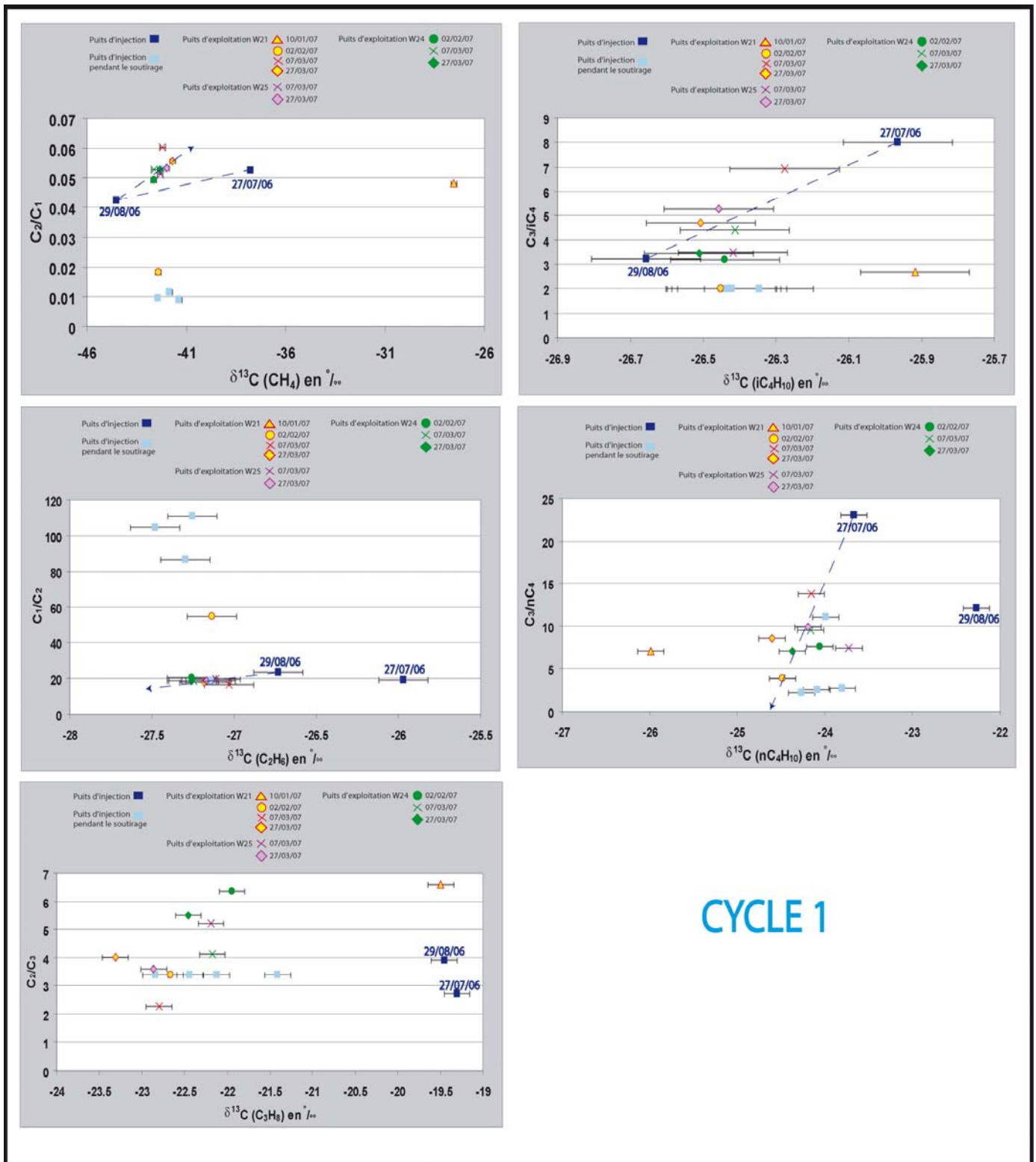
Figure 4.20: Diagrammes de mélange C_2/C_1 versus \delta^{13}\text{C}(\text{CH}_4) , C_1/C_2 versus \delta^{13}\text{C}(C_2H_6) , C_2/C_3 versus \delta^{13}\text{C}(C_3H_8) , C_3/iC_4 versus \delta^{13}\text{C}(iC_4H_{10}) et C_3/nC_4 versus \delta^{13}\text{C}(nC_4H_{10}) représentant les gaz injectés et soutirés au cours du cycle 1. Dans certains d'entre eux, les gaz échantillonnés au cours de l'injection sont des pôles de mélange (diagrammes C_3/iC_4 versus \delta^{13}\text{C}(iC_4H_{10}) , C_2/C_1 versus \delta^{13}\text{C}(\text{CH}_4) ; C_1/C_2 versus \delta^{13}\text{C}(C_2H_6) ; C_3/nC_4 versus \delta^{13}\text{C}(nC_4H_{10}) ), alors que le diagramme C_2/C_3 versus \delta^{13}\text{C}(C_3H_8) met en évidence des pôles inconnus.
