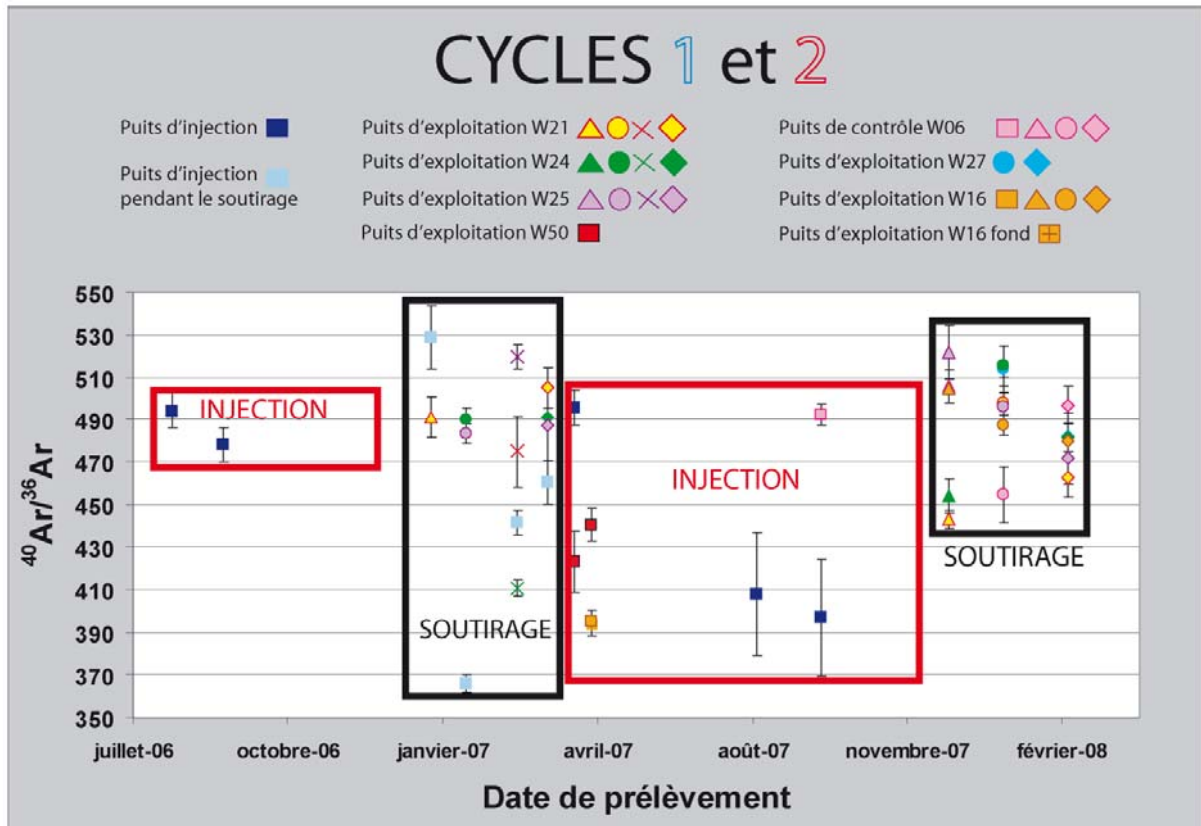
Figure 4.25: Évolution des rapports isotopiques ^{40}\text{Ar}/^{36}\text{Ar} en fonction du temps. Les périodes d'injection et de soutirage sont reportées.
