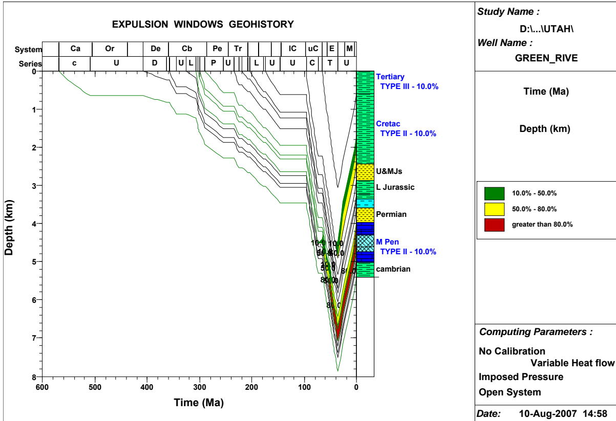
Figure 3.80: Modèle Génex 1D de la région de Green River.
