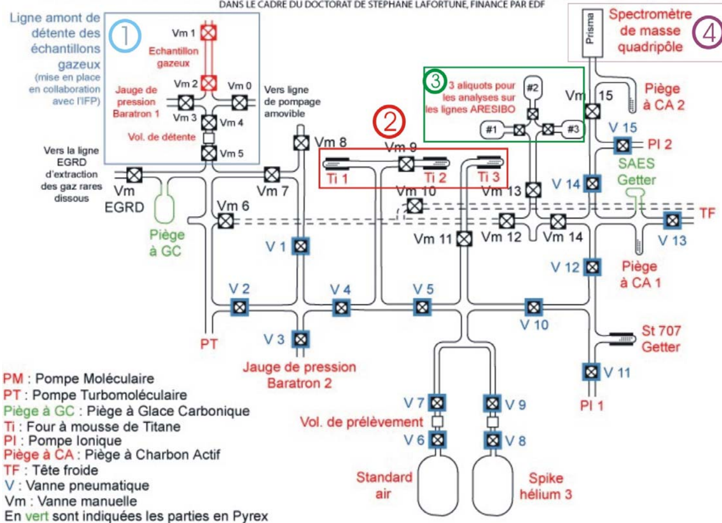
Figure A.9: Purification et analyse des gaz sur la ligne Garodiox (Lafortune, 2007).
