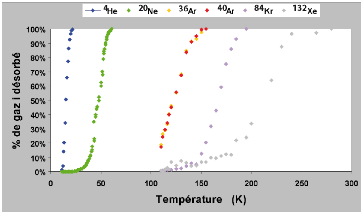
Figure A.8: Courbes expérimentales de désorption des gaz rares.
