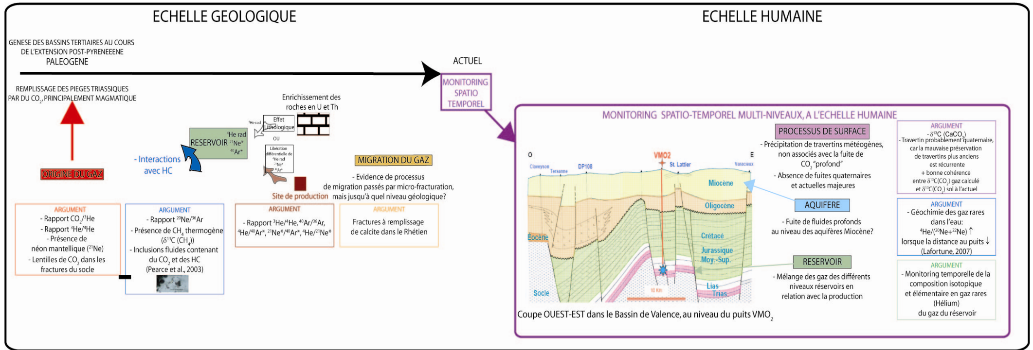
Figure 3.45: Histoire géologique et géochimique du gisement de CO 2 de Montmiral. Coupe: document BRGM.
