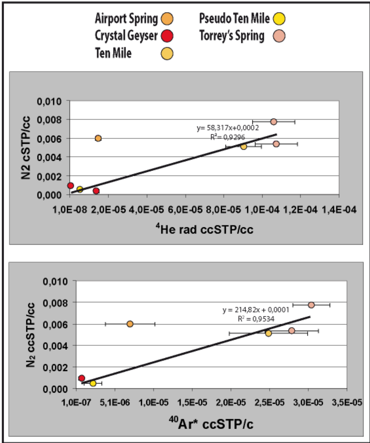
Figure 3.82: N 2 versus 4 He et N 2 versus 40 Ar* (en ccSTP/cc) pour les échantillons de Green River.
