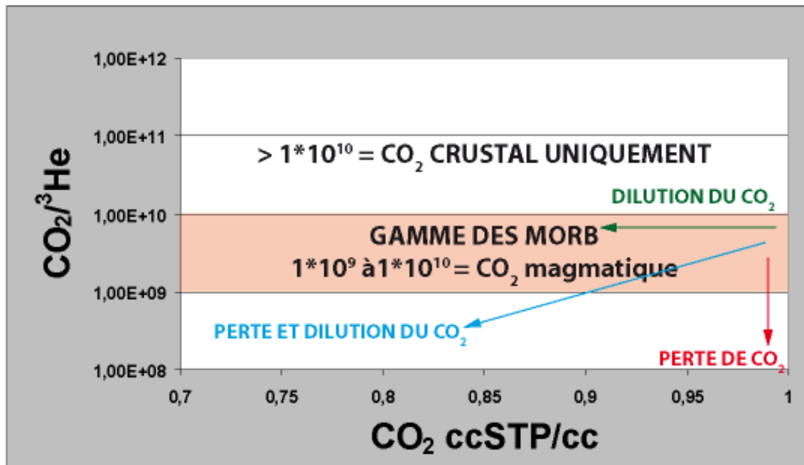
Figure 3.5: Utilisation du diagramme CO_2/{}^3He pour identifier l'origine du CO_2 (modifié, d'après Ballentine et al., 2002a).
