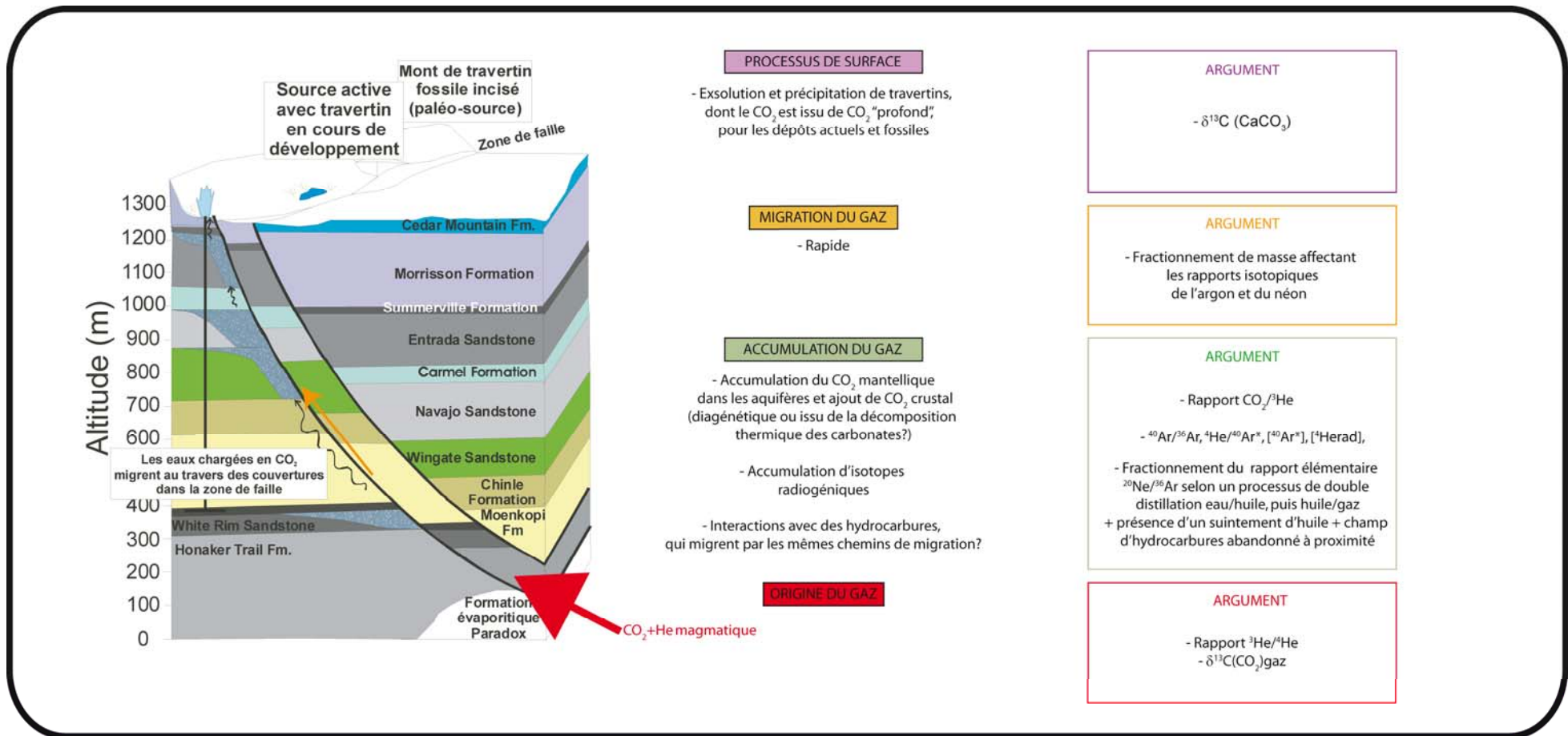
Figure 3.88: Histoire géologique et géochimique des sources carbo-gazeuses et des geysers de Green River.
