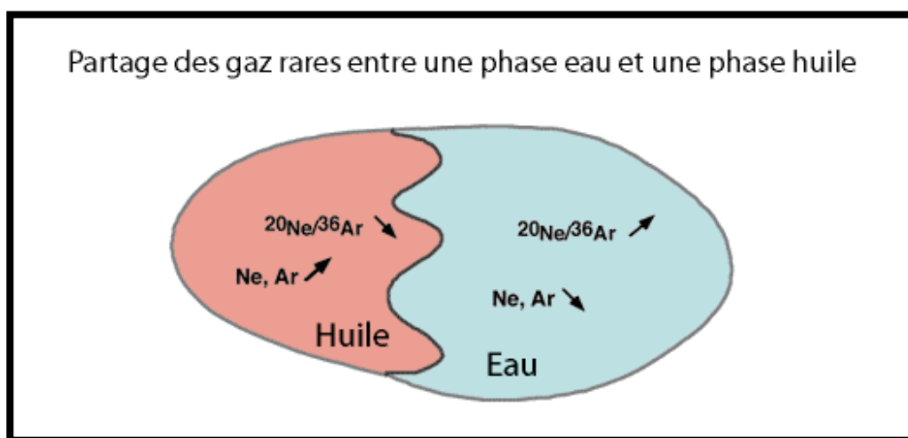
Figure 3.41: Représentation schématisée du partage des gaz rares entre une phase eau et une phase huile en fonction des solubilités respectives des gaz rares dans l'eau.
