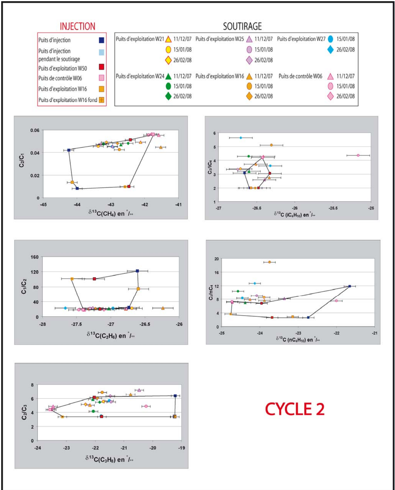
Figure 4.22: Diagrammes de mélange C_2/C_1 versus \delta^{13}C ( CH_4 ), C_1/C_2 versus \delta^{13}C ( C_2H_6 ), C_2/C_3 versus \delta^{13}C ( C_3H_8 ), C_3/iC_4 versus \delta^{13}C ( iC_4H_{10} ) et C_3/nC_4 versus \delta^{13}C ( nC_4H_{10} ) représentant les gaz injectés et soutirés au cours du cycle 2.
