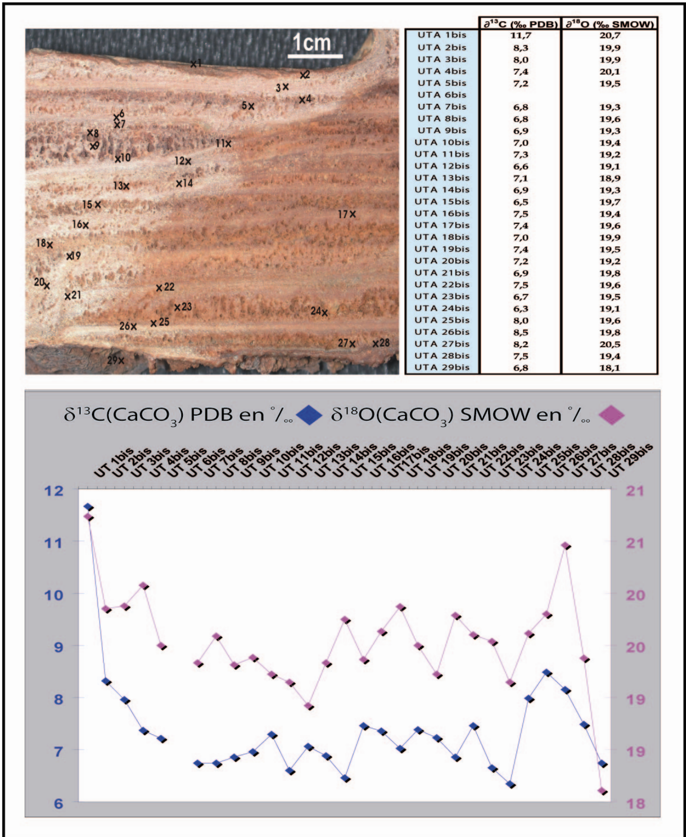
Figure 3.55: Composition isotopique en carbone et en oxygène du travertin actif de Crystal Geysir.
