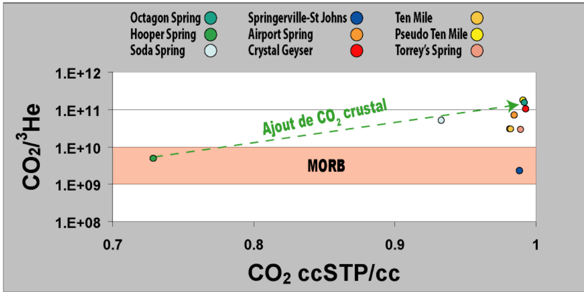
Figure 3.67: Diagramme CO_2/{}^3He versus CO_2 pour les échantillons des Etats-Unis.
