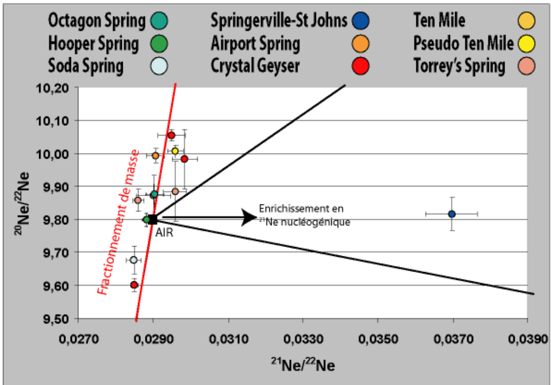
Figure 3.73: Diagrammes ^{40}\text{Ar}/^{36}\text{Ar} versus ^{38}\text{Ar}/^{36}\text{Ar} et ^{20}\text{Ne}/^{22}\text{Ne} versus ^{21}\text{Ne}/^{22}\text{Ne} (Échantillons de Soda Spring et de Green River). L'échantillon de Springerville-St Johns a été représenté sur le diagramme ^{20}\text{Ne}/^{22}\text{Ne} versus ^{21}\text{Ne}/^{22}\text{Ne} pour montrer l'enrichissement en isotopes nucléogéniques.
