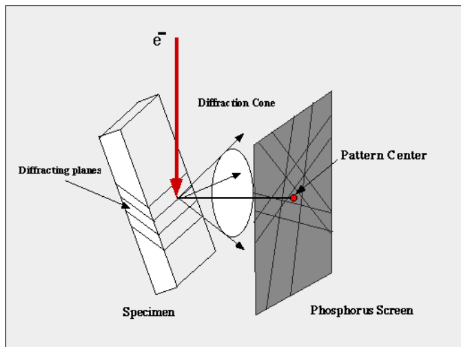
Figure II.26 : Représentation schématique du principe de la méthode EBSP/EBSD.
