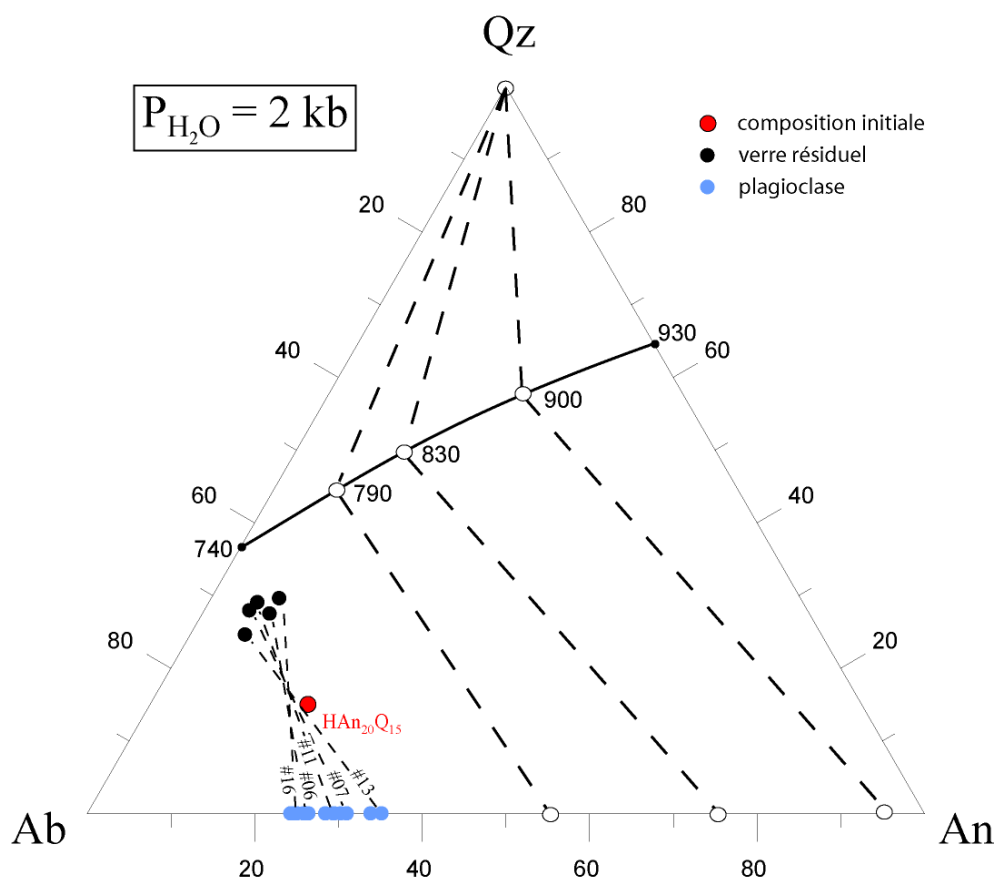
Figure III.26 : Compositions chimiques des verres résiduels et des plagioclases reportées dans un diagramme ternaire Qz-Ab-An. La courbe cotectique (en noir) et les compositions des phases coexistantes sont indiquées pour \text{PH}_2\text{O} = 2 \text{ kbar} (Johannes et Holtz, 1996). Les lignes pointillées relient les phases coexistantes (indiquées par les cercles) pour des températures de 790°, 830 et 900°C. Les points noirs représentent les points eutectiques pour le système binaire Qz-An et Qz-Ab. La composition de départ HAn 20 Q 15 est indiquée par un rond rouge. Les compositions des verres sont indiquées par des ronds noirs. Les compositions des plagioclases sont indiquées en bleu. Verres et plagioclases synthétiques obtenues pour chaque composition sont reliés par des lignes de conjugaison.
