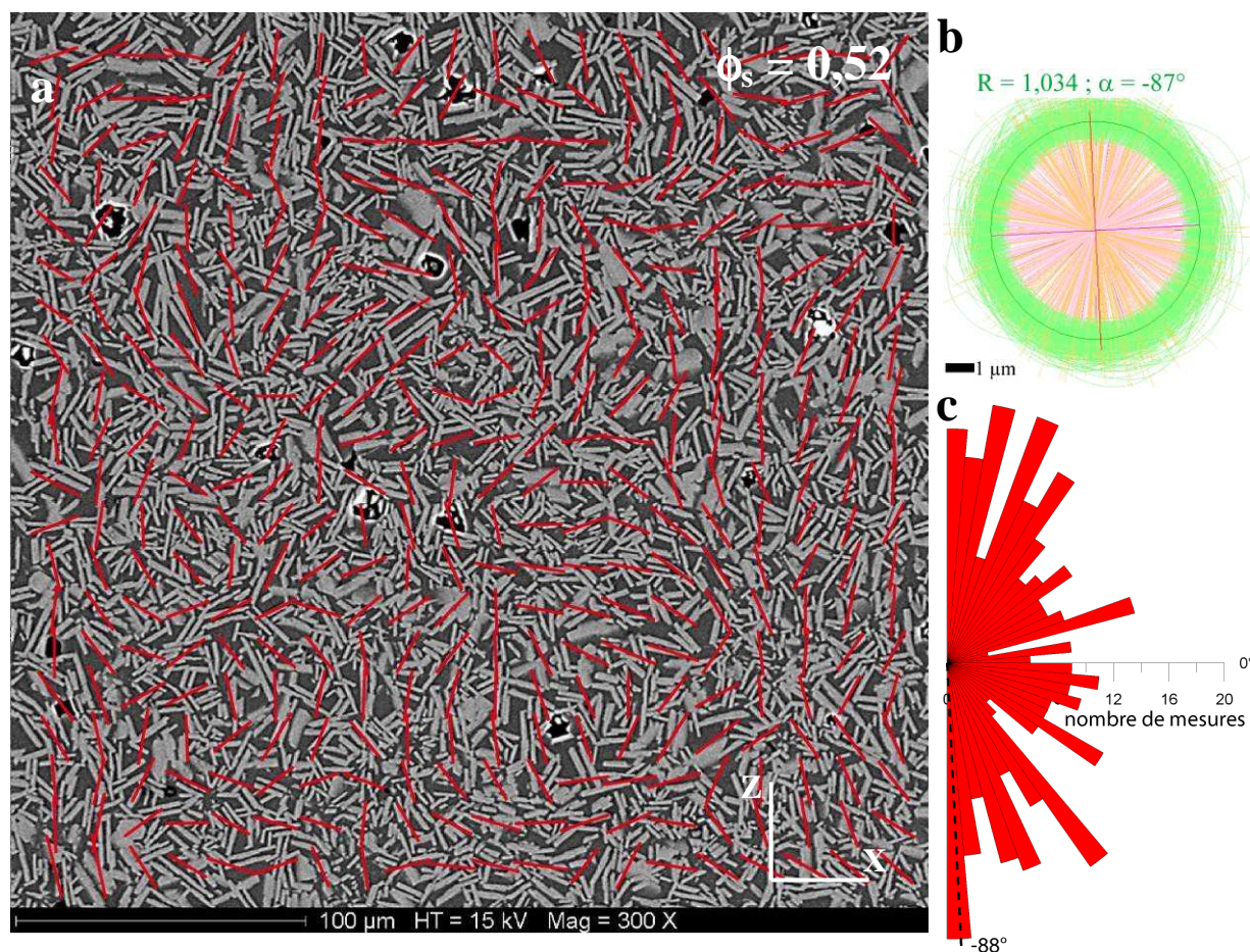
Figure III.14 : Détermination des textures pour des suspensions non déformée contenant \phi_s = 0,52 . (a) Image MEB en électrons rétrodiffusés. Les traits rouges représentent les axes longs des ellipses locales de fabrication de forme. (b) Ellipses tensorielles locales de fabrication de forme. Les valeurs des excentricités des ellipses moyennes ( R ) ainsi que leurs directions d'orientation ( \alpha ) sont indiquées au dessus de l'ellipse. (c.) Rose des directions des axes longs des ellipses locales de fabrication de forme. La direction d'orientation maximale est indiquée en noir.
