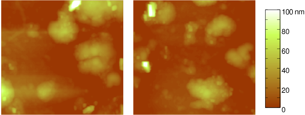
FIG. 3.16 – Deux images AFM représentatives de la surface des grains. Chaque image correspond à une fraction de 5 \mu\text{m} de côté de la surface d'un grain. L'échelle du relief est indiquée à droite, en nanomètres. La rugosité de surface des grains se situe typiquement entre 50 et 100 nm. Ces images ont été réalisées par Cendrine Moskalenko (Laboratoire de Physique, ENS Lyon).
