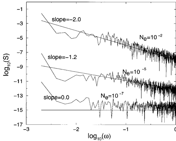
FIG. 2.8 – Spectre de puissance de la contrainte exercée par une couche de grains 2D, cisailée à vitesse imposée et libre de se dilater. Les trois spectres de puissance correspondent à trois pressions de confinement N_e , différentes. Dans les trois cas, le spectre suit une loi de puissance dont l'exposant augmente avec la pression de confinement, confirmant l'idée suivant laquelle sa valeur est liée à la liberté laissée aux grains. Le coefficient de friction inter-grains est ici fixé à \mu = 0.5 . Extrait de (Aharonov & Sparks, 1999).
