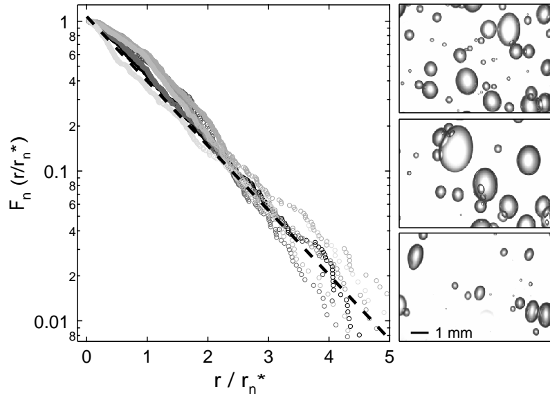
FIG. 6.3 – Bulles piégées dans le colonne. (Gauche) : estimation de la probabilité cumulée F_n des bulles de taille r dans la couche n (les tons de gris sont uniformément répartis : du gris clair pour la tranche la plus basse de la colonne, au noir pour la tranche la plus haute). La distribution F_n est une exponentielle (ajustement linéaire en trait pointillé) de taille caractéristique r_n^* ; l'évolution de r_n^* avec l'altitude z est rapportée sur la figure 6.4 : on en retient que r_n^* est constant sur la hauteur de la colonne avec r_n^* = (0.58 \pm 0.04) mm. (Droite) : les photos de bas en haut correspondent respectivement aux couches d'altitude z \in [0.5; 2.5] cm, z \in [8.5; 10.5] cm et z \in [12.5; 14.5] cm.
