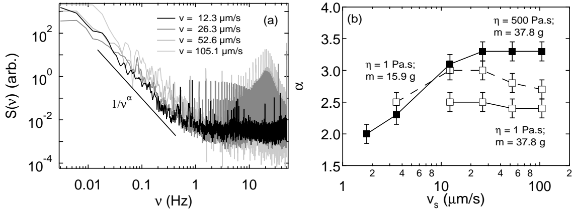
FIG. 4.12 – (a) Spectre de puissance des fluctuations d'altitude |\delta z_f|^2 du patin en fonction de la fréquence \nu . Contrairement aux spectres de puissance des fluctuations de force, les spectres de puissance des fluctuations d'altitude ne se renormalisent pas en considérant la fréquence spatiale \nu/v_s . [ k = 180 \text{ N}\cdot\text{m}^{-1} , d = 451 \text{ }\mu\text{m} , m = 37.8 \text{ g} , \eta = 1 \text{ Pa}\cdot\text{s} ]. (b) Exposant \alpha de la loi de puissance en fonction de la vitesse du patin v_s . Les symboles ouverts (resp. pleins) correspondent à un liquide interstitiel de viscosité \eta = 1 \text{ mPa}\cdot\text{s} (resp. \eta = 500 \text{ mPa}\cdot\text{s} ). Les traits noirs pointillés (resp. continus) correspondent à un patin de masse m = 15.9 \text{ g} (resp. m = 37.8 \text{ g} ).
