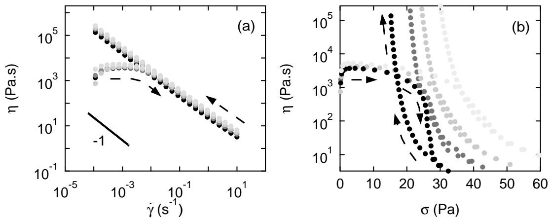
FIG. 6.5 – (a) Viscosité \eta fonction du taux de cisaillement \dot{\gamma} . Les solutions de gel contenant des bulles piégées sont fortement rhéofluidifiantes et présentent une viscosité qui décroît en loi de puissance lorsque le taux de cisaillement augmente suivant : \eta \propto \dot{\gamma}^{-\beta} , avec \beta = 0.95 . L'exposant est plus important que celui mesuré pour une solution sans bulles et sa valeur, très proche de 1, peut s'interpréter par la déformation et la réorganisation des bulles sous l'effet du cisaillement, plutôt que par un éventuel glissement du fluide à la paroi du plan ou encore d'une bande de cisaillement [Manneville (2008)]. (b) Viscosité \eta fonction de la contrainte \sigma . Au sein de la colonne, le seuil du fluide décroît avec l'altitude ; il passe de \sigma_c \simeq 35 Pa à \sigma_c \simeq 20 Pa. De plus, la présence de bulles conduit à une augmentation significative des effets mémoire (thixotropie). En témoigne la divergence de la viscosité mesurée sur la branche retour, à taux de cisaillement imposé (voir texte). Les symboles, du gris clair au noir, correspondent respectivement à z \in [0.5; 2.5] cm, z \in [3.5; 5.5] cm, z \in [8.5; 10.5] cm et z \in [12.5; 14.5] cm. (Fraction massique d'eau ajoutée : 10 %, entrefer e = 1000 \mu m, \Delta t = 15 s, mesures réalisées pour des valeurs croissantes - puis décroissantes - du taux de cisaillement imposé).
