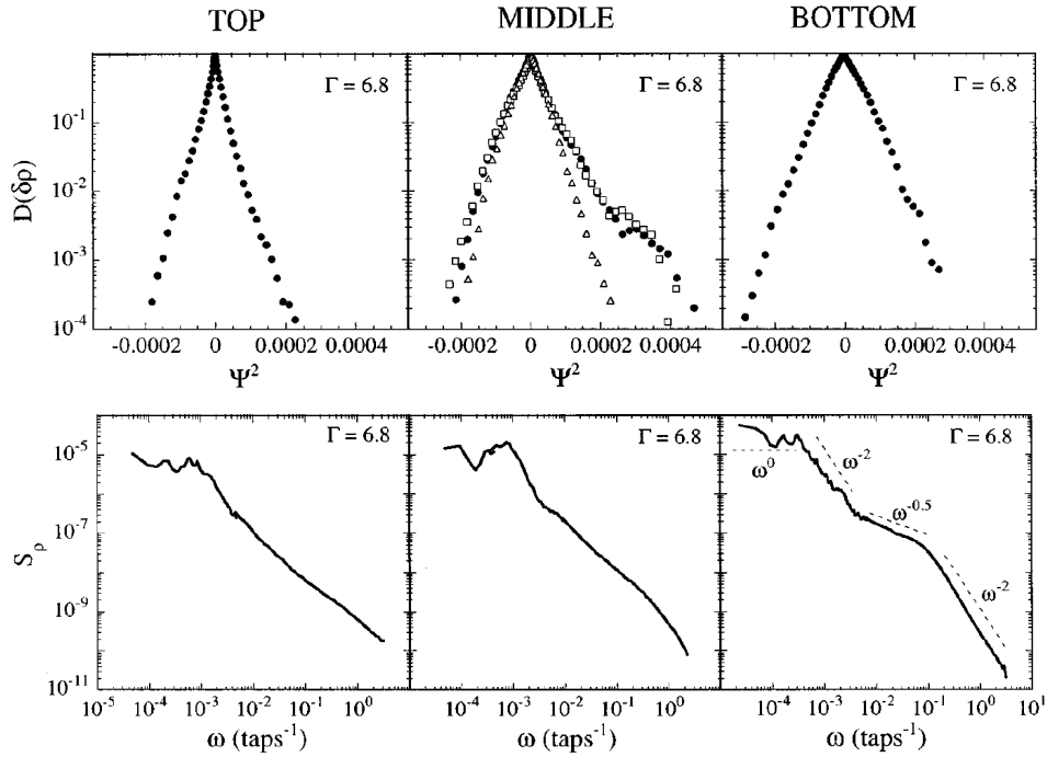
FIG. 2.4 – (Haut) : Distribution de probabilité D(\delta\rho) des fluctuations de compacité \delta\rho d'un empilement de grains soumis à des secousses régulières. Par définition \Psi^2 = \delta\rho^2 \times \text{sgn}(\delta\rho) de telle façon qu'une gaussienne présente une forme triangulaire dans cette représentation. Les fluctuations sont gaussiennes aux différentes hauteurs de la colonne. Ce résultat vaut pour différentes valeurs de \Gamma . (Bas) : Spectre en énergie S_p(\omega) des fluctuations de compacité de la colonne. Ces fluctuations présentent en général trois régimes : (i) un régime de bruit blanc, S_p(\omega) \propto \omega^0 pour \omega < \omega_L , (ii) un régime intermédiaire au sein duquel S_p suit une ou plusieurs lois de puissance d'exposants non triviaux, pour \omega_L < \omega < \omega_H ; (iii) un régime de coupure pour lequel S_p(\omega) \propto \omega^{-2} ("Top", "Middle" et "Bottom", se rapportent à trois altitudes différentes dans la colonne de grains). Extrait de (Nowak et al., 1998).
