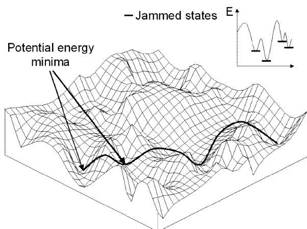
FIG. 2.2 – Représentation schématique du paysage énergétique qui domine la dynamique d'un système vitreux, et en particulier d'un tas de sable, en-deçà de la transition de blocage. Un empilement de grains correspond à un minimum local du paysage énergétique, et provoquer une réorganisation en injectant de l'énergie dans le tas, par le biais d'une secousse, d'un cisaillement, etc. permet d'atteindre un autre minimum local du paysage. Extrait de (Makse et al., 2004a).
