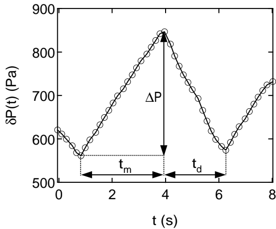
FIG. 6.8 – Évolution du signal de pression sur la durée d'émission d'une bulle. Alimentée en gaz au débit Q , la chambre voit sa surpression \delta P croître sur un temps t_m pour atteindre le seuil de nucléation \Delta P d'une bulle. L'émission d'une bulle entraîne une chute de la pression sur un temps t_d . Le seuil d'émission d'une bulle \Delta P et donc de façon concomitante t_m et t_d , varie d'une bulle à l'autre suivant la valeur de la contrainte seuil du fluide (voir texte).
