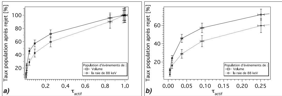
FIGURE 9.10 – Taux d'événements de volume ( E_{\text{recul}} \in [130; 200] \text{ keV} ) et de la raie de 88 keV rejetés en fonction du taux d'ESCRN après rejet actif \tau_{\text{actif}} .
