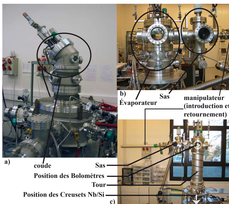
FIGURE 10.3 – Photos des nouveaux dispositifs d'évaporation. a ) et c ) évaporateur dédié au niobium-silicium. b ) évaporateur multi-creusets. Les éléments comme la tour et le sas ont été conçus afin de pouvoir s'adapter sur les deux évaporateurs.
