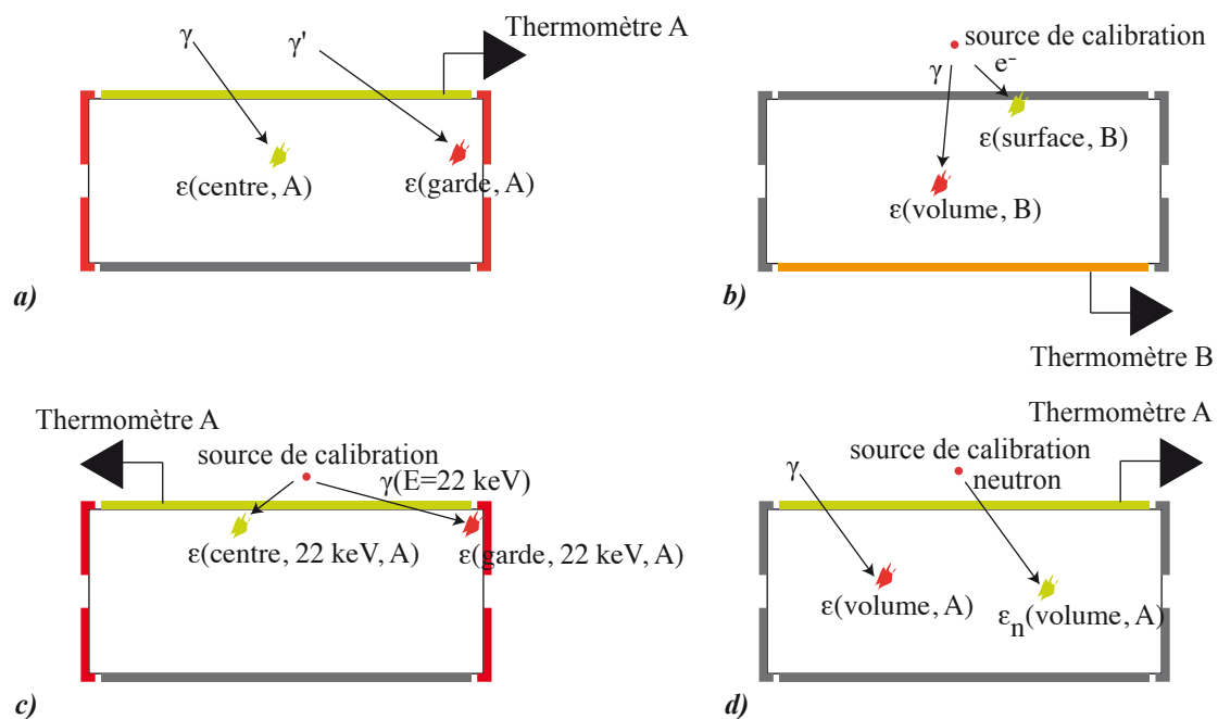
FIGURE 13.11 – Schéma en coupe d'un détecteur. Les populations d'événements sont sélectionnées par différents critère (énergie, profondeur de pénétration, nature de la particule, position de l'interaction,...). Les équations (13.14), (13.15), (13.16), (13.17) correspondent, respectivement, au populations schématisées sur les figures a ), b ), c ) et d ). L'amplificateur représente le film utilisé pour la détermination des amplitudes athermique et thermique.
