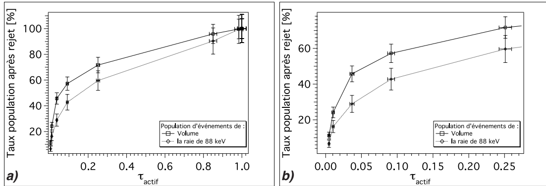
FIGURE 9.10 – Taux d'événements de volume ( E_{\text{recul}} \in [130; 200] \text{ keV} ) et de la raie de 88 keV rejetés en fonction du taux d'ESCRN après rejet actif \tau_{\text{actif}} .
