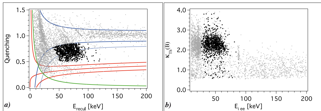
FIGURE 12.8 – a) Q -plot et b) rapport \kappa_{Th} du thermomètre exposé à la source de calibration de ^{109}Cd , en fonction de l'énergie ionisation du Bolo Ge/NbSi 213. Mise en évidence de la population de surface redéfinie.
