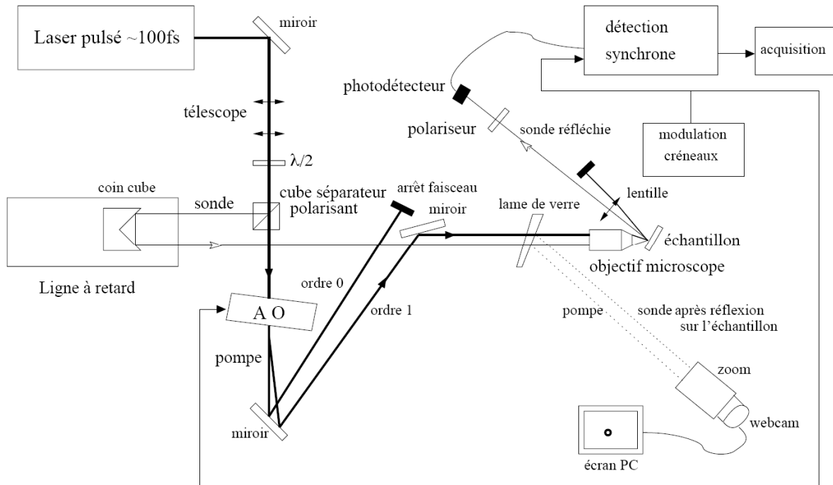
Figure 2 - 18 : Montage réfectométrique en incidence pompe sonde oblique.
