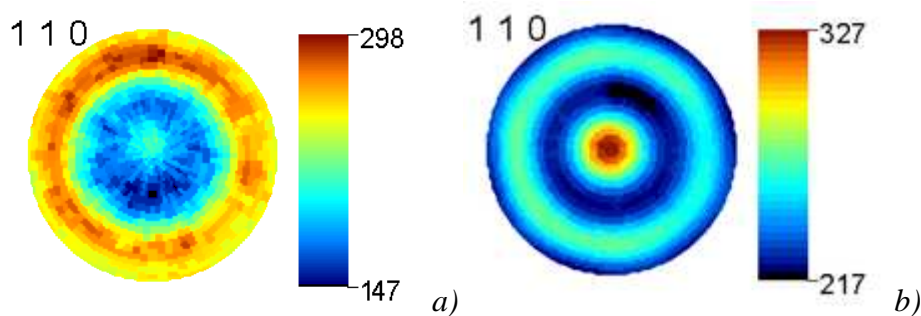
Figure 4 - 12: Figure de pôles expérimentale a) magnétique totale, I_{\{110\}}^m(\vec{y}, \vec{B}) et b) magnétique, I_{\{110\}}^m(\vec{y}, 0) .
