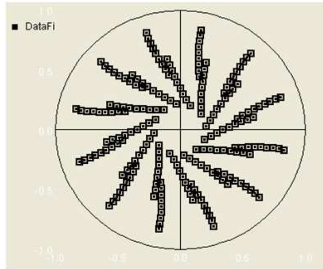
Figure 3 - 25 : Couverture des figures de pôle pour \chi_{plate} = 30^\circ et 55^\circ , un \phi sur 12.
