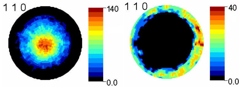
Figure 4 - 11 : Figures de pôles (110) de polarisation magnétique, négative \Delta I_{\{110\}}^{p-}(\vec{y}, \vec{B}) (Gauche) et positive \Delta I_{\{110\}}^{p+}(\vec{y}, \vec{B}) (droite). L'échelle indiquée pour la figure de pôles \Delta I_{\{110\}}^{p-}(\vec{y}, \vec{B}) est négative.
