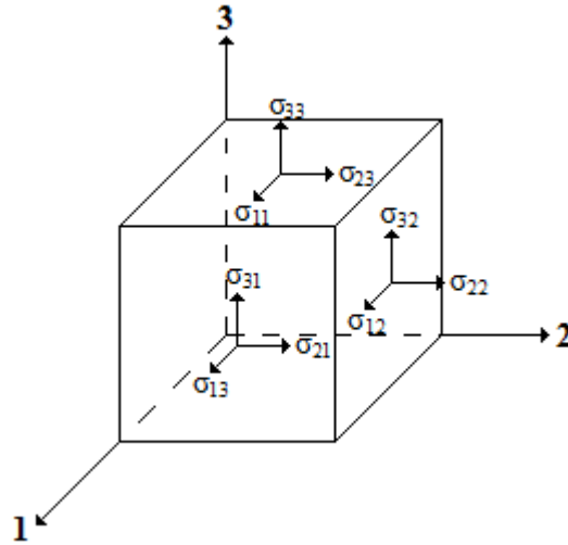
Figure 2 - 2 : Définition des contraintes relatives aux trois axes 1, 2 et 3.
