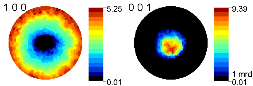
Figure 4 - 25 : Figures de pôles recalculées normalisées {100} et {001}.
