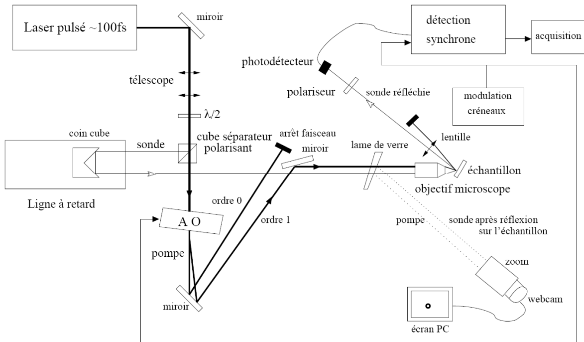
Figure 2 - 18 : Montage réfectométrique en incidence pompe sonde oblique.
