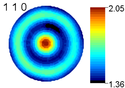
Figure 4 - 6 : Figure de pôles expérimentale, I_{\{110\}}^n(\bar{y}, 0) . Echelle d'intensités divisée par 1 000.
