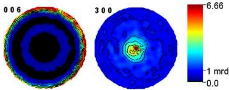
Figure 3 - 19 : Figures de pôles {006} et {300} du rostre de bélemnite du crétacé, mesurées sur D19.
