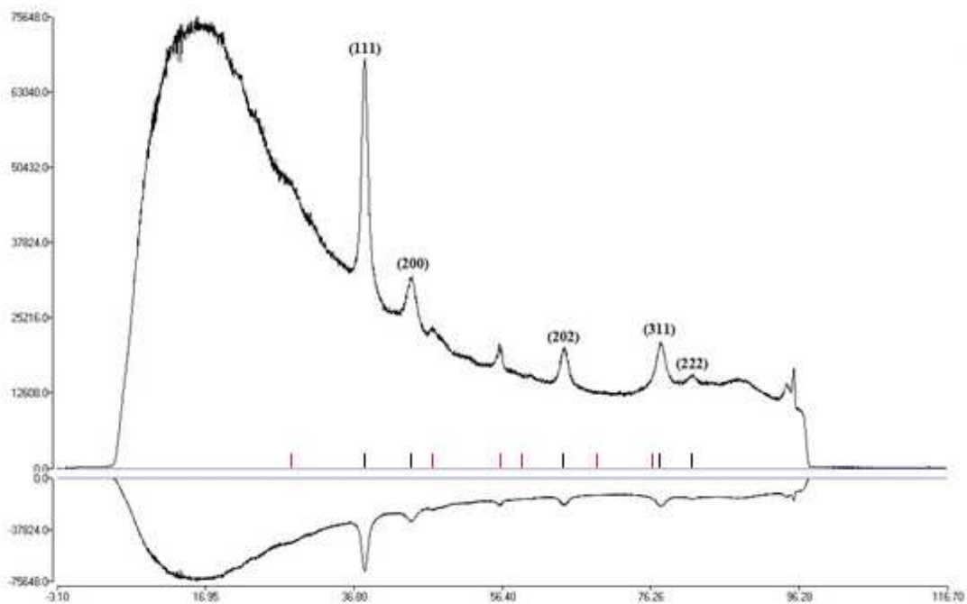
Figure 2 - 3 : Somme de tous les diagrammes de diffraction R-X pour le film d'or de 10 nm d'épaisseur.
