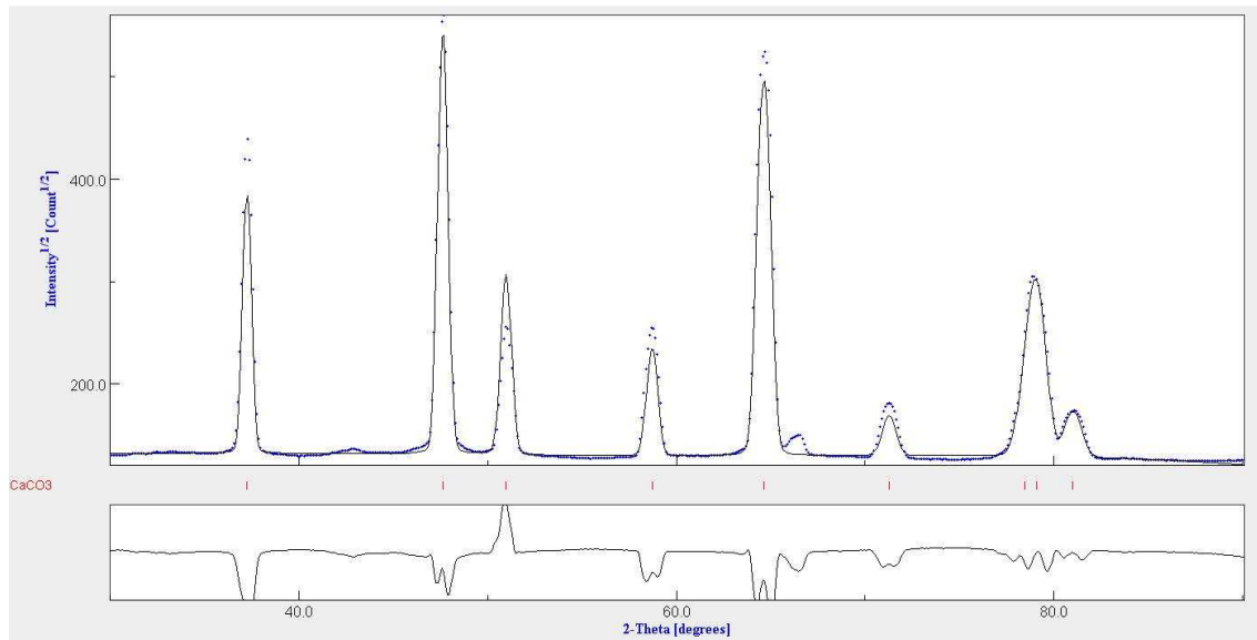
Figure 3 - 16: Somme des 1368 diagrammes mesurés sur un rostre de bélemnite du crétacé ( \lambda=2,42\text{\AA} , D20).
