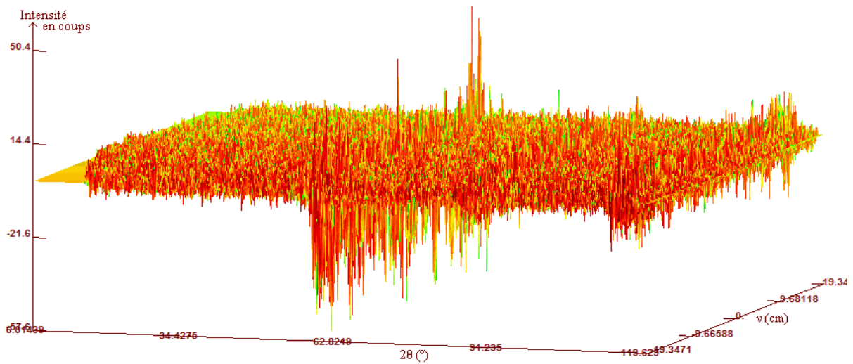
Figure 4 - 4 : Diagramme de Debye-Scherrer différence pour une orientation (\chi_{plate}, \phi) .
