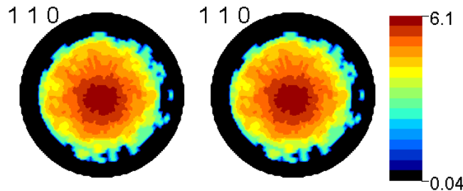
Figure 4 - 26 : Figures de pôles expérimentale et recalculée normalisées, \Delta P_{\{110\}}^{P^-}(\vec{y}, \vec{B}) .
