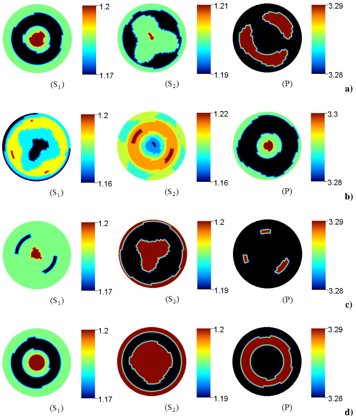
Figure 2 - 8: vitesses transverses et longitudinales pour les échantillons d'or, a) : 10 nm, b) : 15 nm, c) : 35 nm et d) : 40 nm.
