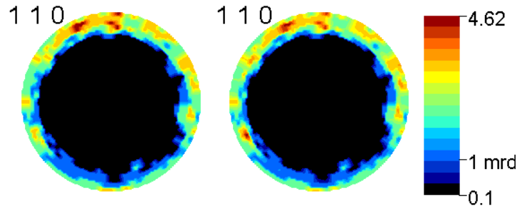
Figure 4 - 24 : Figures de pôles expérimentale et recalculée normalisées, \Delta P_{\{110\}}^{p+}(\vec{y}, \vec{B}) .
