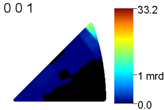
Figure 2 - 12 : figure de pôles inverse, film d'or de 20 nm d'épaisseur.
