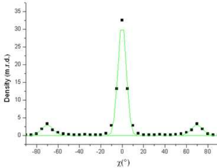
Figure 2 - 13 : Courbe représentant l'orientation préférentielle suivant l'axe \langle 111 \rangle , échantillon 20 nm.
