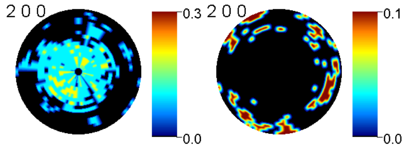
Figure 4 - 14: Figures de pôles de polarisation magnétique, négative \Delta I_{\{200\}}^{p-}(\vec{y}, \vec{B}) et positive \Delta I_{\{200\}}^{p+}(\vec{y}, \vec{B}) (droite). Echelle d'intensité, divisée par 100. L'échelle indiquée pour la figure de pôles \Delta I_{\{200\}}^{p-}(\vec{y}, \vec{B}) est négative.
