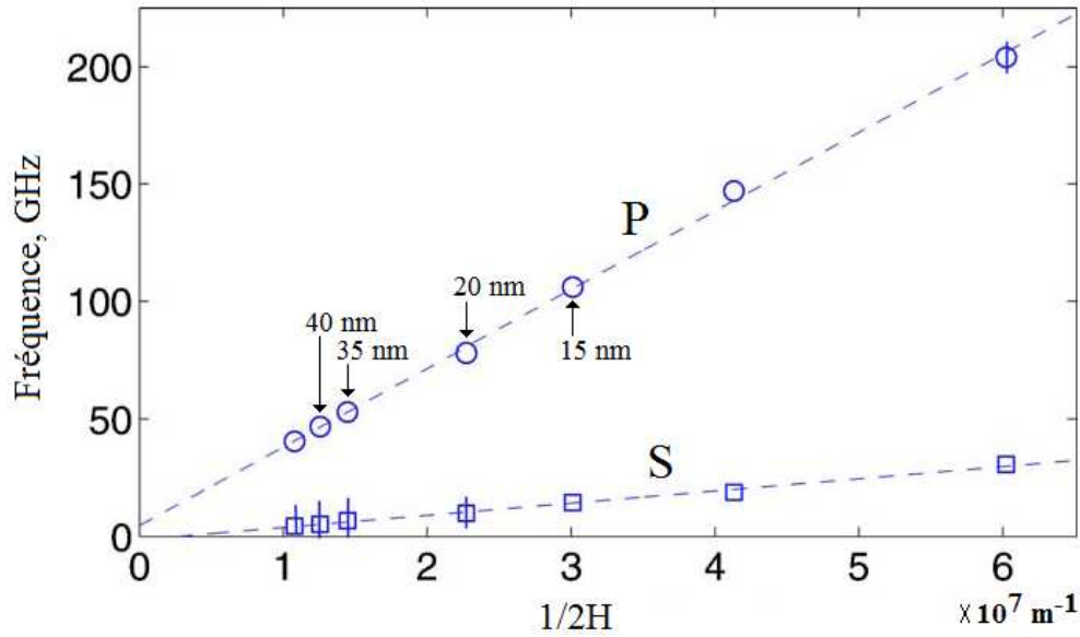
Figure 2 - 21 : Mode transverse (S) et longitudinal (P) en fonction de l'épaisseur des échantillons H. Sur cette figure sont également indiqués 3 films non étudiés en texture, et le film de 10 nm n'a pas été mesuré en réflectivité.
