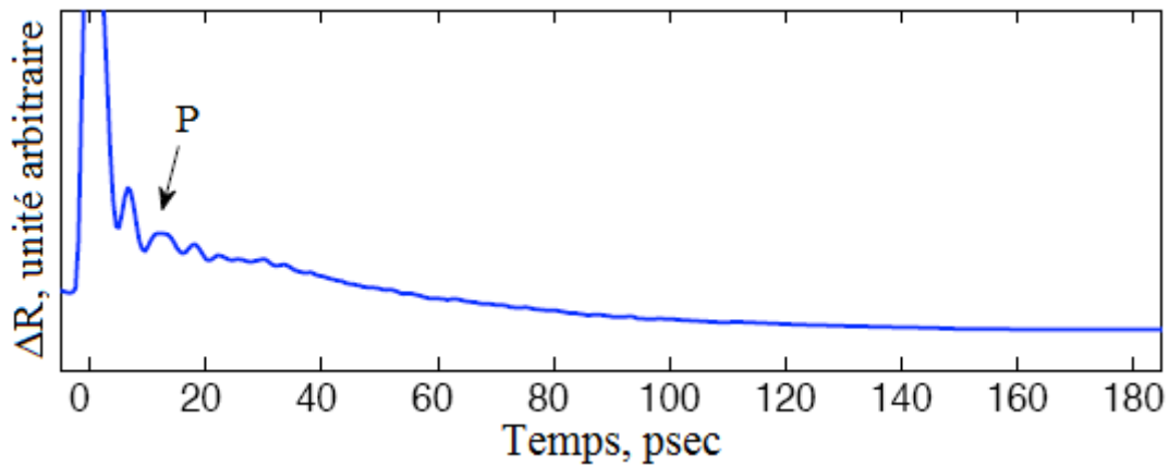
Figure 2 - 20 : Courbe de réflectivité pour la longueur d'onde 400 nm, seule l'onde longitudinale (P) est présente.
