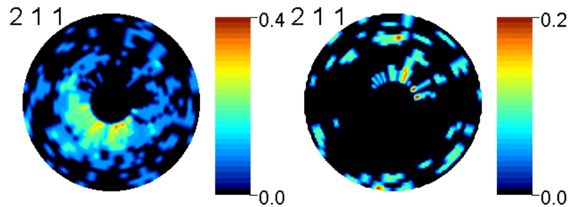
Figure 4 - 17 : Figures de pôles de polarisation magnétique, négative \Delta I_{\{211\}}^p(\vec{y}, \vec{B}) (Gauche) et positive \Delta I_{\{211\}}^{p+}(\vec{y}, \vec{B}) (droite). Echelle d'intensité, divisée par 100. L'échelle indiquée pour la figure de pôles \Delta I_{\{211\}}^p(\vec{y}, \vec{B}) est négative.
