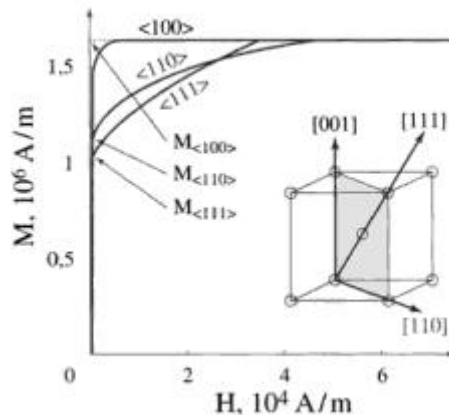
Figure 1 - 1 : Courbe d'aimantation d'un monocristal de fer, lorsque le champ est appliqué selon les trois directions de haute symétrie (Herpin 1968) (Du Trémolet de Lacheisserie 1999).
