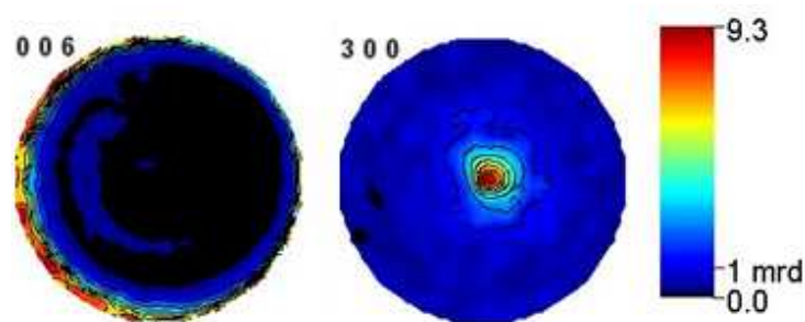
Figure 3 - 17 : Figures de pôles recalculées {006} et {300} du rostre de bélemnite, mesures réalisées sur D20.
