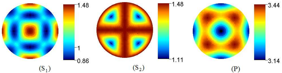
Figure 2 - 7 : Répartition des vitesses de propagations des ondes S 1 , S 2 et P dans le repère de l'échantillon K 5 pour le monocristal d'or.
