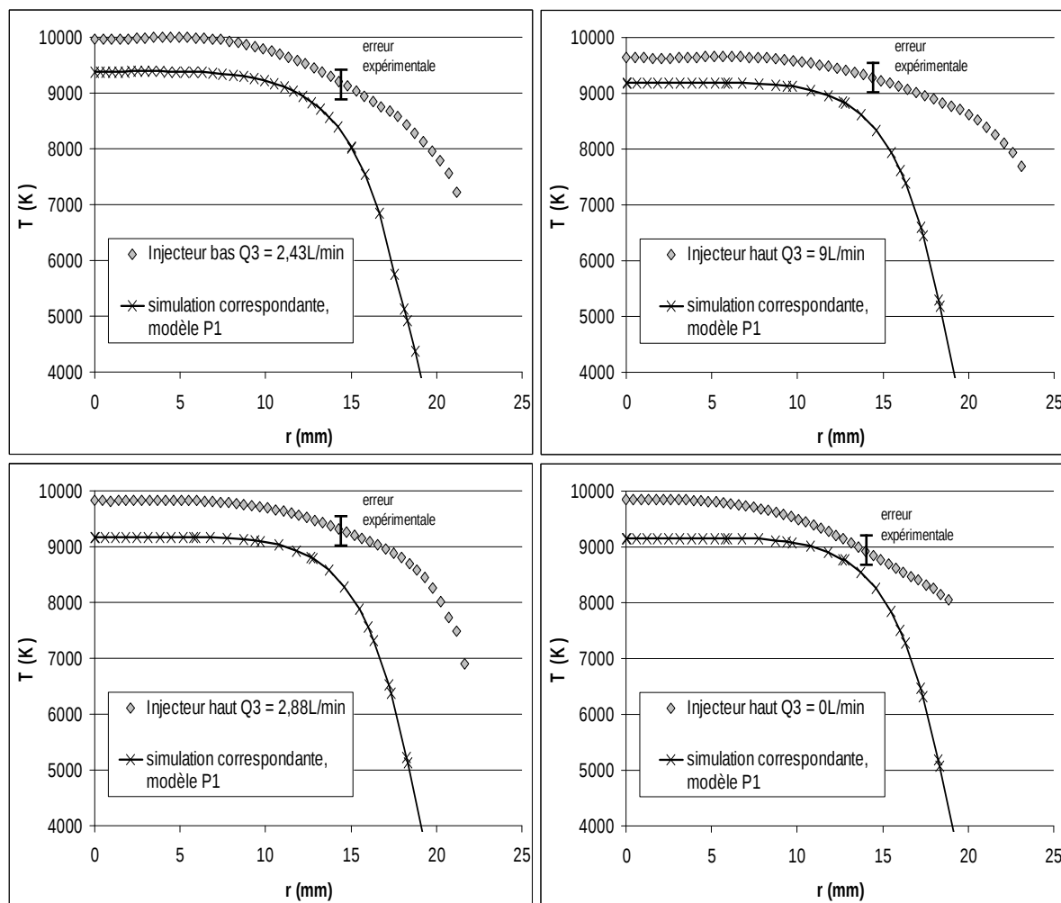
Figure VII-7 : comparaison calcul-expérience pour la torche procédé.
