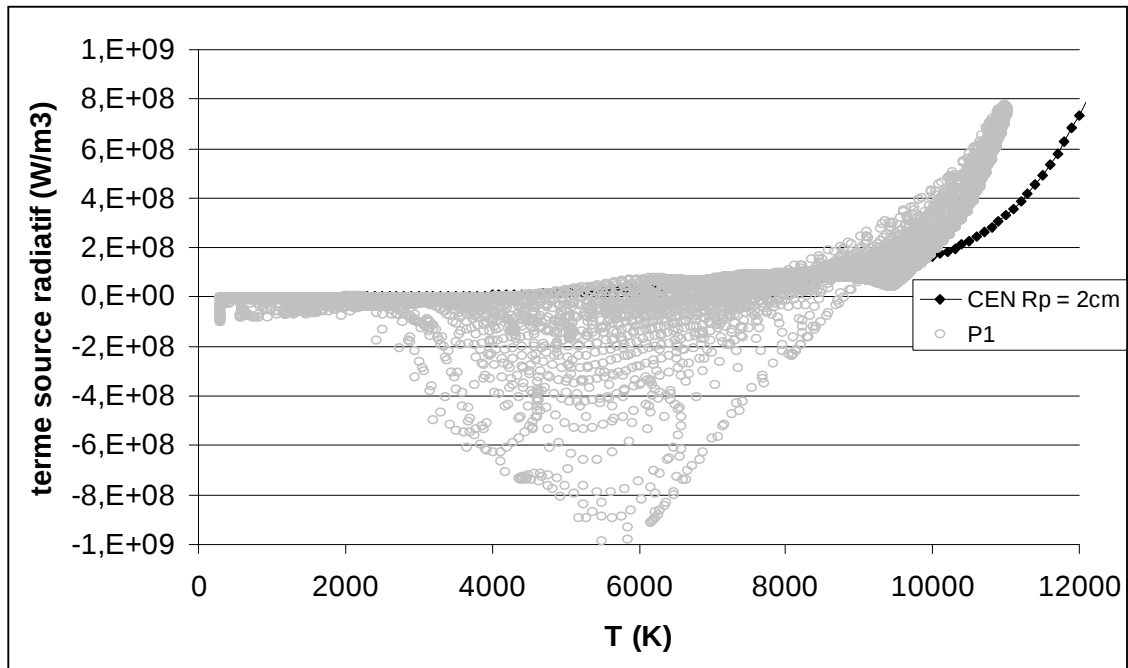
Figure V-25 : termes sources radiatifs correspondant aux deux calculs de la Figure V-24.
