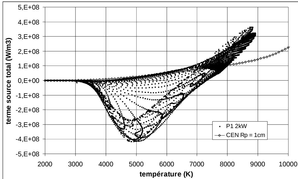
Figure V-14 : termes source radiatif pour un plasma d'analyse en Ar-O 2 avec le CEN (trait plein) et le modèle P1 (marques). P_{\text{ind}} = 2000\text{W} , Q_3 = 0,5\text{L/min} , Q_2 = 0,6\text{L/min} , Q_1 = 15\text{L/min} .
