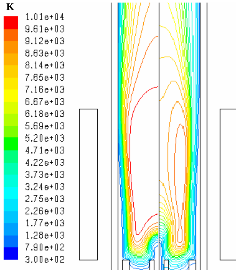
Figure V-11 : température obtenues avec le modèle CEN ( R_p = 1\text{cm} ) en argon pur (gauche) et avec un mélange Ar 95%, O 2 5% molaire (droite). P_{\text{ind}} = 2000\text{W} , Q_3 = 0,5\text{L/min} , Q_2 = 0,6\text{L/min} , Q_1 = 15\text{L/min} .
