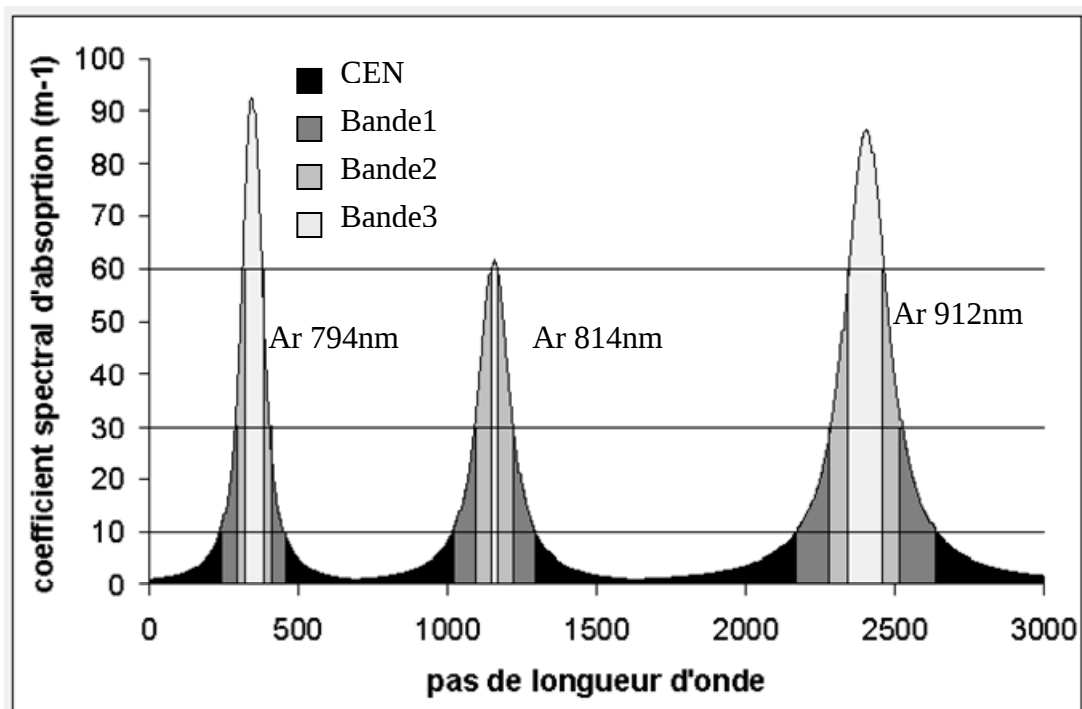
Figure IV-17 : Plages du spectre intégrées dans les différentes bandes du modèle P1 pour le groupe 4.
