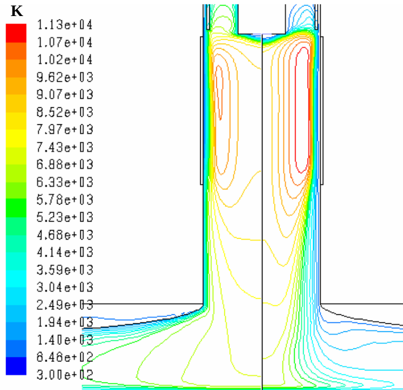
Figure V-24 : champ de température dans une torche procédé en argon-oxygène avec le modèle P1 (gauche) et le modèle CEN ( R_p = 2\text{cm} , droite). P_{\text{ind}} = 20000\text{W} , Q_3 = 2,9\text{L/min} , Q_2 = 3,3\text{L/min} , Q_1 = 94\text{L/min} .
