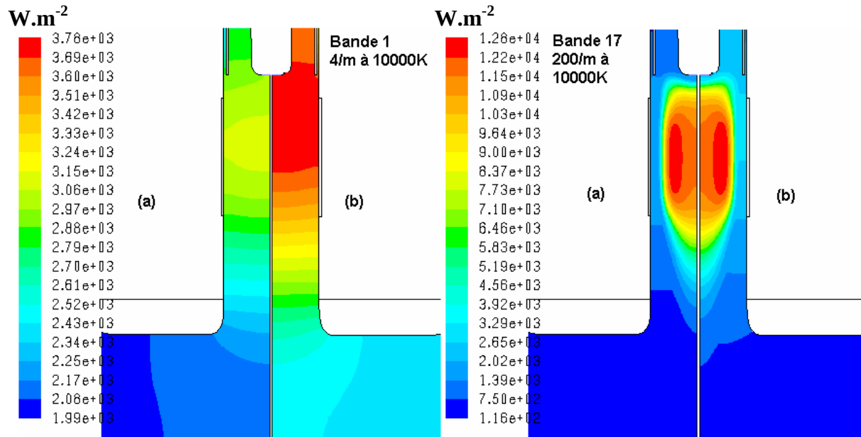
Figure III-11 : comparaison des intensités radiatives en fonction de l'émissivité des parois pour deux bandes du modèle P1 (bande 1 peu absorbée et bande 17 modérément absorbée)
