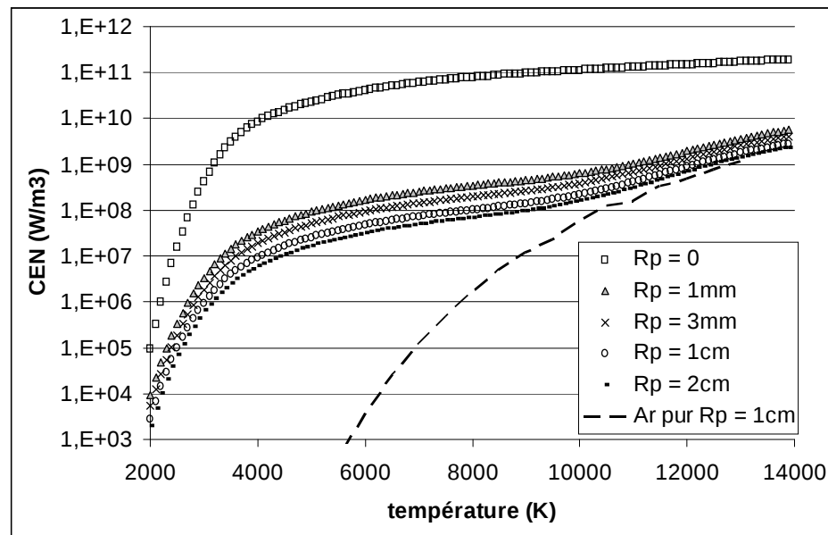
Figure IV-8 : coefficient d'émission net d'un mélange 95%Ar, 5% O 2 en volume en fonction de T et pour différents rayons plasma. Les valeurs obtenues en argon pur sont rappelées pour faciliter la comparaison.
