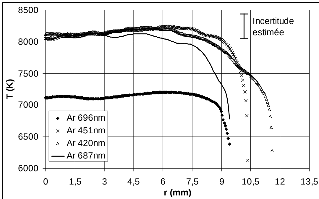
Figure VI-21 : température mesurée en z = 0,5\text{mm} avec 4 raies de l'argon.
