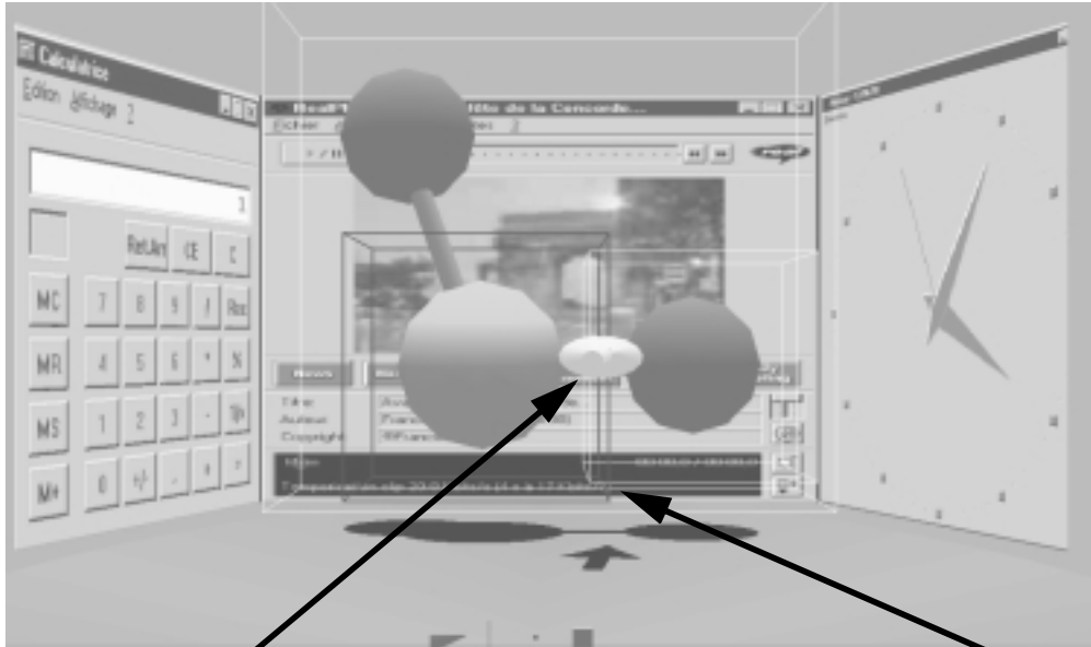
Figure 7.1 le pointeur 3D désigne l'objet sur la table (une molécule d'eau), on voit les boîtes englobantes progressives s'afficher.
