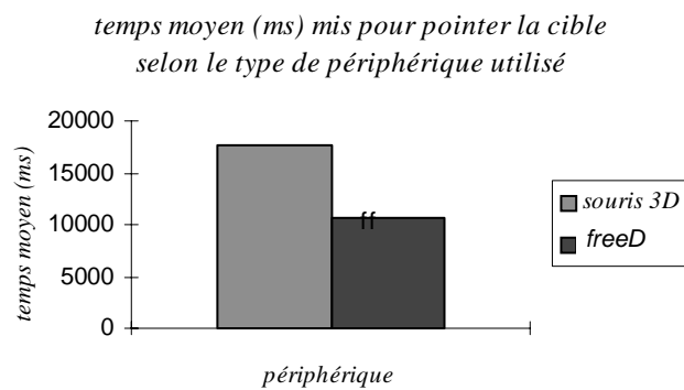
Figure 4.8 temps moyen de pointage / périphérique
