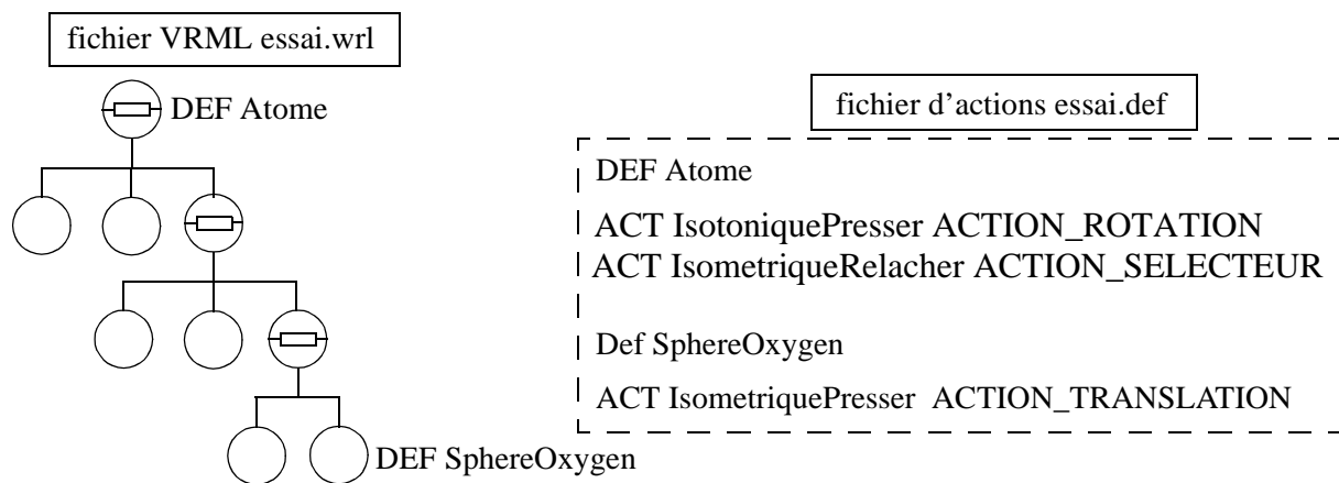
Figure 1.8 un document 3D au format VRML (essai.wrl) et son fichier de comportements associé (essai.def)
