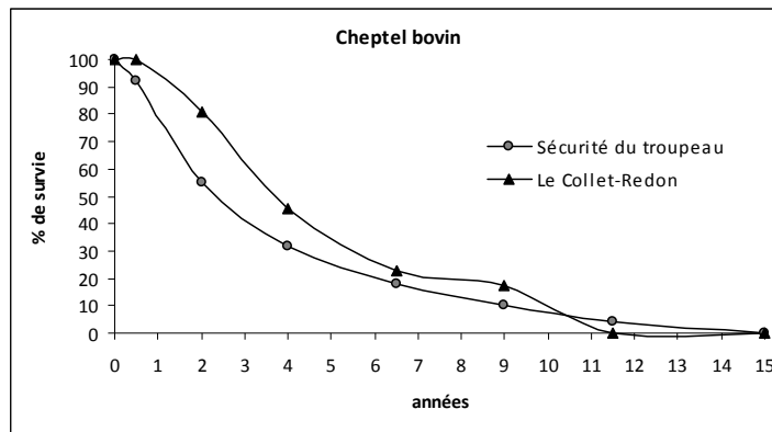
Fig. 79 : Courbe de survie des bœufs du Collet-Redon et modèle théorique pour la sécurité du troupeau
