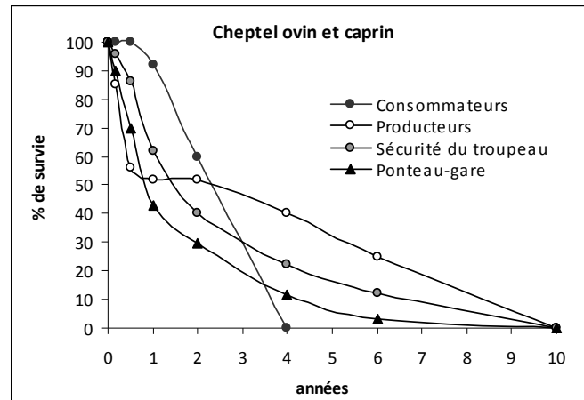
Fig. 111 : Courbes théoriques de survie des groupes consommateurs, producteurs et de la viabilité du troupeau et courbe de survie des caprinés de Ponteau-Gare (NRd)
