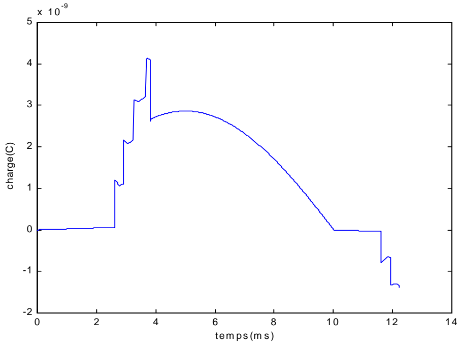
Figure 5.39: Charge en fonction du temps pour le cas d'un isolateur de longueur 50 cm, de rayon 5 cm et de conductivité 50 \mu S (cas de la longueur de fuite variable)
