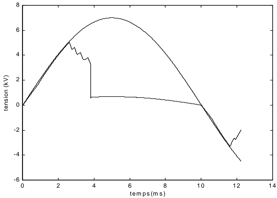
Figure 5.40: Tension appliquée (____), tension à la tête de l'arc (.....) en fonction du temps pour le cas d'un isolateur de longueur 50 cm, de rayon 5 cm et de conductivité 50 \mu S (cas de la longueur de fuite variable)
