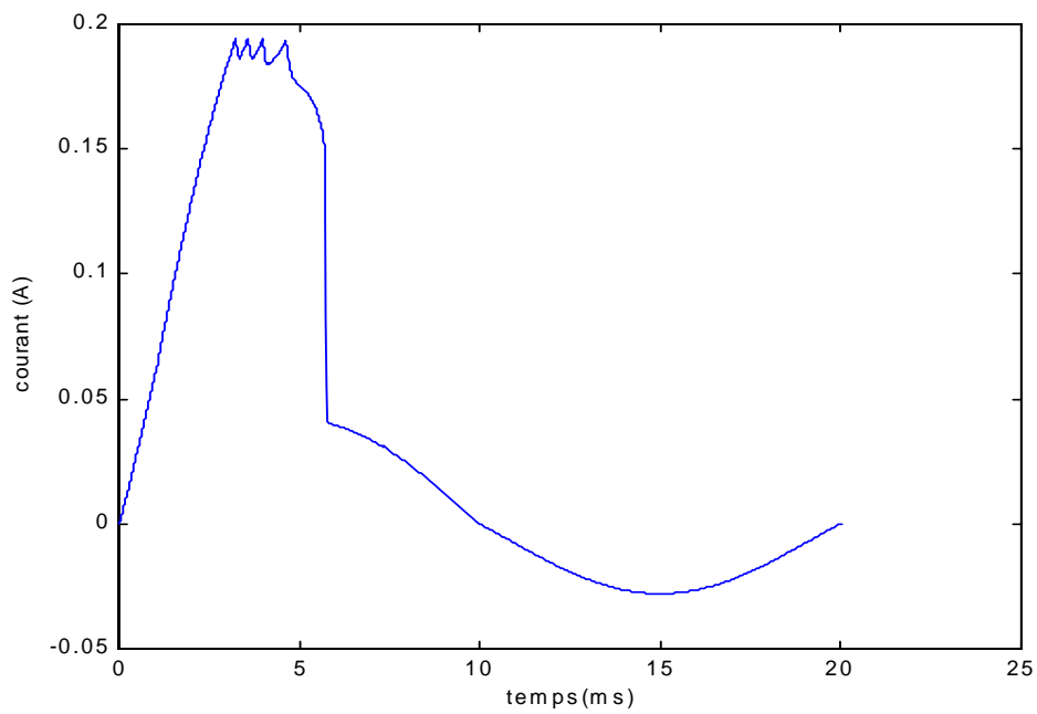
Figure 5.31: Courant de la décharge en fonction du temps pour le cas d'un isolateur de longueur 50 cm, de rayon 5 cm et de conductivité 50 \mu\text{S} (cas de la couche sèche)
