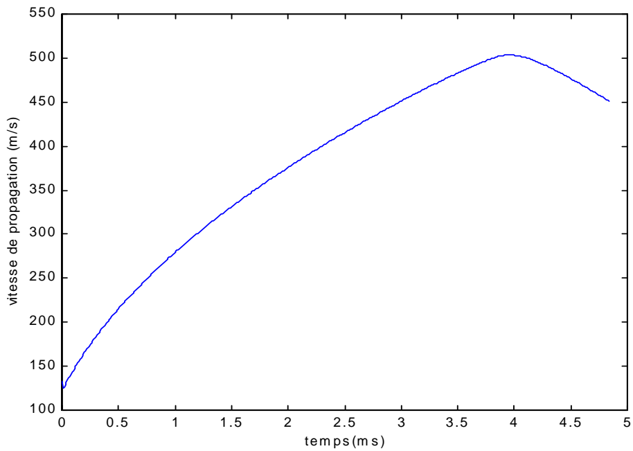
Figure 4.14: Vitesse de propagation de la décharge en fonction du temps pour le cas d'un isolateur de longueur 187 cm, de rayon moyen 15 cm, et de conductivité 50 \mu S
