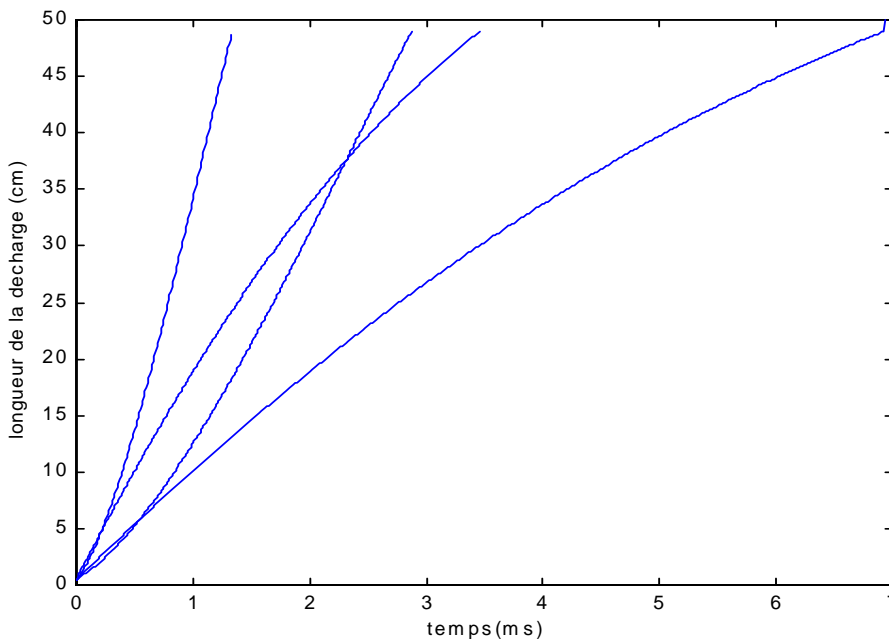
Figure 4.4: longueur de la décharge en fonction du temps pour différentes expressions de la vitesse: (-.-.-): \beta=10\% , (.....): \beta=1\% , (-----): \mu=100 \text{ cm}^2/\text{Vs} , (___): \mu=50 \text{ cm}^2/\text{Vs}
