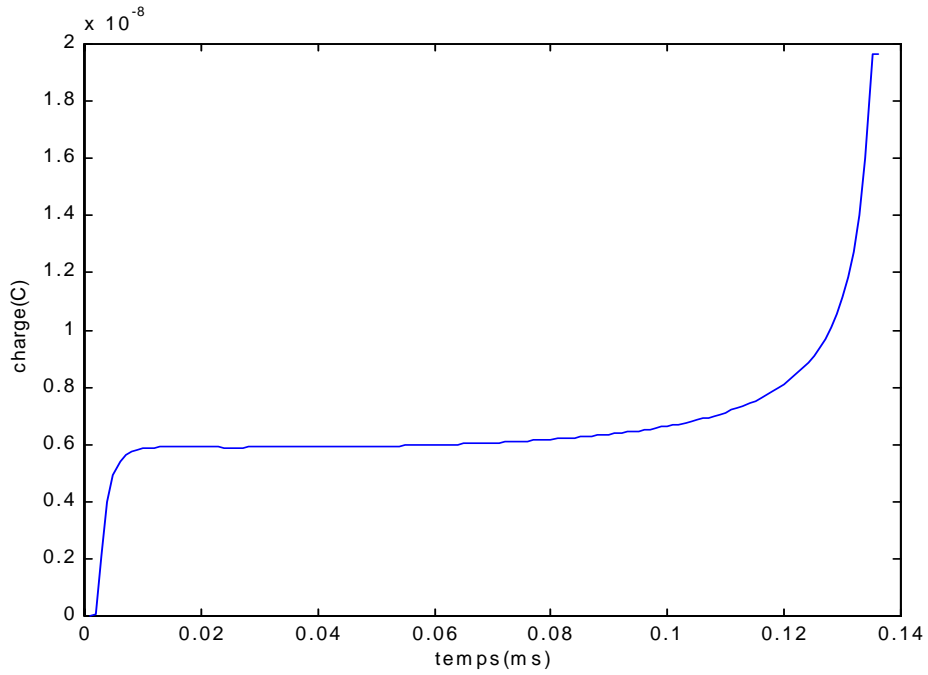
Figure 4.24: Charge à la tête de la décharge en fonction du temps pour le cas d'un isolateur de longueur de fuite 10 cm, de largeur 1 cm, de résistivité 380 Ωcm et une onde de 10/800 μs
