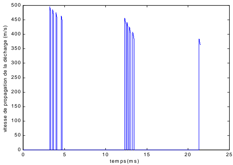
figure 5.48: Vitesse de propagation de la décharge en fonction du temps pour le cas d'un isolateur de longueur 50 cm, de rayon 5 cm et de conductivité 50 \mu S (longueur de la décharge variable)
