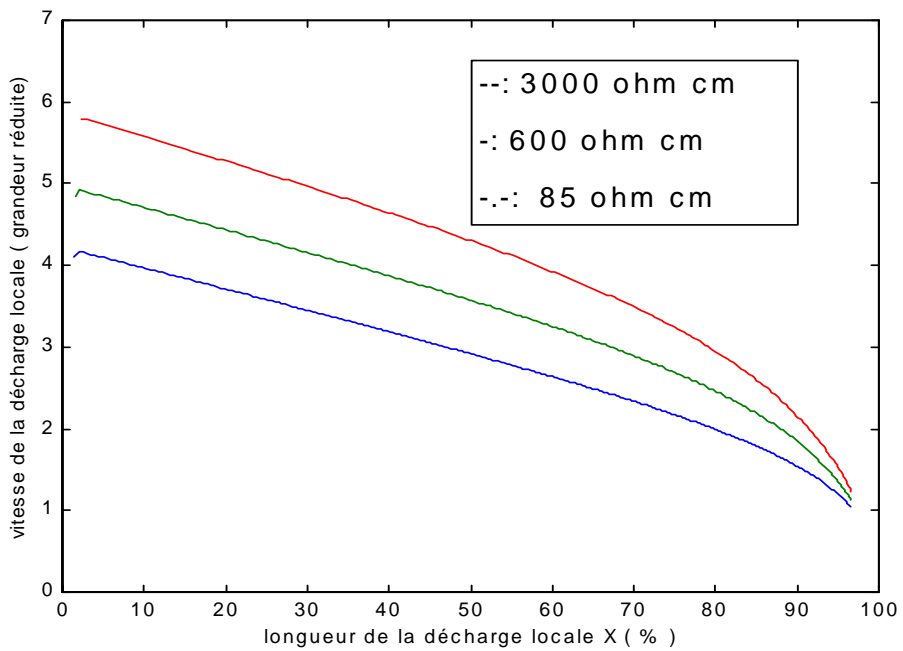
Figure 4.32: vitesse de propagation pour le cas d'un isolateur de longueur de fuite 10 cm, de largeur 1 cm, une onde de 2/80 \mu\text{s} et d'épaisseur de la solution 5 mm, comparée à une vitesse de 120 m/s
