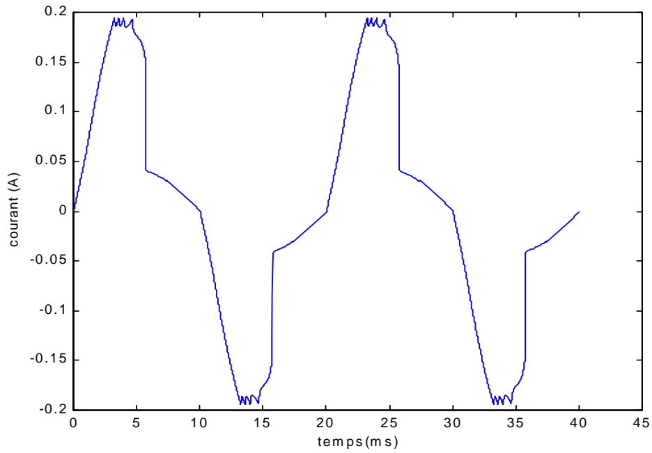
Figure 5.24: Courant de la décharge en fonction du temps pour le cas d'un isolateur de longueur 50 cm, de rayon de 5 cm et de conductivité 50 \mu\text{S} (réamorçage symétrique)
