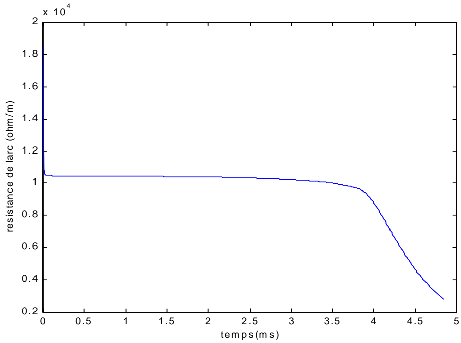
Figure 4.13: Résistance de l'arc en fonction du temps pour le cas d'un isolateur de longueur 187 cm, de rayon moyen 15 cm, et de conductivité 50 \mu S
