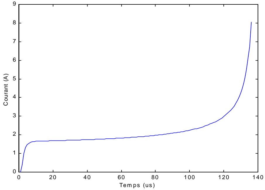
Figure 4.22: Courant de la décharge en fonction du temps calculé par le modèle dynamique pour le cas d'un isolateur de longueur de fuite 10 cm, de largeur 1 cm, de résistivité 380 Ωcm et une onde de 10/800 μs
