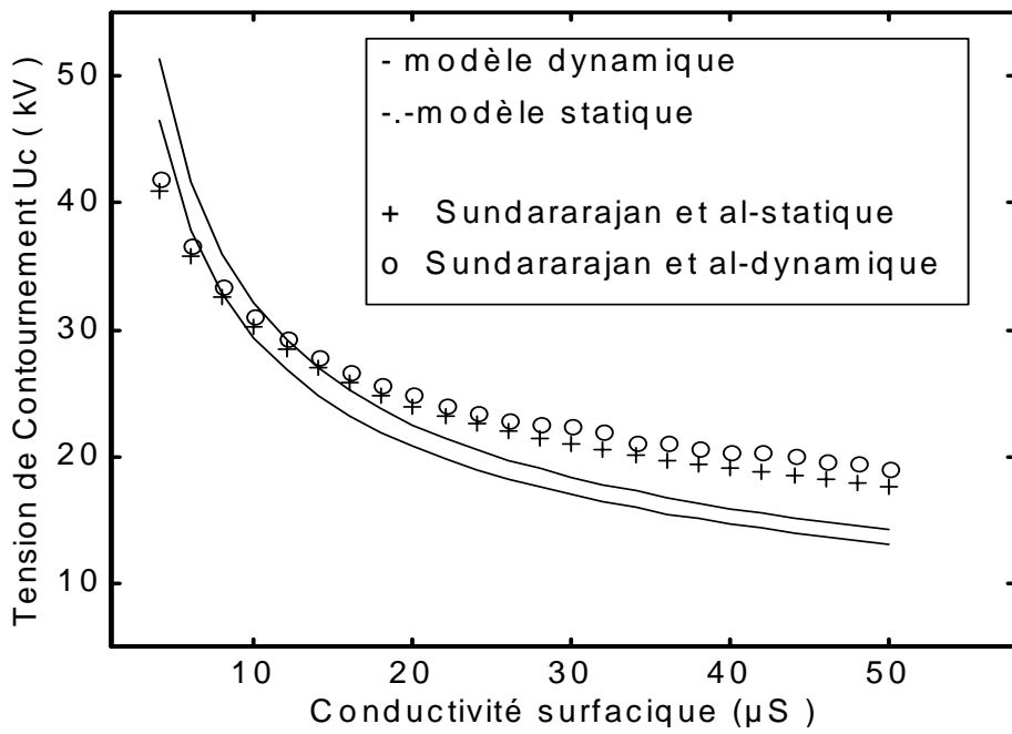
Figure 4.2: Tension de contournement en fonction de la conductivité surfacique
