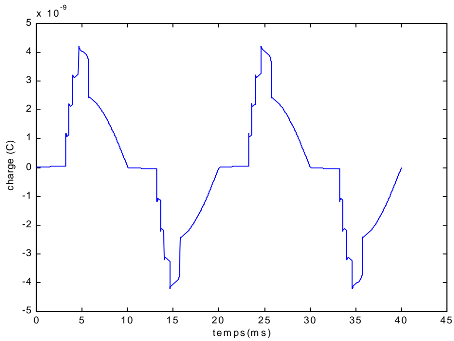
Figure 5.26: Charge en fonction du temps pour le cas d'un isolateur de longueur 50 cm, de rayon 5 cm et de conductivité 50 \mu\text{S} (réamorçage symétrique)
