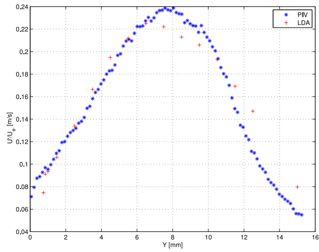
FIG. 2.25 – Profils d'intensité de turbulence de la vitesse longitudinale, comparaison PIV/LDA, x=302 mm.
