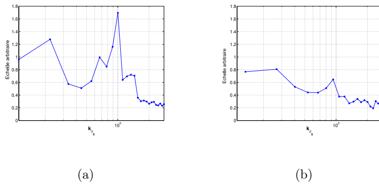
FIG. 3.21 – Spectre de Fourier associé avec Fig. 3.20. (a) : avec rugosité, (b) : sans rugosité.
