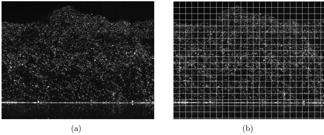
FIG. 2.4 – Exemple d’images PIV de traceurs dans notre écoulement (a), et découpages en cellule pour la corrélation (b)
