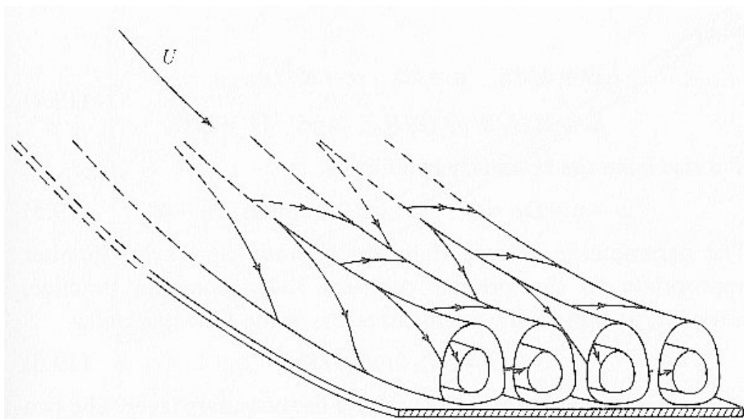
FIG. 3.22 – Organisation longitudinale des tourbillons de Görtler (tiré de Smits & Dussauge (1996) )
