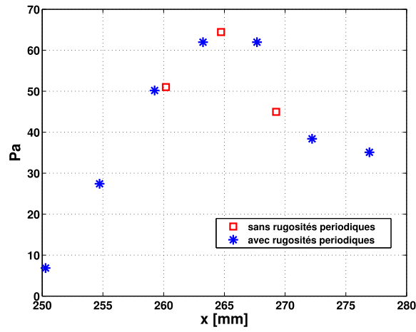
FIG. 3.24 – Pression RMS près du pied du choc réfléchi.
