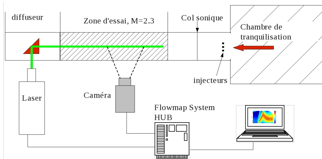
FIG. 2.13 – Schématisation du système PIV 2D
