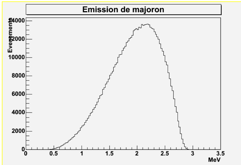
Fig. 7.3 : Spectre de l'énergie totale pour des évènements simulés de double désintégration bêta sans neutrino avec émission d'un Majoron.
