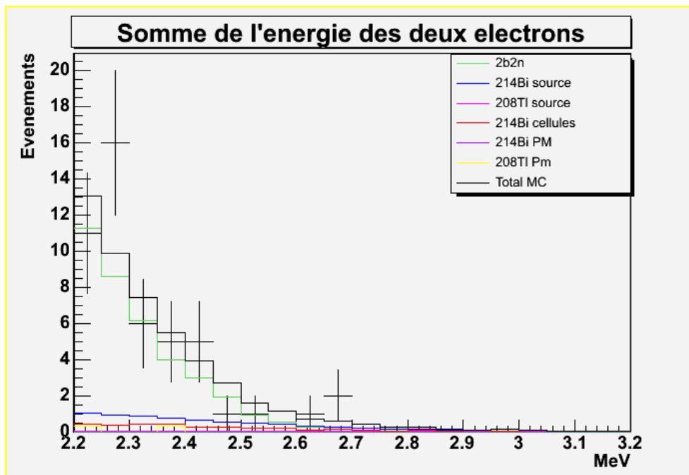
Fig. 7.7 : Spectre de la somme en énergie des deux électrons pour les évènements de type double bêta réels dans la fenêtre en énergie [2,2-3,2] MeV de la phase II, et contribution estimée des bruits de fond. La contribution totale des bruits de fond est indiquée par la ligne noire. Le signal est recherché sur l'intervalle [2,4-2,9] MeV.
