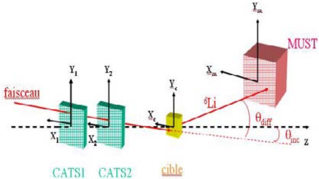
Figure 3.10 : Schéma explicatif du calcul de l'angle de diffusion.
