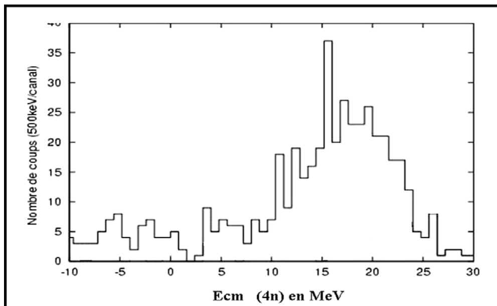
Figure 5.20: Spectre en énergie du système 4n issu de la réaction {}^8\text{He}(d, d\alpha) (détecteurs externes disposés entre 23 et 40°)
