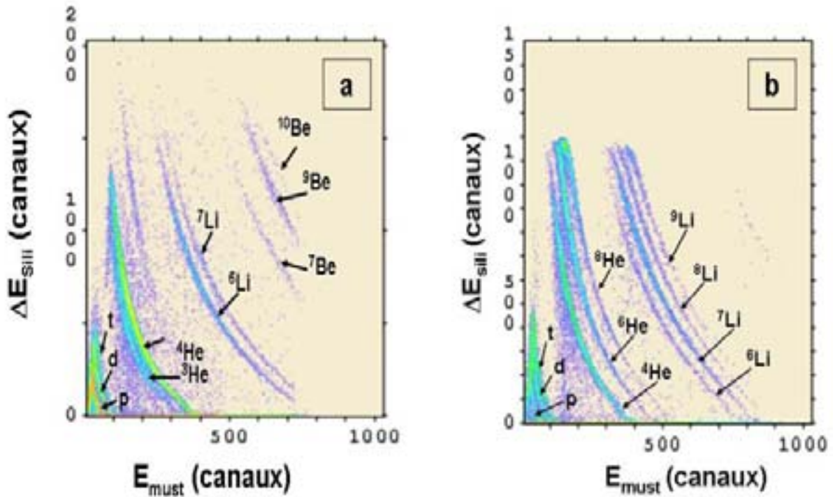
Figure 3.8.a et 3.8.b : Identification E_{\text{must}}-\Delta E_{\text{Sili}} , avec le faisceau de ^{12}\text{C}^{3+} en (a) et celui de ^8\text{He}^{2+} en (b).
