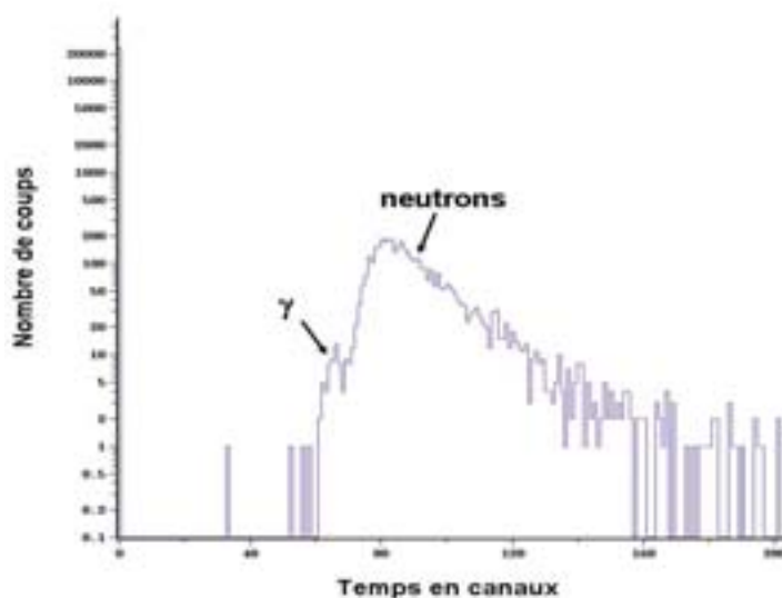
Figure 3.2 : Graphe des temps des détecteurs plastiques calibrés sommés ( T_{bntot} ).
