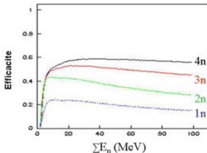
Figure 2.13: Efficacité intrinsèque de détection de 1,2,3 ou 4 neutrons.
