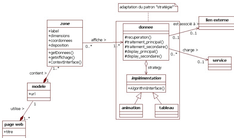
Figure 110 : modèle associé à la dimension « présentation »
