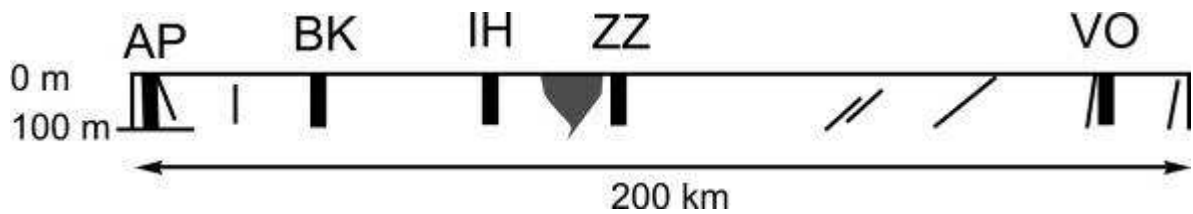
Figure 7.11 : Coupe verticale par interprétation des données gravimétriques par rehaussement vers le haut. AP : ZC d'Ampanihy ; BK : ZC de Beraketa ; IH : ZC d'Ihoisy ; ZZ : ZC de zafafotsy ; VO : ZC de Vondrozo. On met en évidence deux types de structures des zones à fort pendages et qui correspondent au ZC majeures, d'autres domaines avec de plus faible pendage (prendre en compte l'échelle des hauteurs). L'anomalie centrée sur Ihoisy pourrait correspondre à un corps magmatique.
