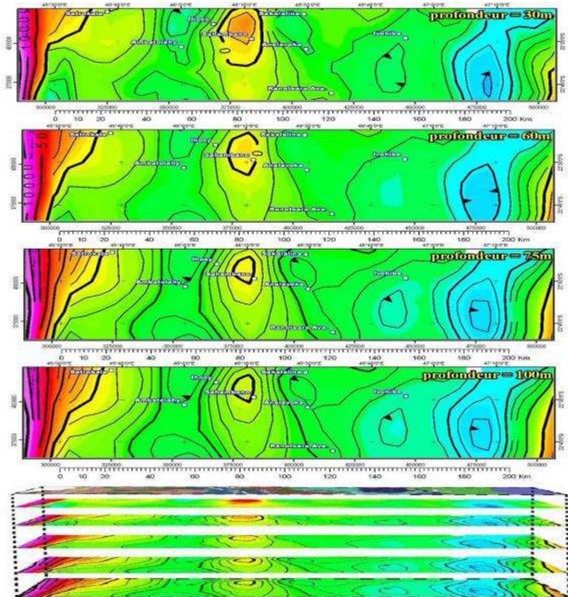
Figures 7.10 : (a) en haut, cartes de profondeur gravimétrique pour un rehaussement successif vers le haut de 30 m, 60m, 75m et 100m (région Ihoisy). Les triangles noirs indiquent la direction de décroissance de valeur (valeur en 10^{-2} mGal). (b) en bas, bloc diagramme 3D : mêmes figures placées sur une verticale, l'échelle des hauteurs est de 100 m, la largeur est de 200 km.
