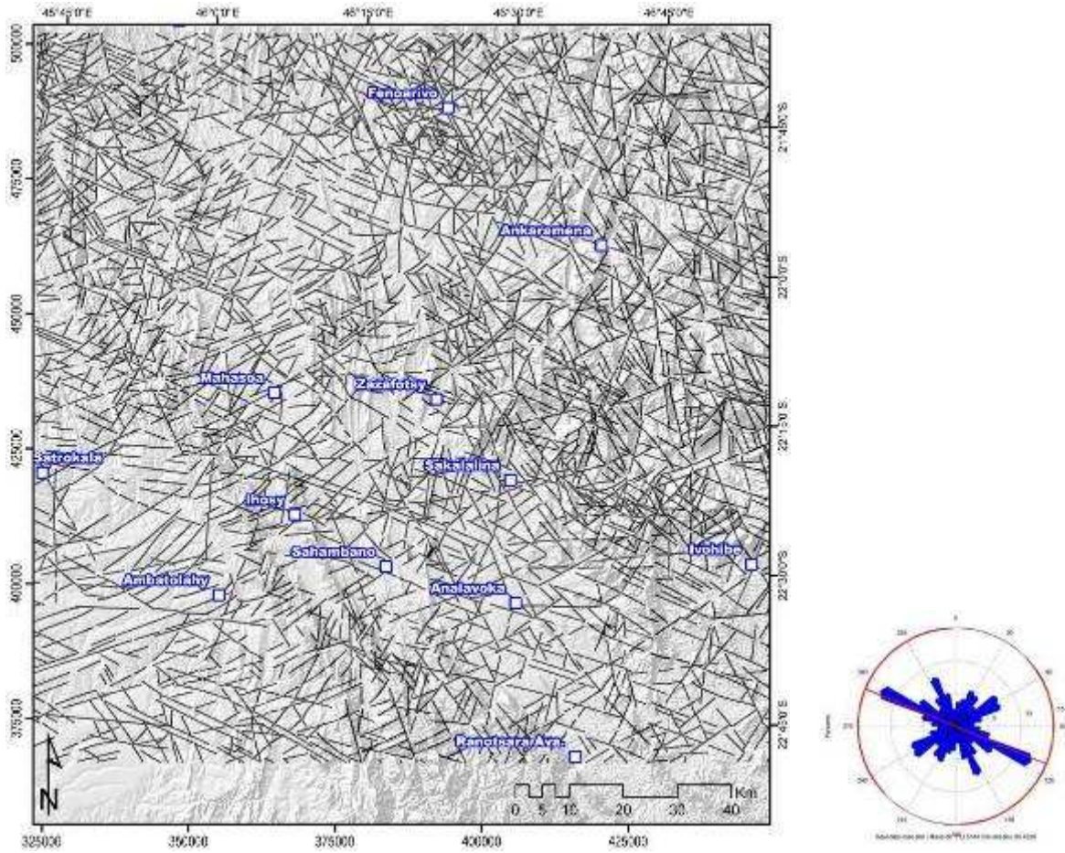
Figure 2.4 : Ensemble des Fractures cartographiées dans la région d'Ithos ; et diagramme de rose correspondant (direction majeure N 115° et autres directions moins représentées N 30°, N 60°, N 160°).
