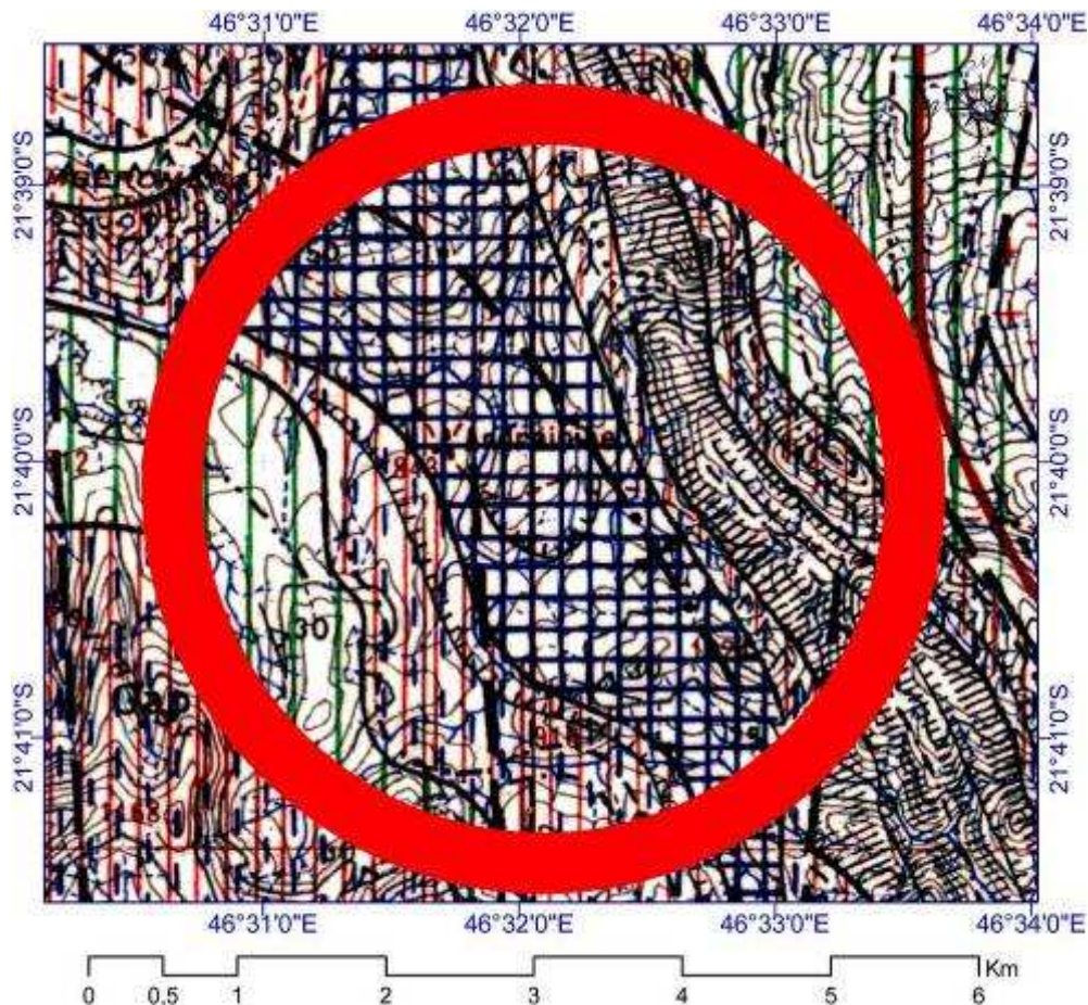
Figure 4.19 : Région de Fenoarivo (Nord – Ouest d’Ankaramena : relation « bull-eyes », ZC, et dykes (a) page précédente, sur une carte de champ magnétique résiduel H' , avec localisation d’une caldeira (cercle rouge) sur la carte géologique 1/100 000, feuille M54. Les « bull-eyes » sont associés principalement à de grands dykes kilométriques, ainsi qu’à leur intersection avec (i) d’autres dykes (cas BE1), (ii) des directions de foliations majeures (cas BE2), (iii) l’intersection avec la ZC de Zazafotsy (cas BE3), et (iv) un réseau d’anomalies ponctuelles négatives (cas BE4). Deux ZC (limites en lignes blanches) sont visibles sur cette image : la ZC de Morarano (à l’Ouest) et celle de Zazafotsy (à l’Est) ; (b) en haut, vue rapprochée du cercle rouge, caldeira dans la prolongation des dykes N 170°. Il est repéré (au centre du cercle rouge) sur la carte géologique 1/100 000, feuille Ankaramena -M54 (Bésairie, 1971) . Remarquez que la caldeira s’aligne comme les bull-eyes et les dykes, sur la direction des dykes N 170°- 160°. Je note que la caldeira ne figure pas sur la légende de la feuille Ankaramena.
