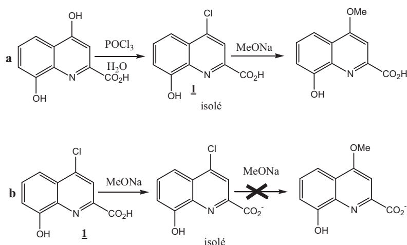
Figure 27 : Schéma de synthèse de la Quinolobactine par POCl 3 selon Neuenhaus et al.
