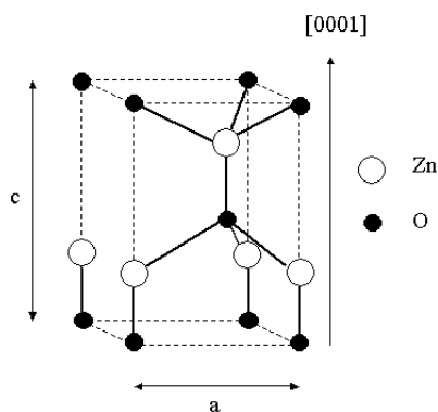
FIG. 1.2 – Maille primitive de la structure würtzite.
