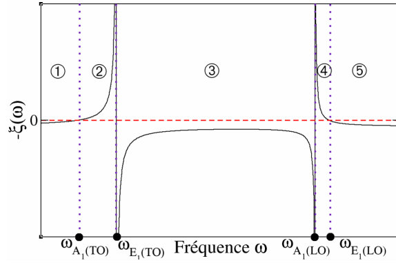
FIG. 3.1 – Graphe de la fonction -\xi = -\varepsilon_{\parallel}/\varepsilon_{\perp} . Les tirets rouges repèrent l'origine des ordonnées, les pointillés violets délimitent les domaines où -\xi(\omega) garde un signe constant.
