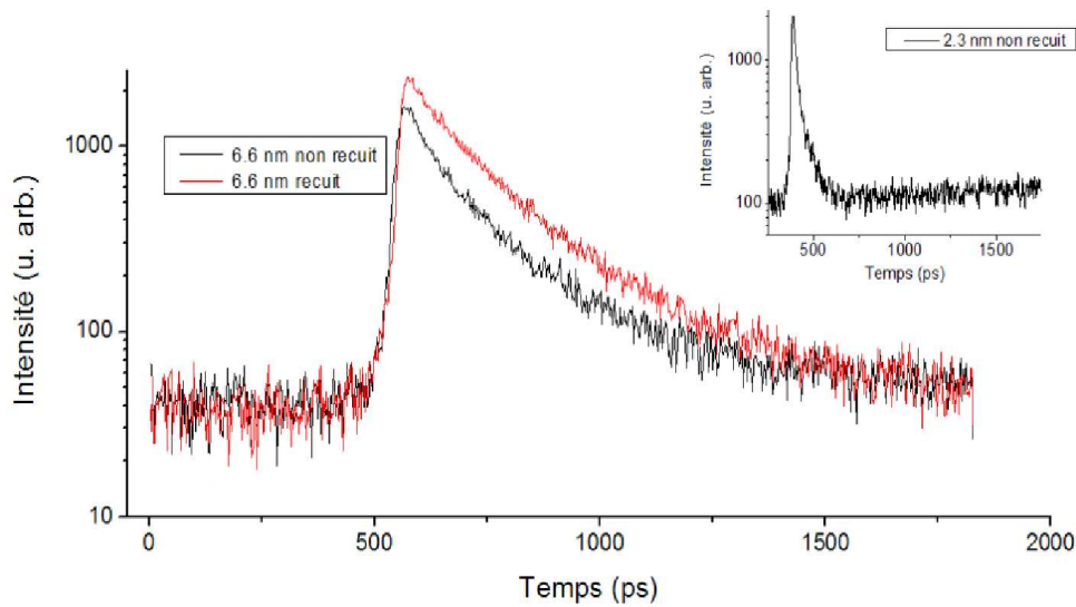
FIG. 4.7 – Traces temporelles de la nanoparticule de 6.6 nm avant (noir) et après (rouge) recuit. Insert : trace temporelle de la nanoparticule de 2.3 nm avant recuit.
