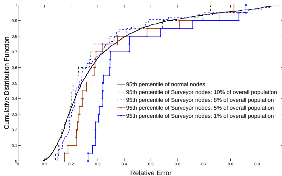
Figure 7.8 : Impact de la proportion de nœuds d'expert sur leur représentativité
