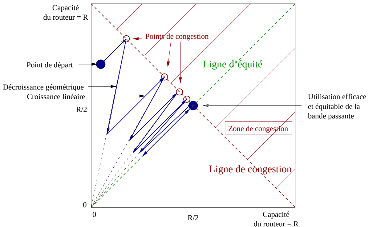
Figure 6.1 : Deux sources AIMD partageant une même ressource critique
