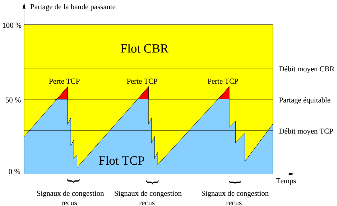
Figure 6.5 : L'effet rafale
