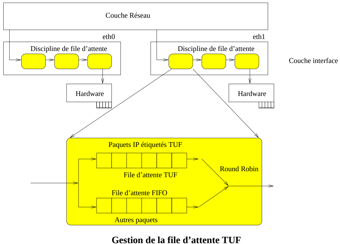
Figure 6.23 : Insertion de TUF dans le noyau linux
