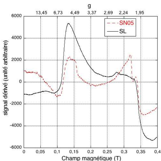
Figure IV-17 Spectres de RPE des verres SN05 et SL. P_{\text{micro-ondes}} : 63mW ; A_{\text{modu}} : 5G ; t_{\text{acq}} : 82ms ; t_{\text{filtr}} : 164ms ; gain : 3 \cdot 10^5
