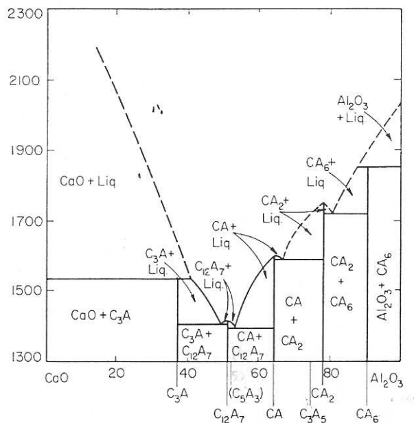
Figure II-3 Diagramme binaire du système \text{Al}_2\text{O}_3 - \text{CaO} (Levin et al. 1964). La composition est indiquée en pourcentage massique de \text{Al}_2\text{O}_3 .
