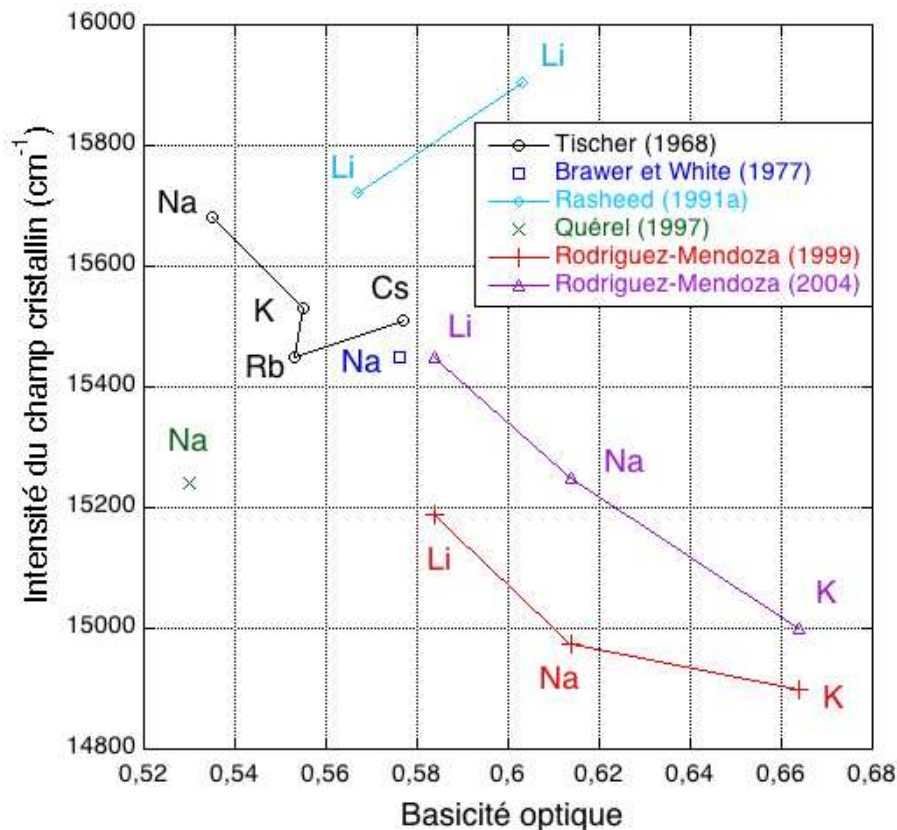
Figure I-13 Valeurs du champ cristallin \Delta_0 en fonction de la basicité optique (calculée selon Duffy) dans des verres de silicate d'alcalin. D'après Tischer (1968), Brawer et White (1977), Rasheed et al. (1991a), Quérel (1997), Rodriguez-Mendoza et al. (1999 et 2004).
