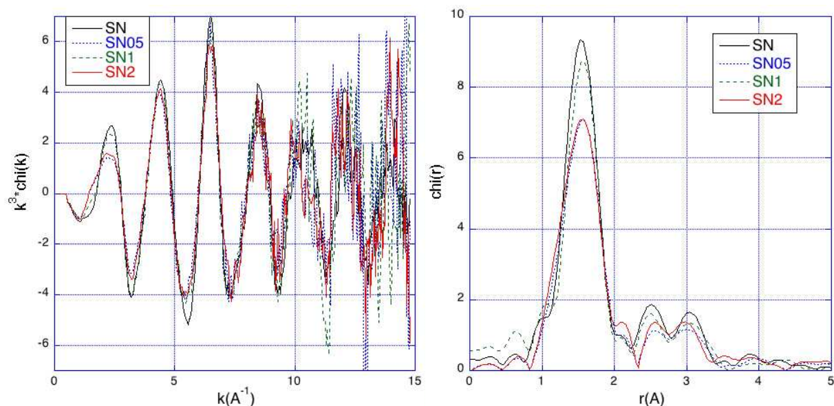
Figure IV-10 Comparaison du signal EXAFS (à gauche) des verres silicatés sodiques à concentration croissante en Cr (0,04, 0,5, 1 et 2% de Cr 2 O 3 ). Comparaison de la TF entre 2,7 et 10,5 Å -1 (à droite).
