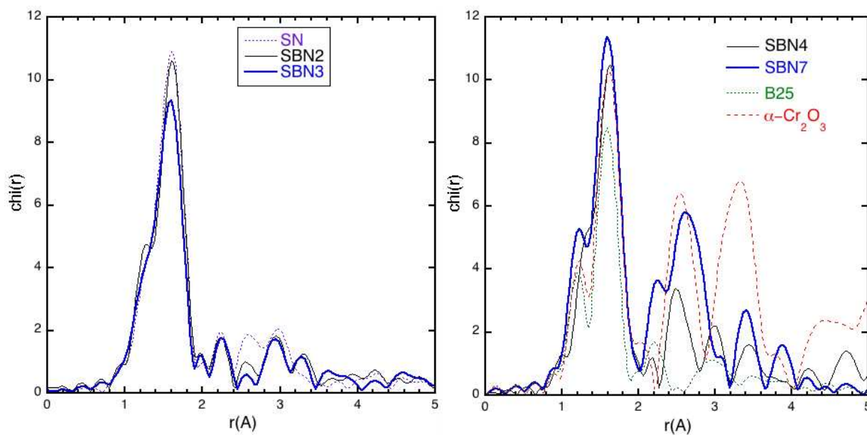
Figure V-17 TF des spectres EXAFS de la Figure I-11. A gauche , verres SBN2 et SBN3 (entre 2,7 et 14,2 \text{\AA}^{-1} ). Comparaison avec le verre SN (entre 2,7 et 14,3 \text{\AA}^{-1} ). A droite , verres SBN4 et SBN7 (de 2,7 à 14,5 et 14,2 \text{\AA}^{-1} ). Comparaison avec le verre B25 et \alpha\text{-Cr}_2\text{O}_3 (entre 2,7 et 14,3 \text{\AA}^{-1} ).
