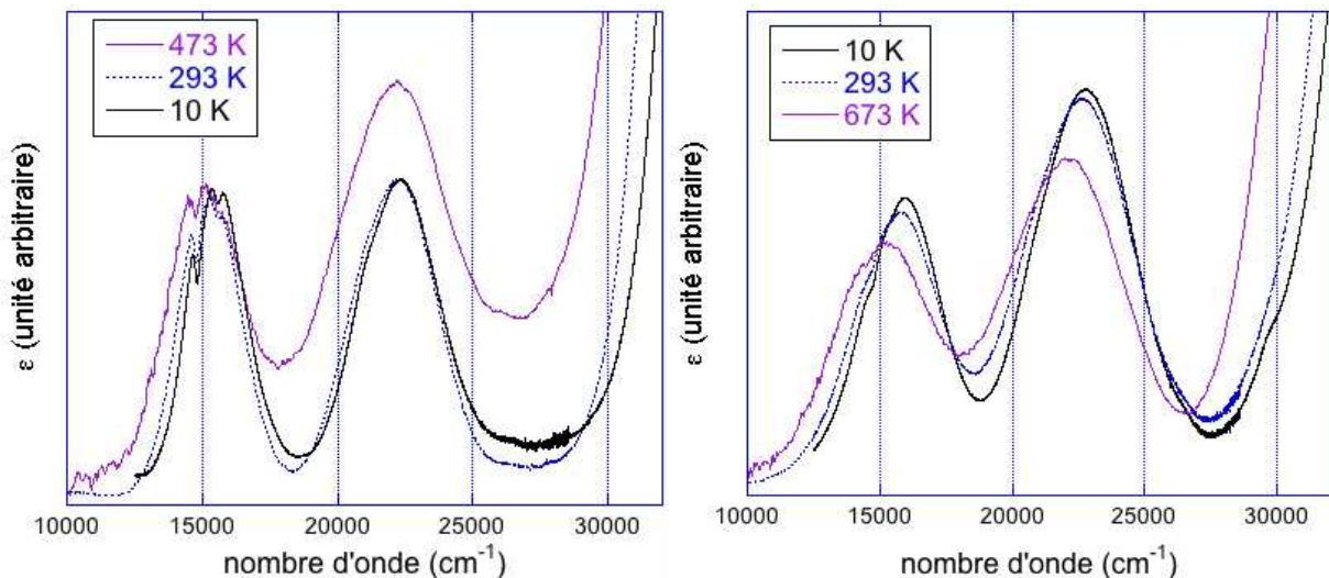
Figure VI-4 Spectres d'absorption optique de 10 à 473 K du verre SN (à gauche). Spectres d'absorption optique de 10 à 673 K du verre SBN3 (à droite).
