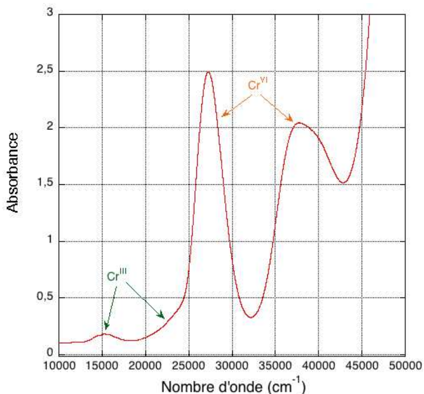
Figure 6-2 Spectre d'absorption optique d'un verre silicaté sodique ( 75\text{SiO}_2\text{-}25\text{Na}_2\text{O} ) à très forte proportion relative de \text{Cr}^{\text{VI}} .
