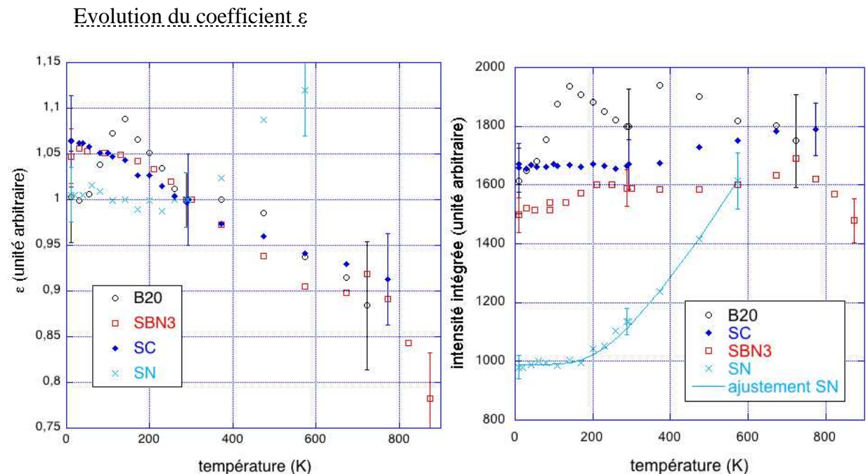
Figure VI-11. (à gauche) Intensité (coefficient d'extinction molaire \varepsilon ) de la bande de champ cristallin en fonction de la température. (à droite) Intensité intégrée (produit de la largeur par \varepsilon ). L'évaluation de l'incertitude a été indiquée à température ambiante et aux températures extrêmes.
