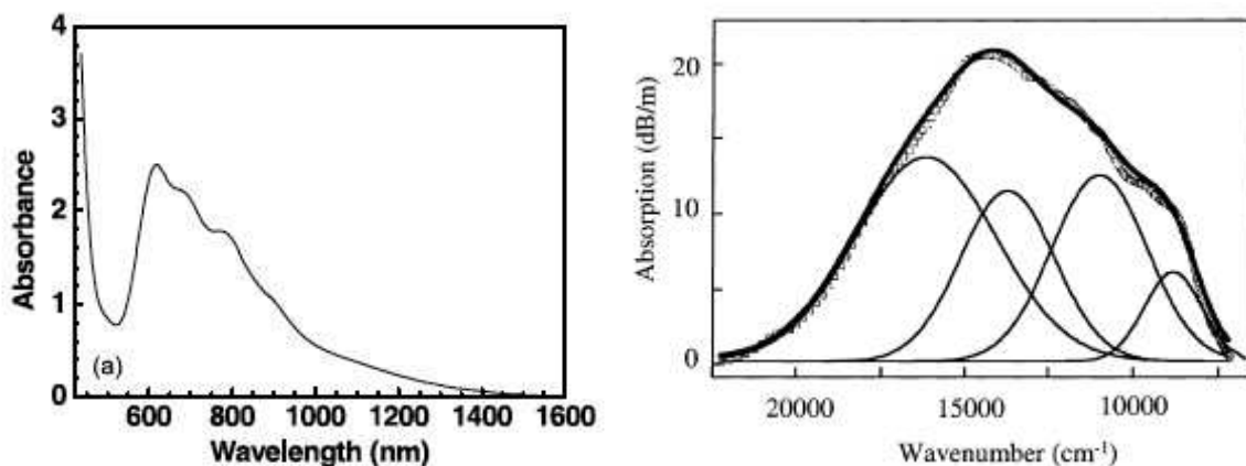
Figure I-8 (à gauche) Spectre d'absorption optique du \text{Cr}^{\text{IV}} (et \text{Cr}^{\text{VI}} ) dans un verre 66\text{CaO}-29\text{Al}_2\text{O}_3-5\text{SiO}_2-0,1\text{Cr}_2\text{O}_3 . D'après Feng et Tanabe (2002). (à droite) Spectre d'absorption corrigé du fond de la fibre dopée au Cr et codopée Al (cercles) ; ajustement (trait plein épais) et sa décomposition en quatre gaussiennes correspondant au \text{Cr}^{4+} (trait plein fin). D'après Felice et al. (2001)
