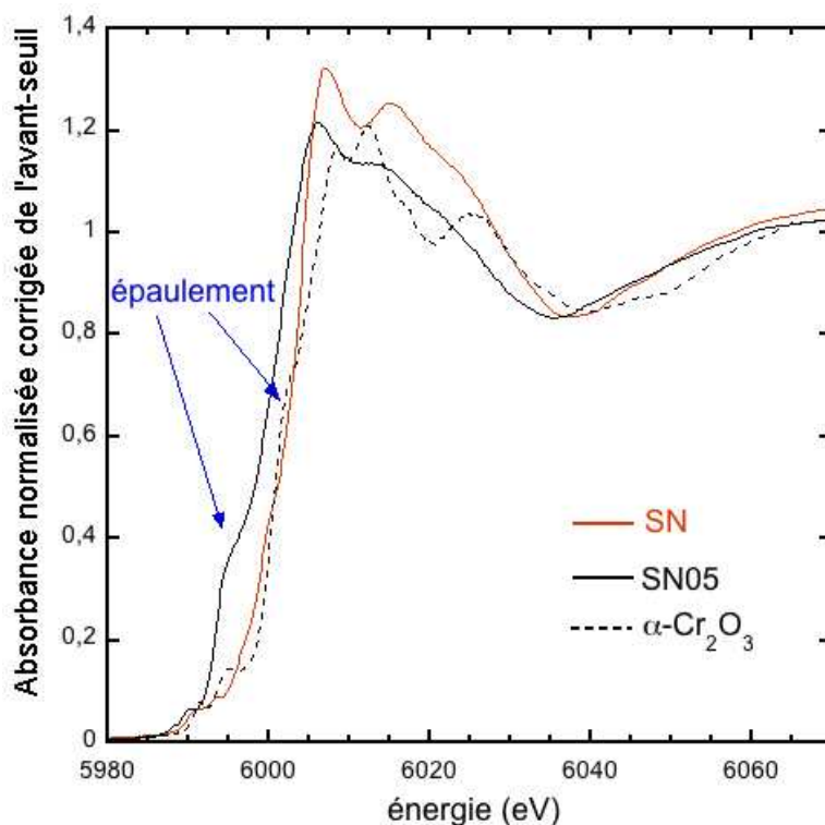
Figure IV-9 Evolution des spectres XANES (normalisés) avec la concentration en Cr dans un verre de trisilicate de sodium (SN et SN05). Référence cristallisée ( \alpha -Cr 2 O 3 ).
