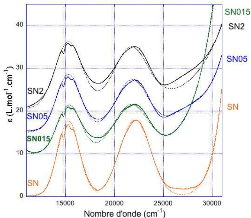
Figure IV-8 Spectres d'absorption optique des verres silicatés à 26 % de Na 2 O. Le pourcentage nominal de Cr 2 O 3 est de 2 %, 0,5 %, 0,15 % et 0,04 % (de haut en bas). Les spectres sont représentés en coefficient d'extinction molaire et décalés en ordonnée. Les spectres expérimentaux sont en trait plein, leurs ajustements sont en pointillé.
