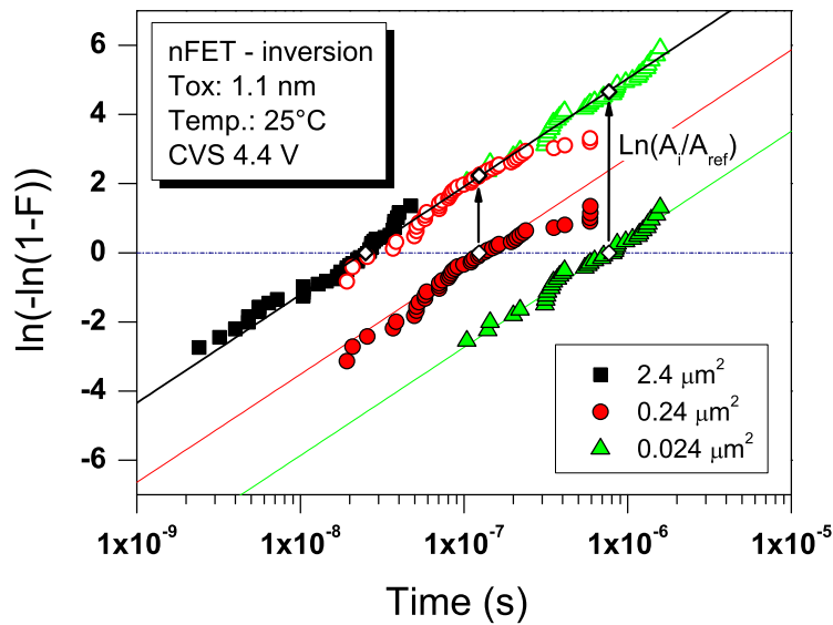
Figure 4: Les distributions de temps au claquage de dispositifs nFET de 1.1 nm d'épaisseur d'oxyde de grille différentes surfaces d'oxyde de grille sont tracées pour des stress à tension constante (CVS) à 4.4 V et 25 °C.
