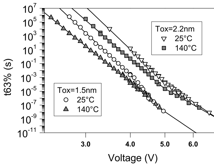
Figure 8: Accélération en tension des dispositifs de type nFET d'épaisseur d'oxyde de grille T_{\text{ox}} = 1.5 nm et 2.2 nm à 25 °C et à 140 °C [22].
