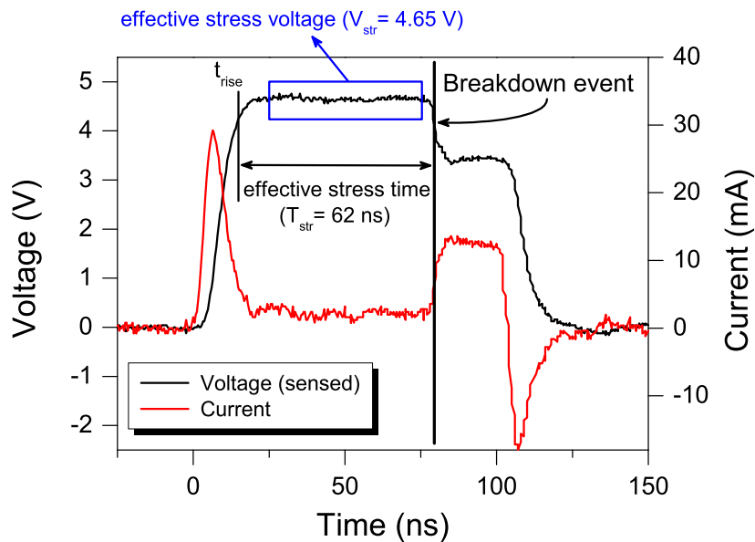
Figure 2: Forme d'onde mesurée à la grille pour un stress à 4.65 V. La détection de l'événement du claquage durant le pulse est présentée pour la détermination du temps effectif de claquage ( T_{BD,eff} = 62 ns). Les pics de courant observés au début et à la fin du pulse sont induits par la réflexion de la ligne de transmission.
