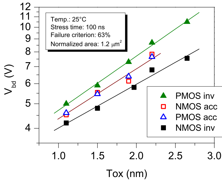
Figure 7: Accélération en tension du claquage en fonction de l'épaisseur physique de l'oxyde pour des dispositifs nFET et pFET stressés à 25 °C dans le régime HBM (~ 100 ns pulse) pour une surface de grille normalisée à 1.2 \mu\text{m}^2 [20].
