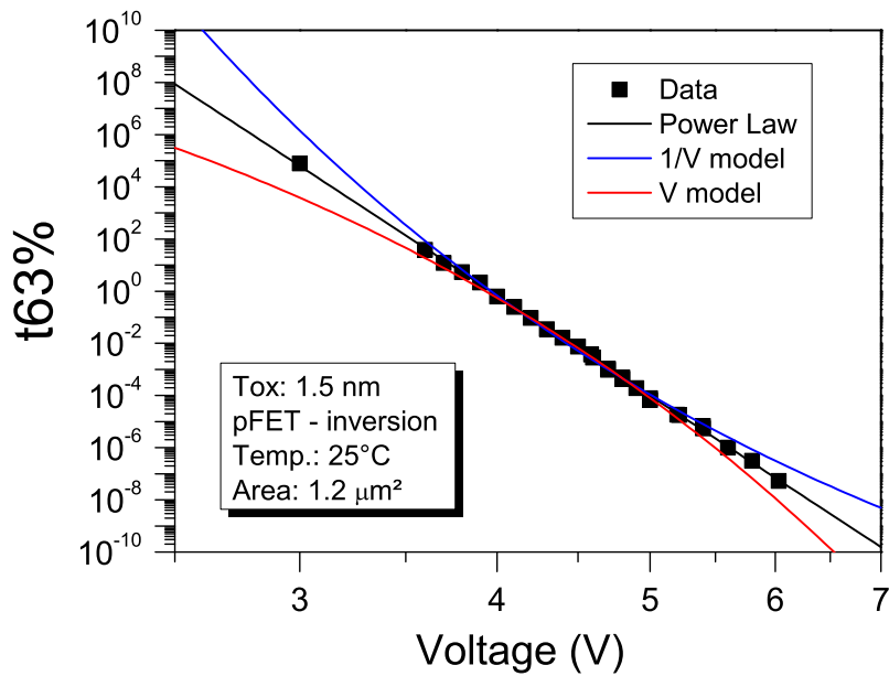
Figure 6: TDDb des dispositifs de type pFET pour une épaisseur d'oxyde de 1.5 nm stressé en inversion à 25 °C [21].
