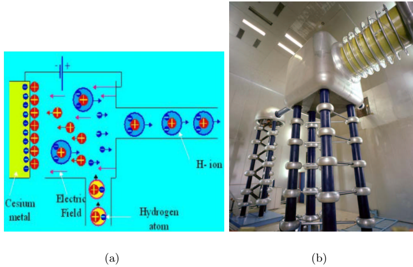
FIG. 2.1 – Principe de production des ions H^- (a) dans l'accélérateur Cockcroft-Walton (b).
