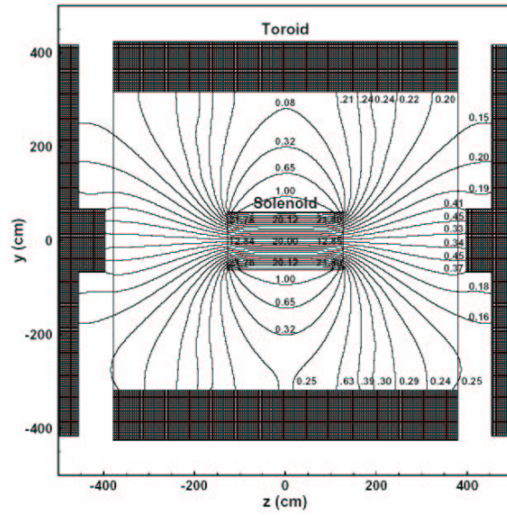
FIG. 2.12 – Carte du champ magnétique du solénoïde de D\bar{O} . Les valeurs du champ magnétique sont indiquées en kG ( 1 \text{ kG} = 0,1 \text{ T} ).
