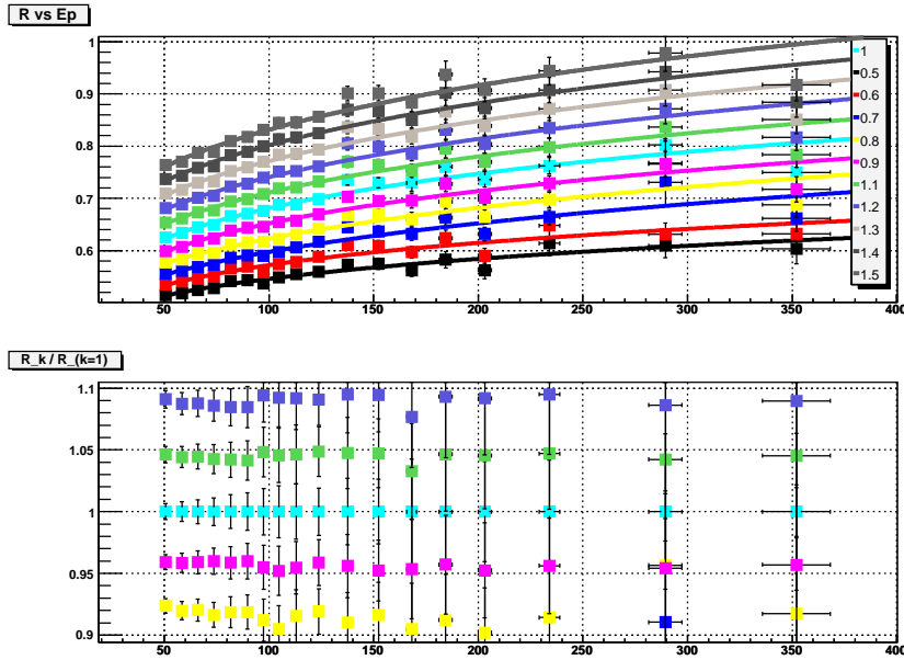
FIG. A.3 – La figure du haut présente le coefficient de réponse du calorimètre hadronique pour des jets dans l’ICR ( 0,8 < |\eta_{\text{jet}}^{\text{det}}| < 2 ) en fonction de E' , déterminée par la méthode “MPF” dans des données \gamma +jet. Les différentes couleurs correspondent à différentes valeurs multiplicatives appliquées aux constantes de calibration en \eta du calorimètre, indiquées dans la légende de la figure. La figure du bas présente le rapport de ce coefficient de réponse par rapport au coefficient obtenu avec les constantes actuelles de calibration, en fonction de E' .
