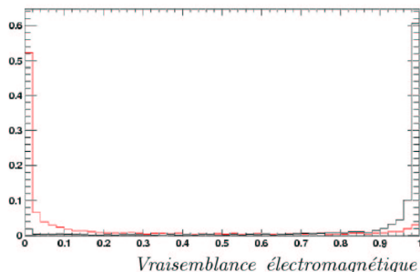
FIG. 3.7 – Vraisemblance électromagnétique pour des électrons dans le calorimètre central dans des données Z \rightarrow e^+e^- + \text{jets} (en noir) et pour des jets dans des données dijets (en rouge) [66].
