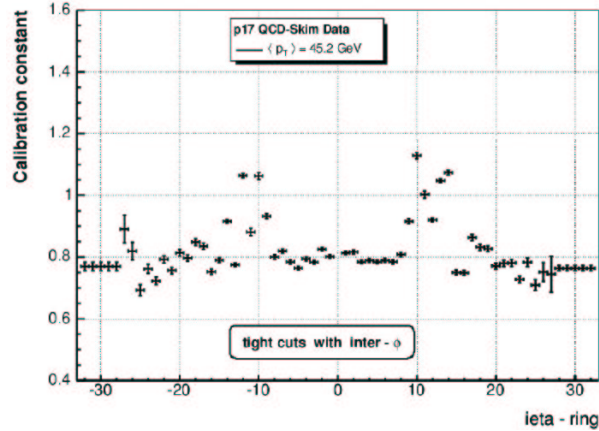
FIG. 3.13 – Constantes de calibration du calorimètre hadronique en fonction de i\eta \approx 10 \times \eta (Run IIa).
