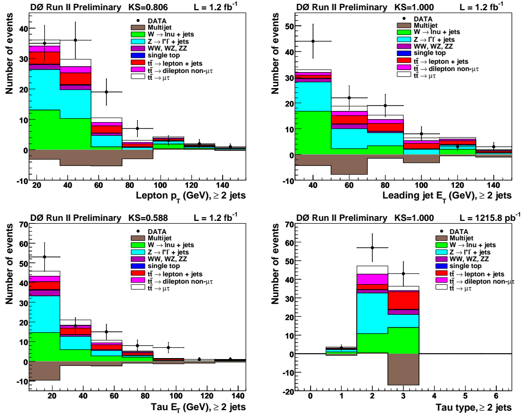
FIG. 7.15 – Distributions de l'impulsion transverse du muon (de l'électron), du jet de plus grand p_T et du tau, ainsi que le type du tau, pour les événements Lepton+Jets+Tau du canal \mu + \tau . Les données sont représentées par des points; les couleurs représentant les différents bruits de fond sont données dans la légende des figures.
