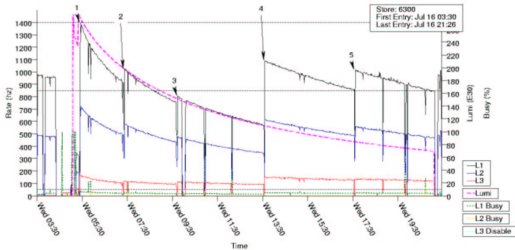
FIG. 2.4 – Taux de déclenchement en fonction du temps des différents niveaux du système d’acquisition des données (noir : niveau 1, bleu : niveau 2 et rouge : niveau 3) durant un “store”. La courbe rose représente l’évolution de la luminosité instantanée. Les chiffres noirs indiquent le début de chaque “run”.
