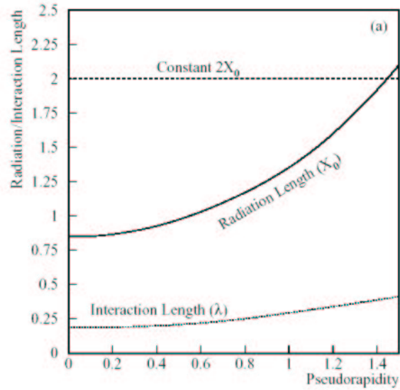
FIG. 2.13 – Longueur de radiation équivalente de l'aimant solénoïdal en fonction de la pseudorapidité.
