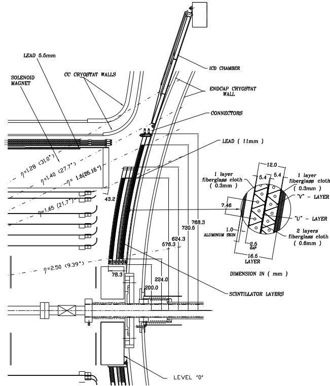
FIG. 2.22 – Coupe longitudinale de la partie supérieure d'un des FPS.
