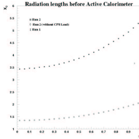
FIG. 2.16 – Nombre de longueurs de radiation X_0 avant la première couche active du calorimètre pour le Run I et le Run II, en fonction de la pseudorapidity \eta .
