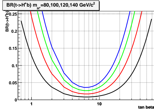
FIG. 1.11 – Rapport d’embranchement du top en un boson de Higgs chargé et un quark b , en fonction de \tan\beta . La courbe bleue correspond à un boson de Higgs chargé d’une masse de 80 \text{ GeV}/c^2 , la courbe verte de 100 \text{ GeV}/c^2 , la courbe rouge de 120 \text{ GeV}/c^2 et la courbe noire d’une masse de 140 \text{ GeV}/c^2 .
