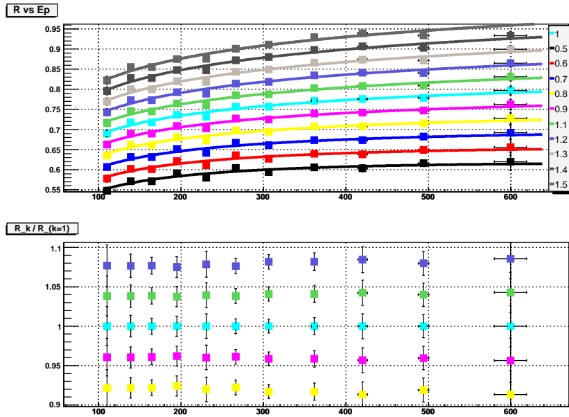
FIG. A.2 – La figure du haut présente le coefficient de réponse du calorimètre hadronique pour des jets dans l’EC ( 1,6 < |\eta_{\text{jet}}^{\text{det}}| < 2,0 ) en fonction de E' , déterminée par la méthode “MPF” dans des événements Monte Carlo \gamma +jet. Les différentes couleurs correspondent à différentes valeurs multiplicatives appliquées aux constantes de calibration en \eta du calorimètre, indiquées dans la légende de la figure. La figure du bas présente le rapport de ce coefficient de réponse par rapport au coefficient de réponse obtenu avec les constantes actuelles de calibration, en fonction de l’énergie du jet.
