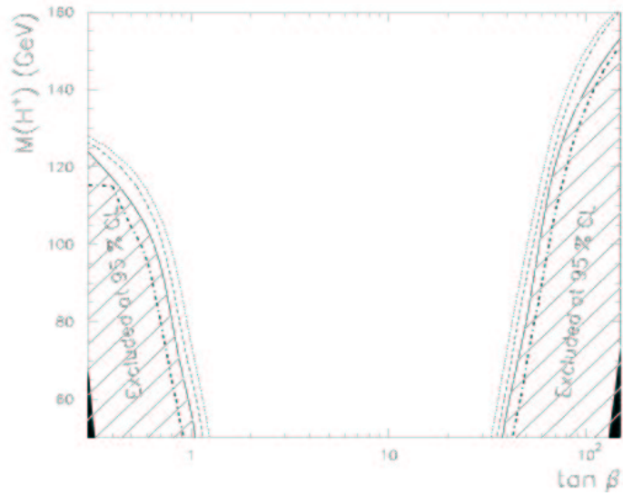
FIG. 1.22 – Zones d'exclusion, avec un niveau de confiance de 95%, du boson de Higgs chargé dans le plan (\tan \beta, m_{H^\pm}) obtenues par l'expérience D\bar{O} au Run I [27]. La masse du top est supposée à 175 \text{ GeV}/c^2 et la section efficace de production \sigma(t\bar{t}) est fixée à 5,5 pb (régions hachurées, lignes pleines), à 5 pb (lignes segmentées) et à 4,5 pb (lignes pointillées). Les lignes alternant points et tirets à l'intérieur des régions hachurées correspondent à une analyse fréquentiste avec \sigma(t\bar{t}) = 5,5 \text{ pb} .
