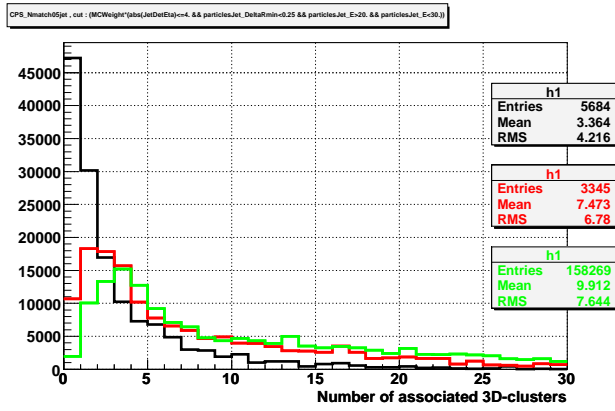
FIG. 6.2 – Distribution du nombre de clusters-3D associés par jet dans les événements Monte Carlo \gamma +jet. Seuls les événements avec un jet central ( |\eta_{\text{jet}}^{\text{det}}| < 0,4 ) sont considérés. L'énergie originelle des particules constituant le jet est requise entre 20 et 30 GeV pour la courbe noire, entre 50 et 60 GeV pour la courbe rouge et supérieure à 100 GeV pour la courbe verte.
